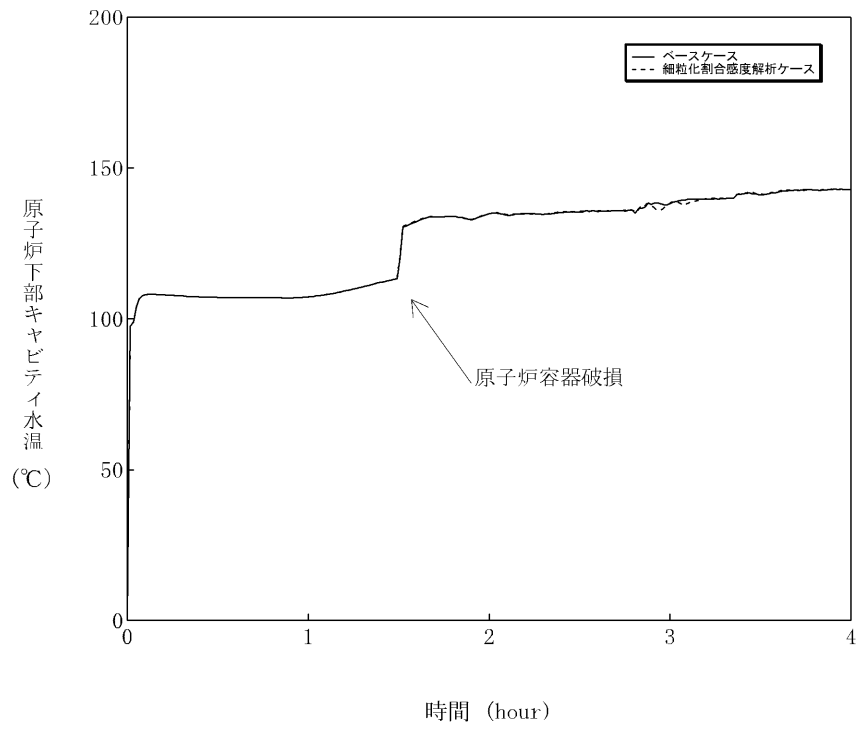
図 5・3・5 エントレインメント係数感度解析 (5)
