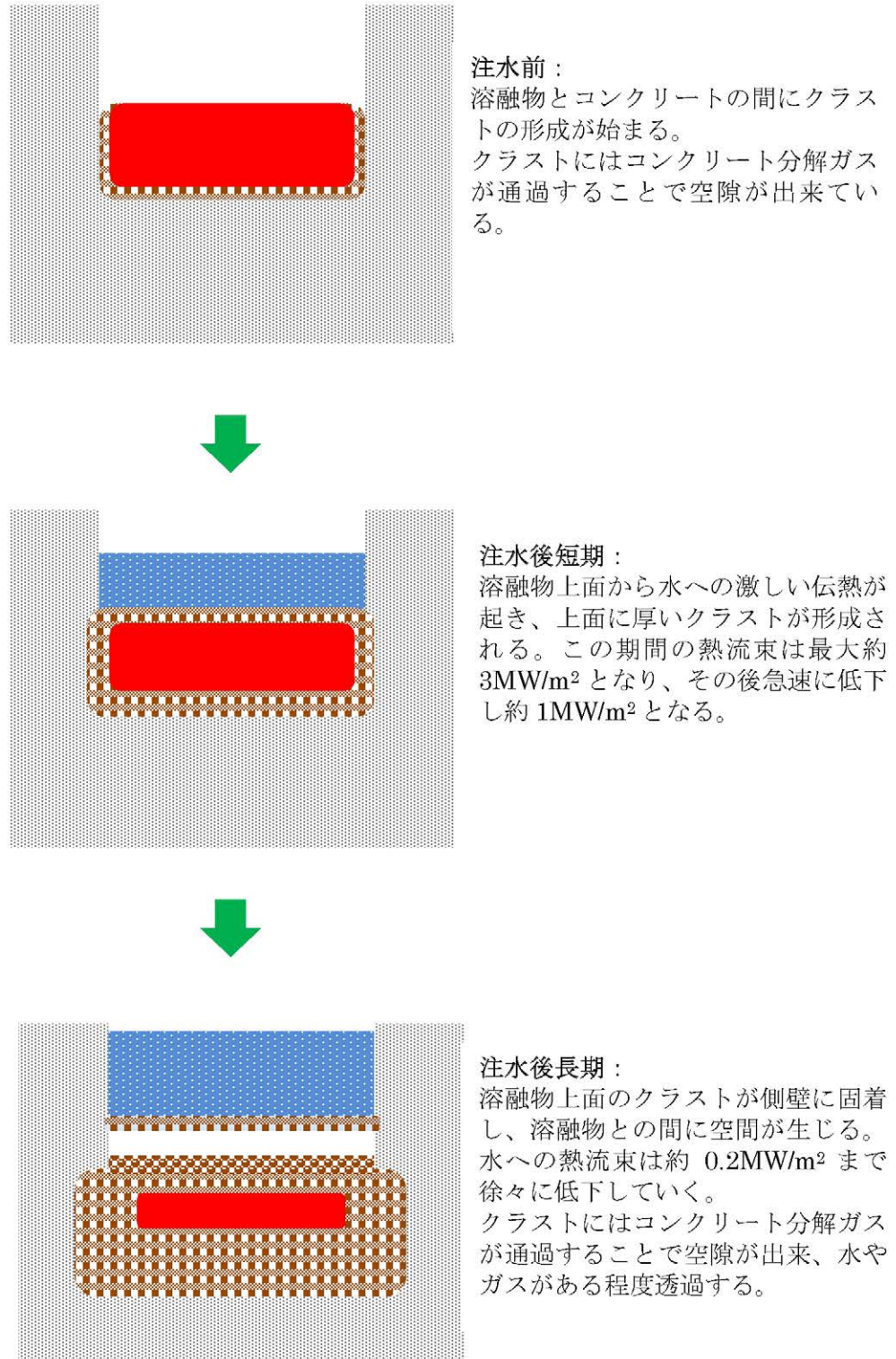
図 3.3-1 MCCI 実験での挙動
