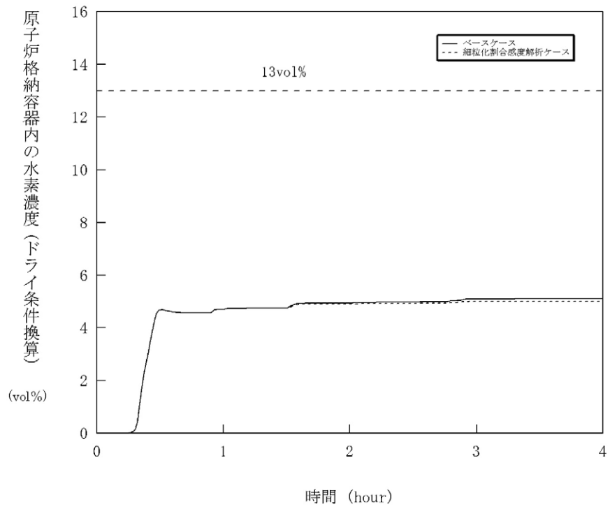
図 5-2-9 溶融炉心の細粒化割合感度解析 (9)
