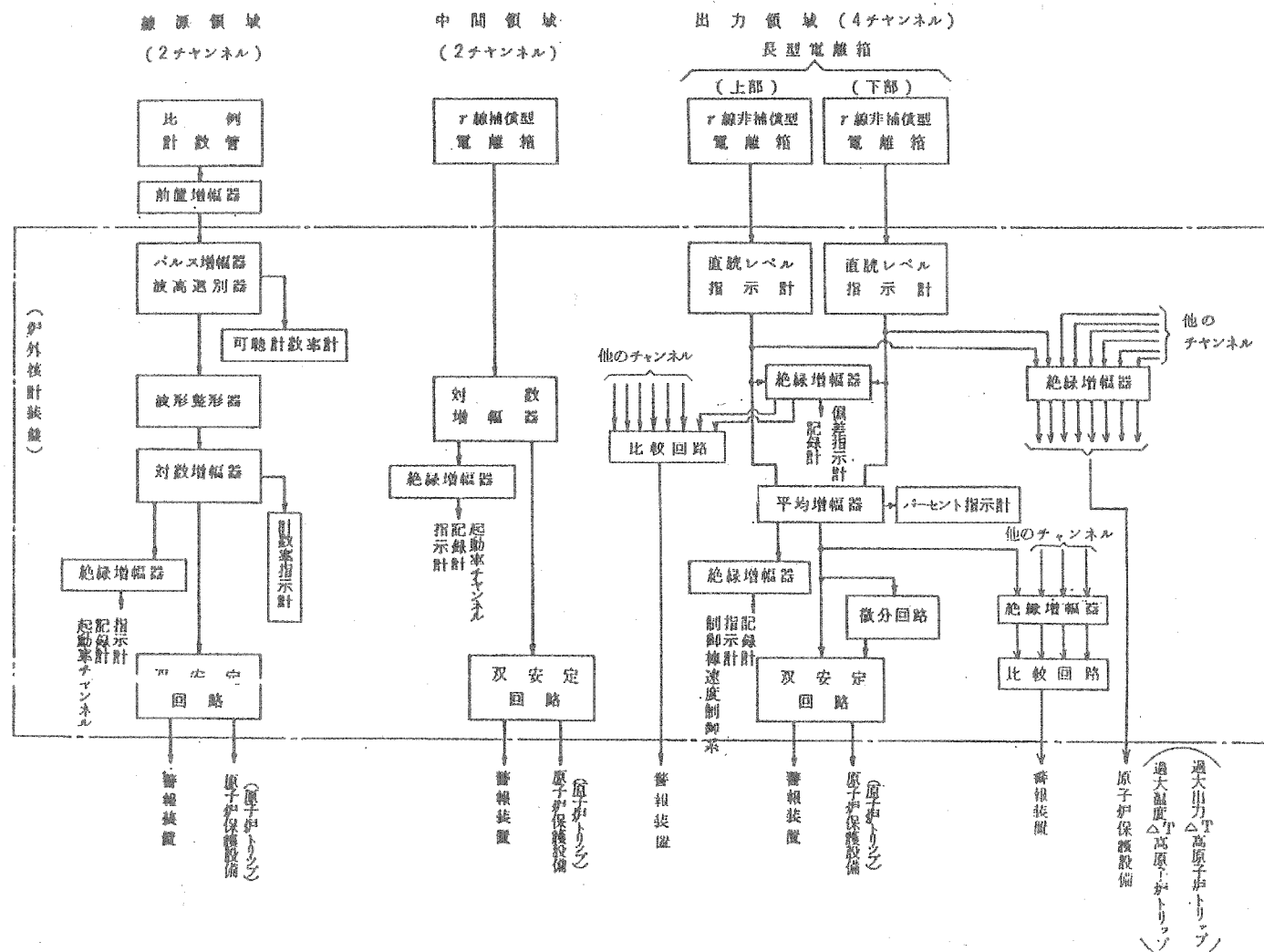
第1.7-18図 炉外核計装概略図
