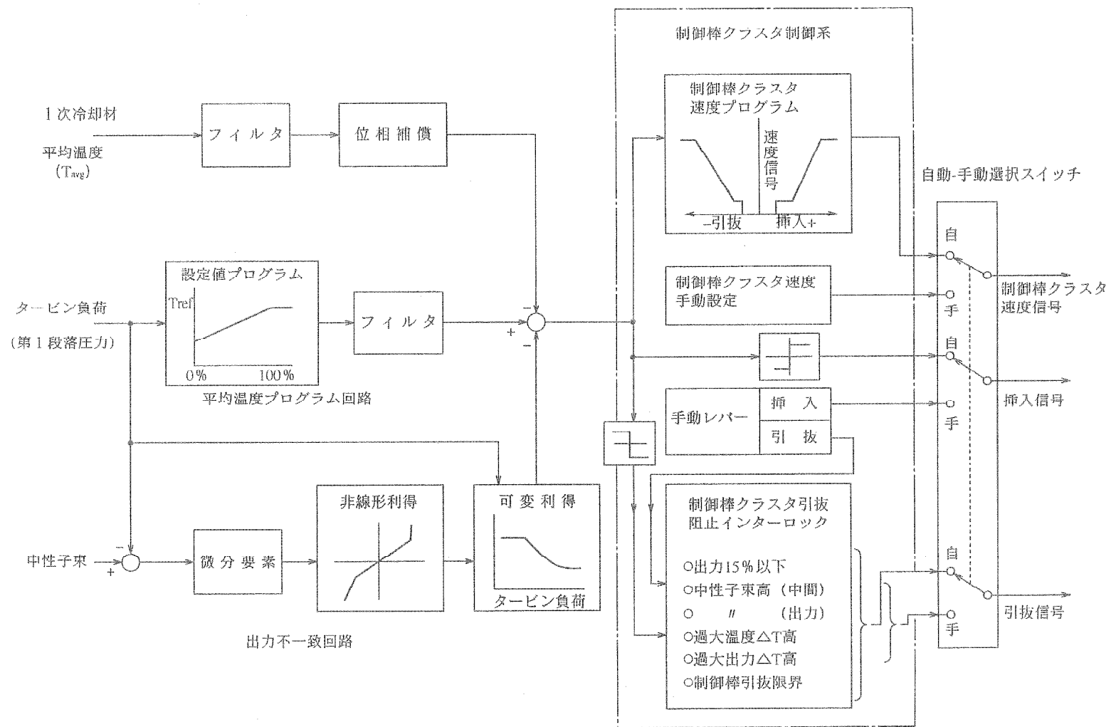
第1.7-3図 制御棒クラスタ制御系説明図
