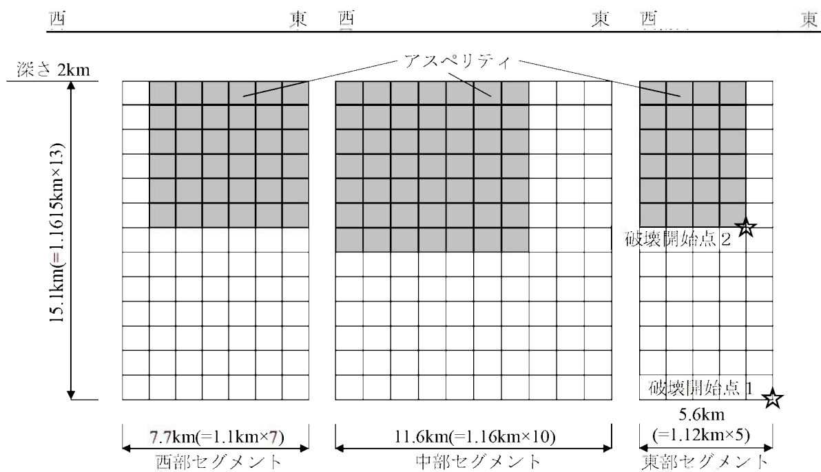
(b) 断面図
