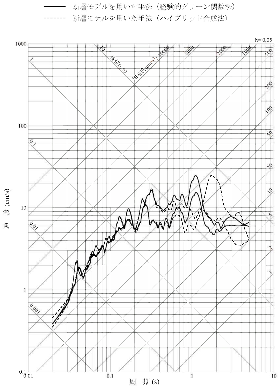
第1.2-289図 市来断層帯甕海峡中央区間による地震の不確かさを考慮した地震動の応答スペクトル （応力降下量の不確かさを考慮したケース:鉛直方向）
