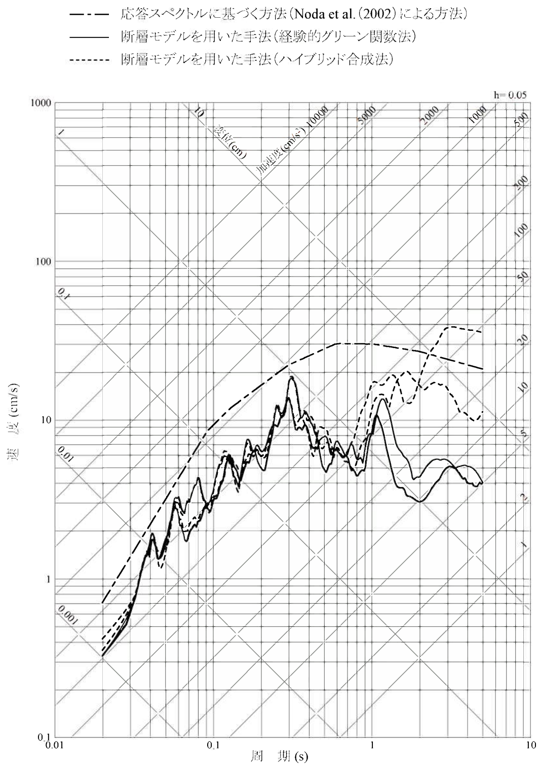
第1.2-283図 断層帯断層傾斜角の不確かさを考慮した地震動の応答スペクトル (断層傾斜角の不確かさを考慮したケース:鉛直方向)
