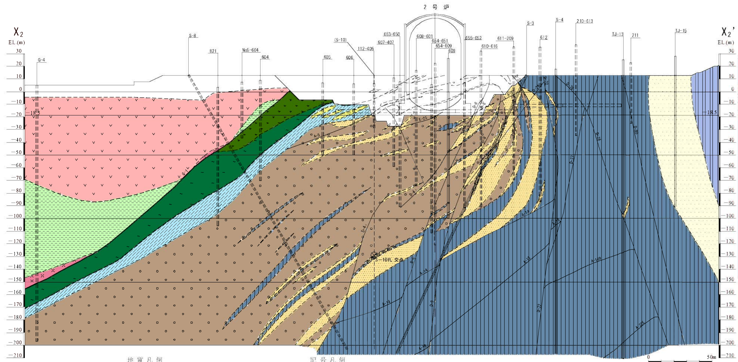
地質凡例
