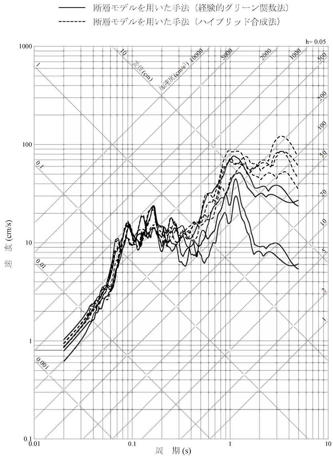
第1.2-288図 市来断層帯甕海峡中央区間による地震の不確かさを考慮した 地震動の応答スペクトル (応力降下量の不確かさを考慮したケース: 水平方向)
