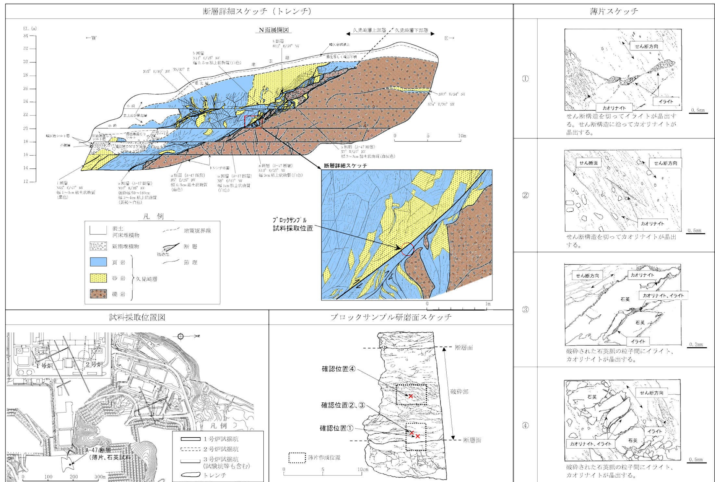
第1.2-209図 断層詳細スケッチ・薄片観察結果(A-47断層) 1.2-713
