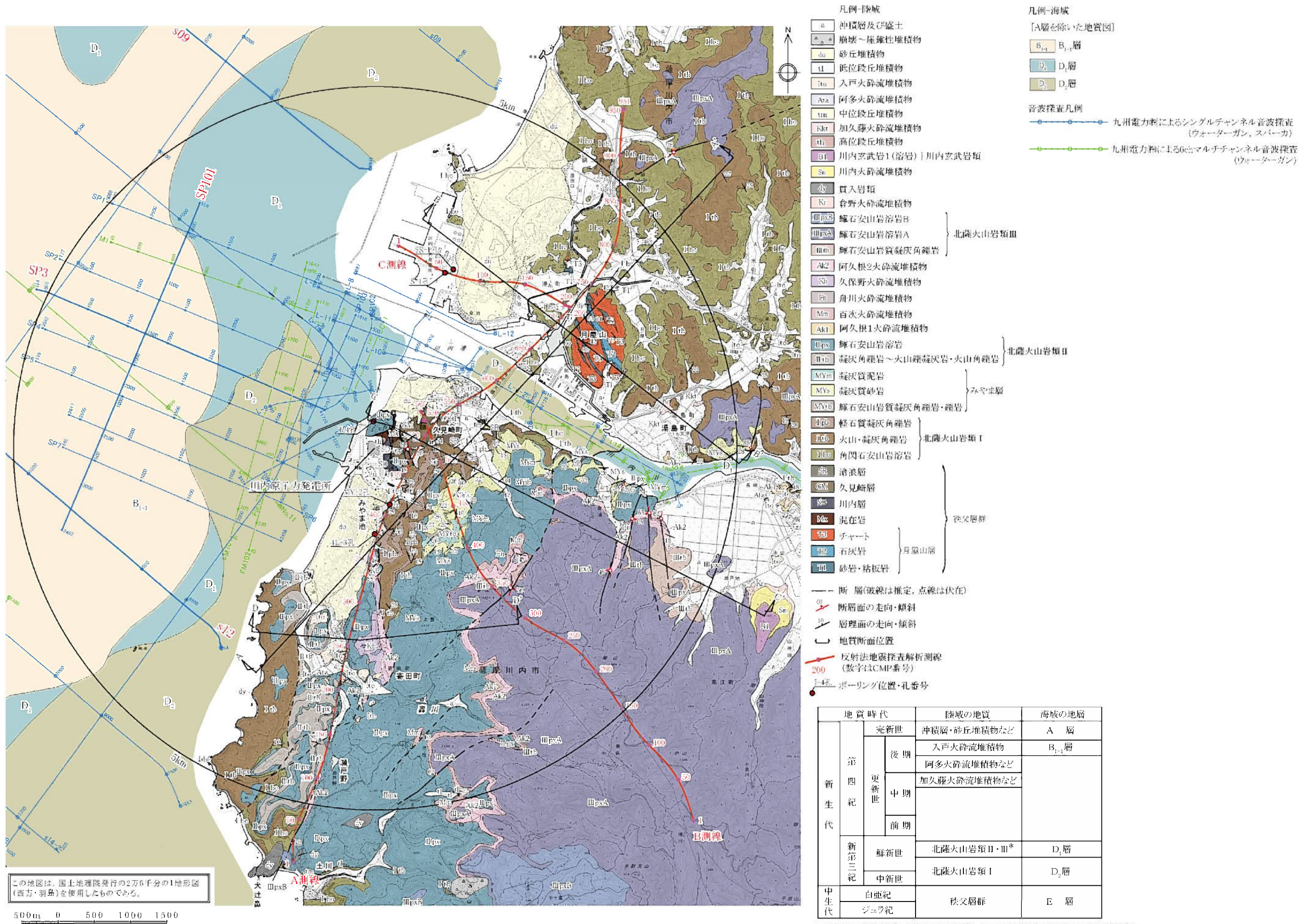
第1.2-182図 敷地近傍の地質図 1.2-681
