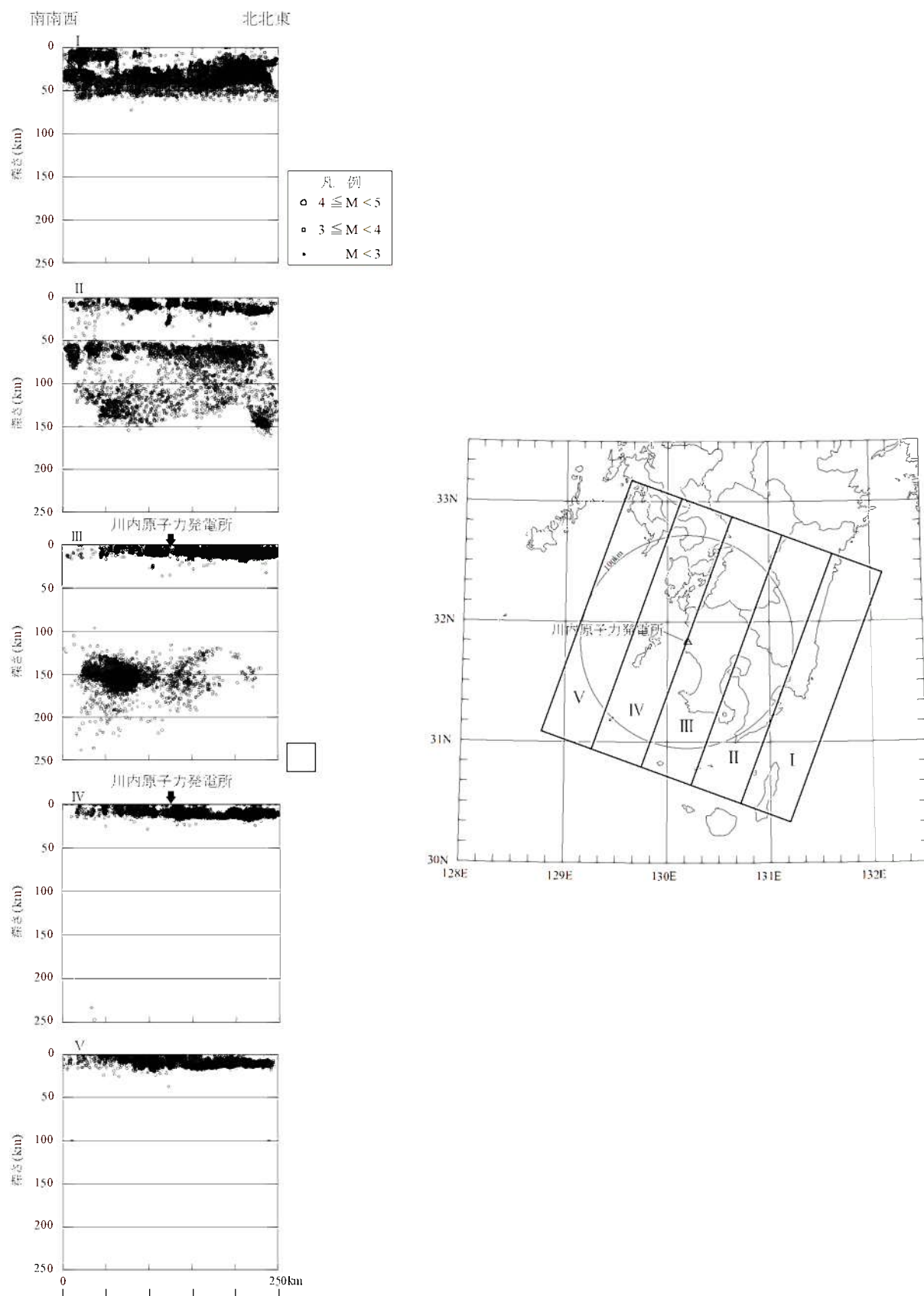
第1.2-243図(2) 気象庁地震カタログによる微小地震の震源鉛直分布(南南西～北北東) (1997年10月～2011年12月)
