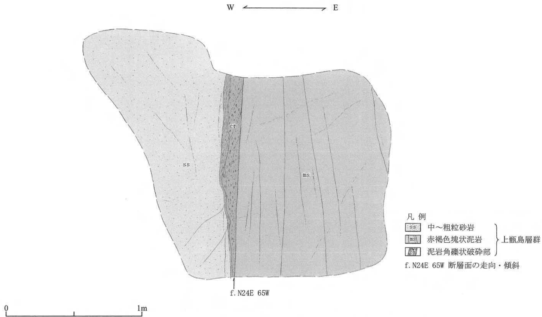
第1.2.3.2.2.58図(1) 露頭スケッチ (Loc.m1145、薩摩川内市江石北方)
