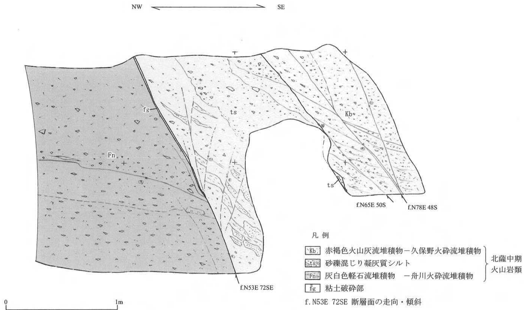
第1.2.3.2.2.28図(2) 露頭スケッチ (Loc.m87、いちき串木野市久保野西方)
