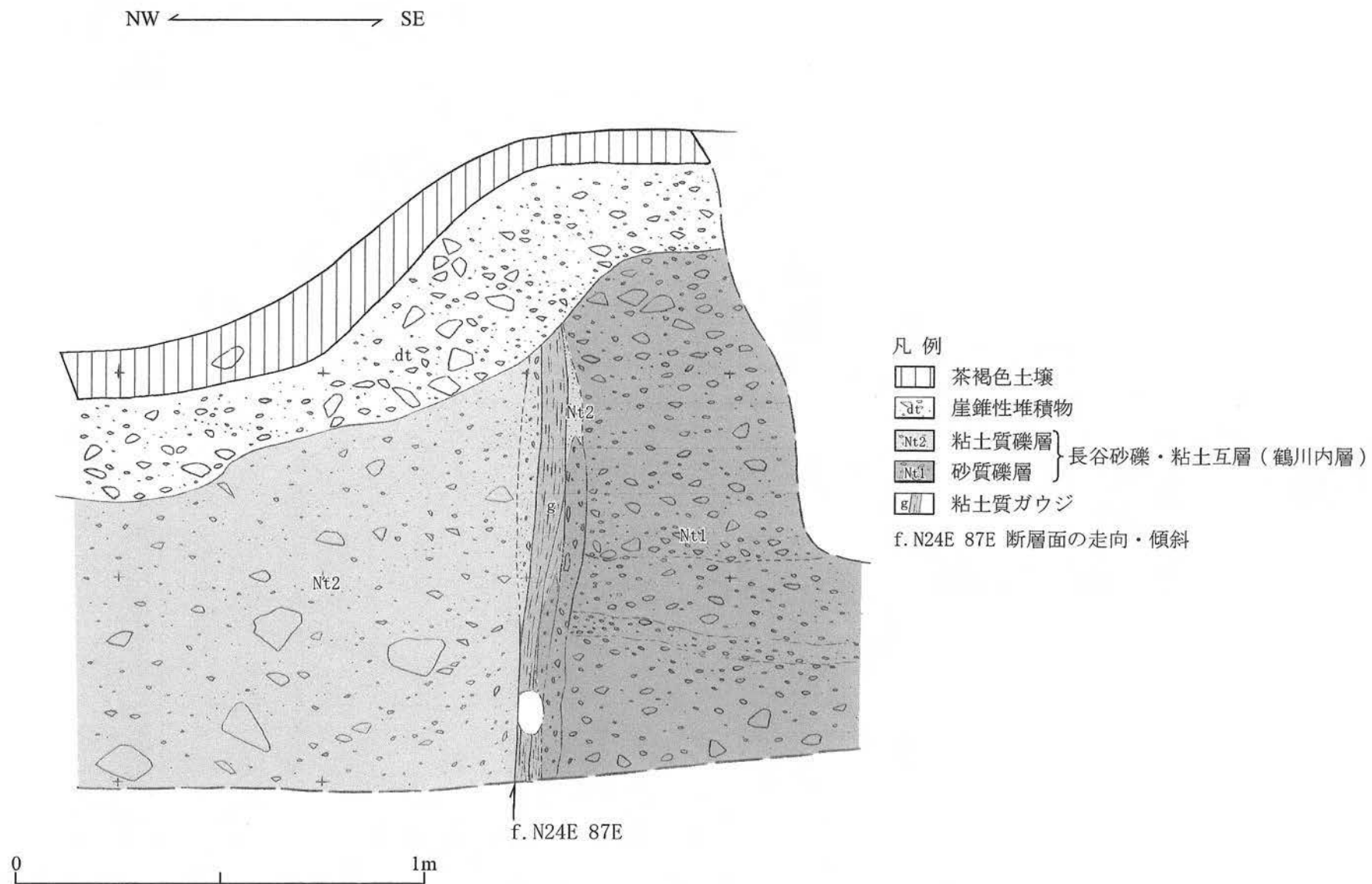
第1.2.3.2.2.45図(3) 露頭スケッチ(Loc.k805、出水市大丸)
