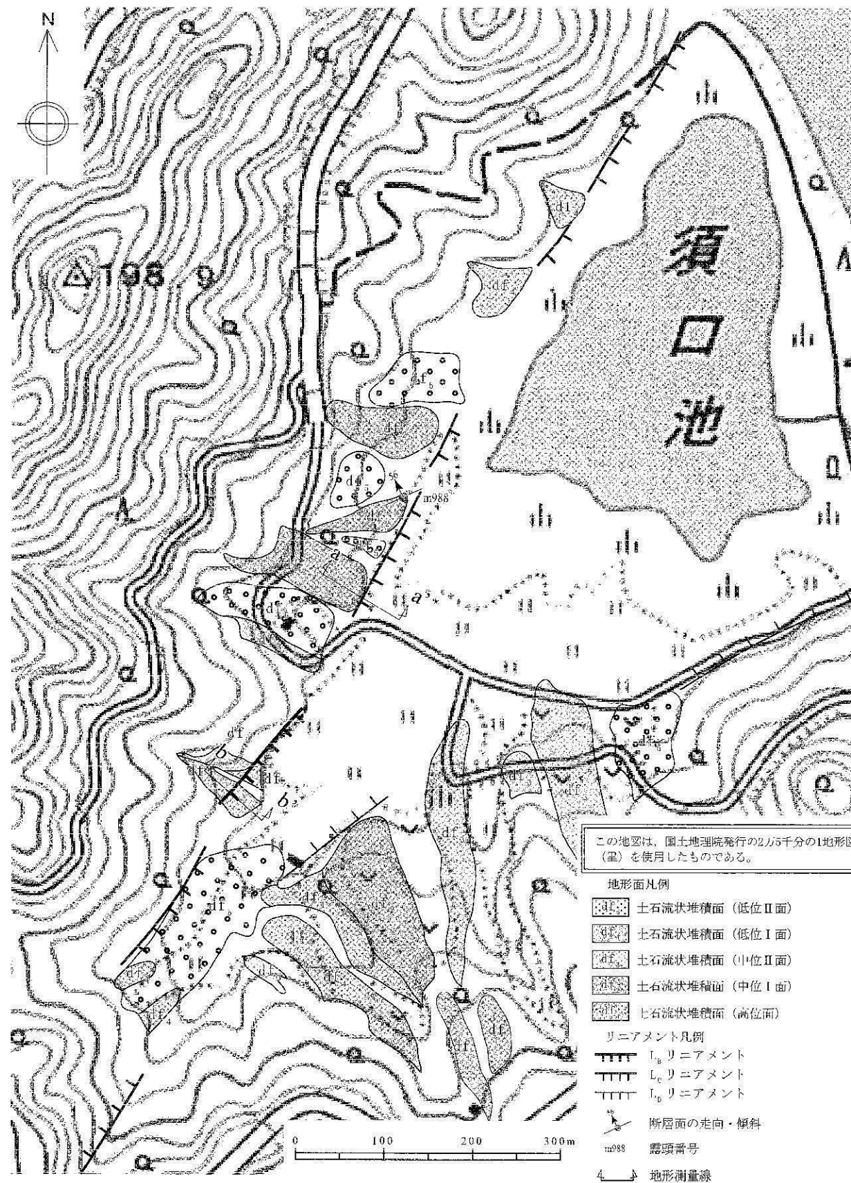
第1.2.3.2.2.55図 空中写真判読図・地形断面図(薩摩川内市須口池付近)
