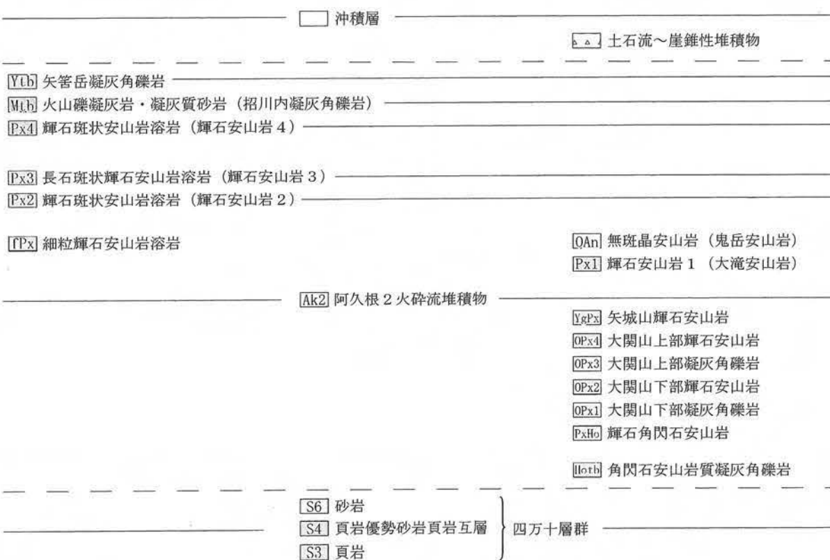
第1.2.3.2.2.38図(1) 出水断層系周辺の地質断面図(その1)
