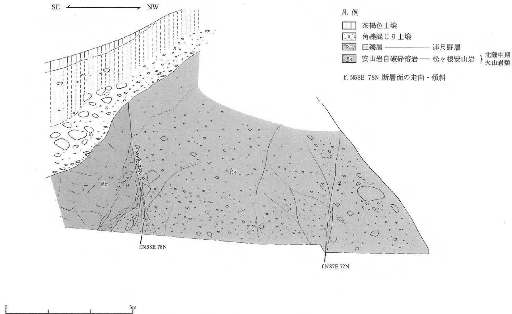
第1.2.3.2.2.53図 露頭スケッチ (Loc.t2191、出水市連尺野)
