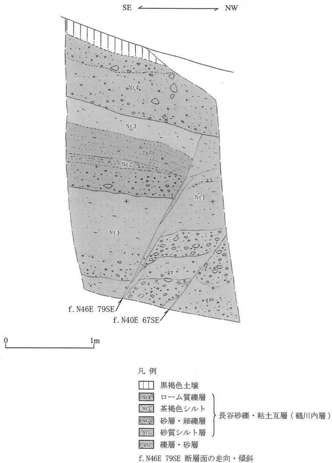
第1.2.3.2.2.45図(2) 露頭スケッチ (Loc.m1280、阿久根市梅)
