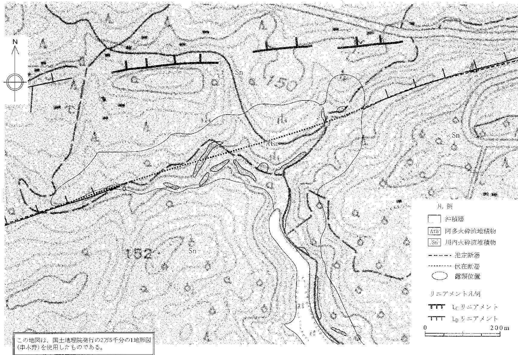
第1.2.3.2.2.29図 ルートマップ(日置市皆田西北方付近)
