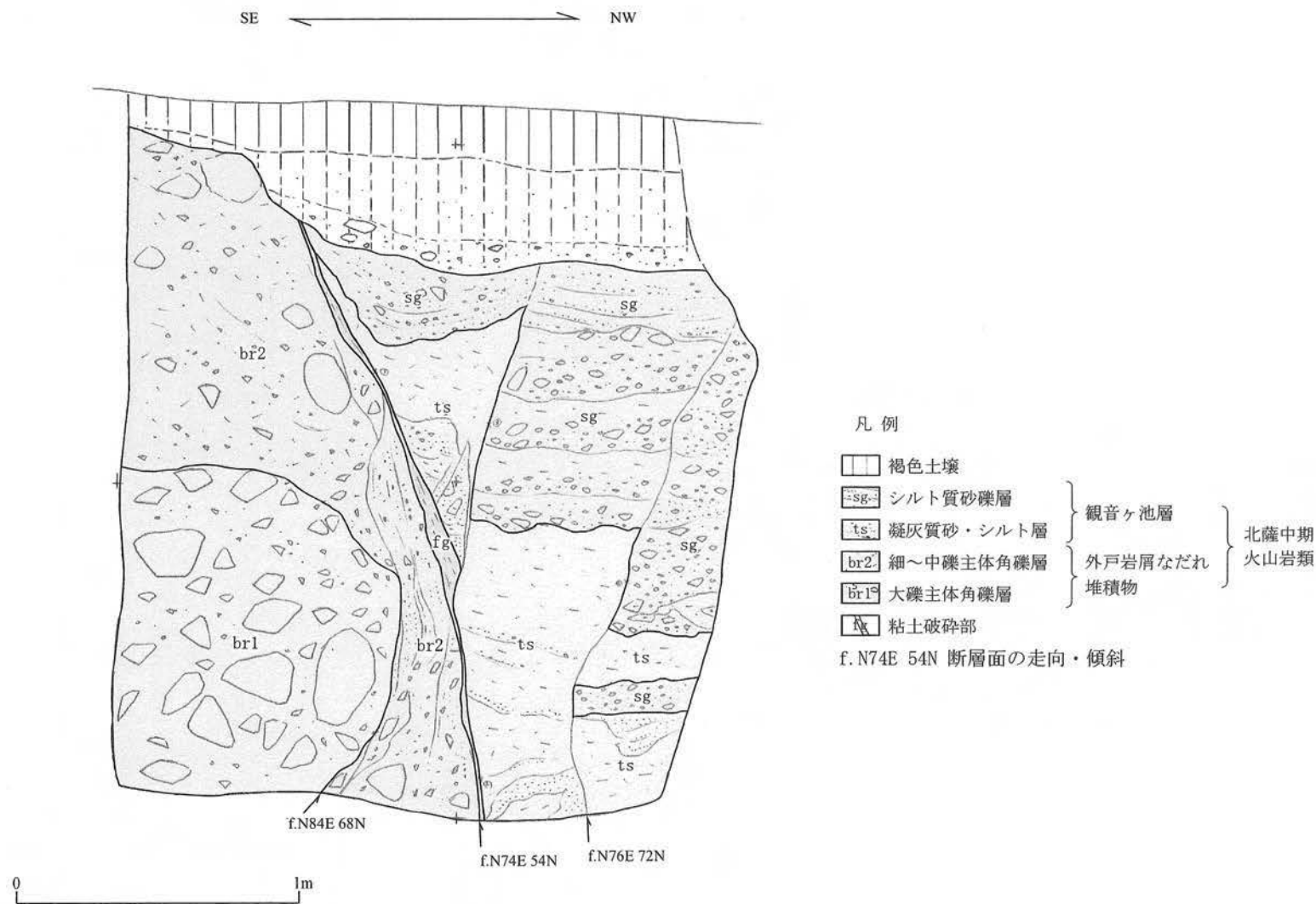
第1.2.3.2.2.28図(1) 露頭スケッチ (Loc.m291、いちき串木野市観音ヶ池西方)
