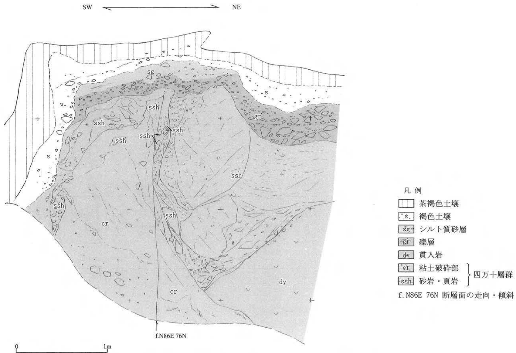
第1.2.3.2.2.39図(1) 露頭スケッチ (Loc.Y15、出水市内木場)
