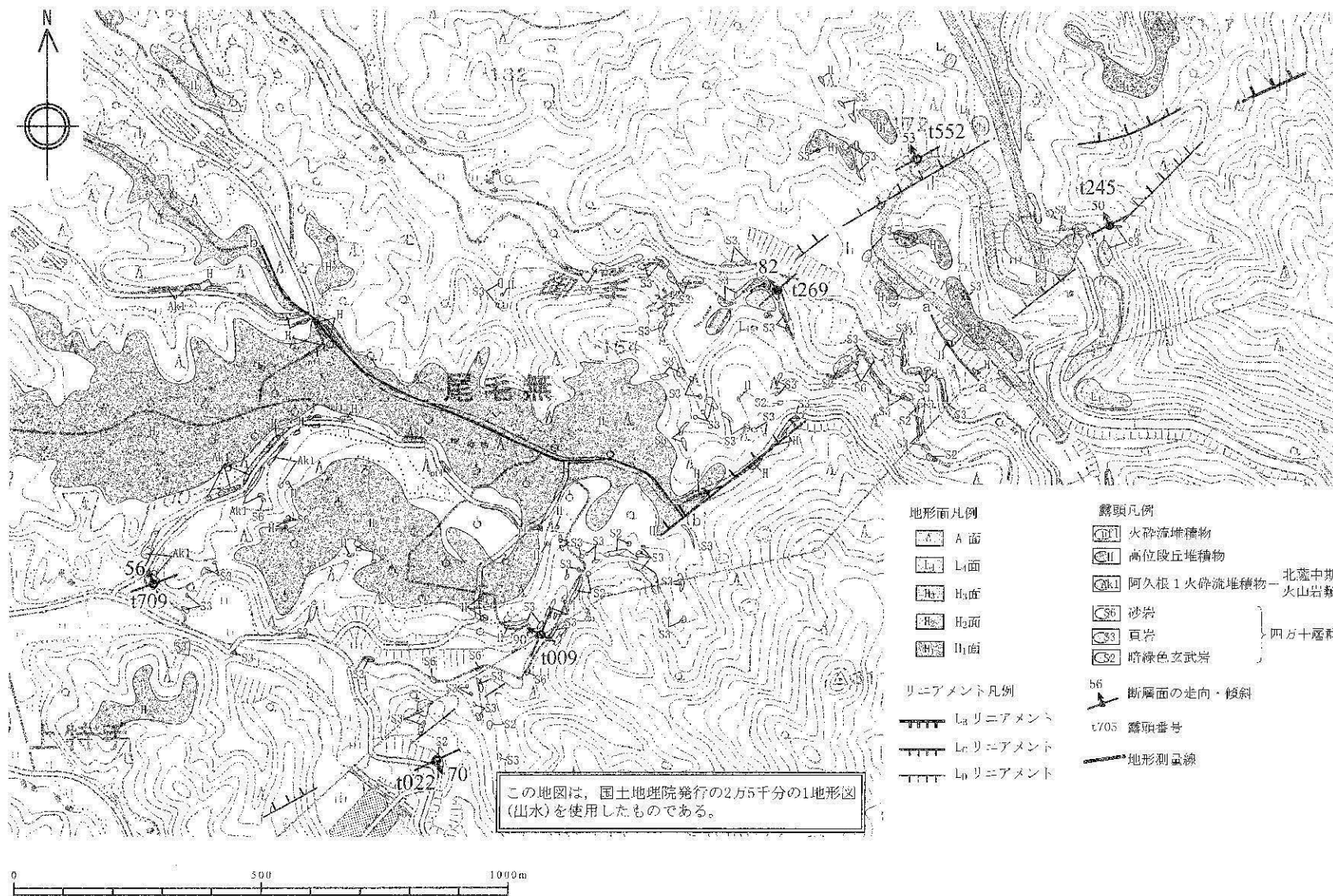
第1.2.3.2.2.41図(1) ルートマップ(出水市尾毛無付近)
