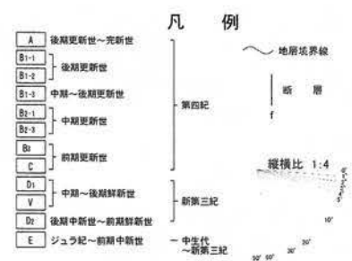
第1.2.3.2.2.68図(4) F-C断層の音波探査記録・海底地質断面図(s17測線)
