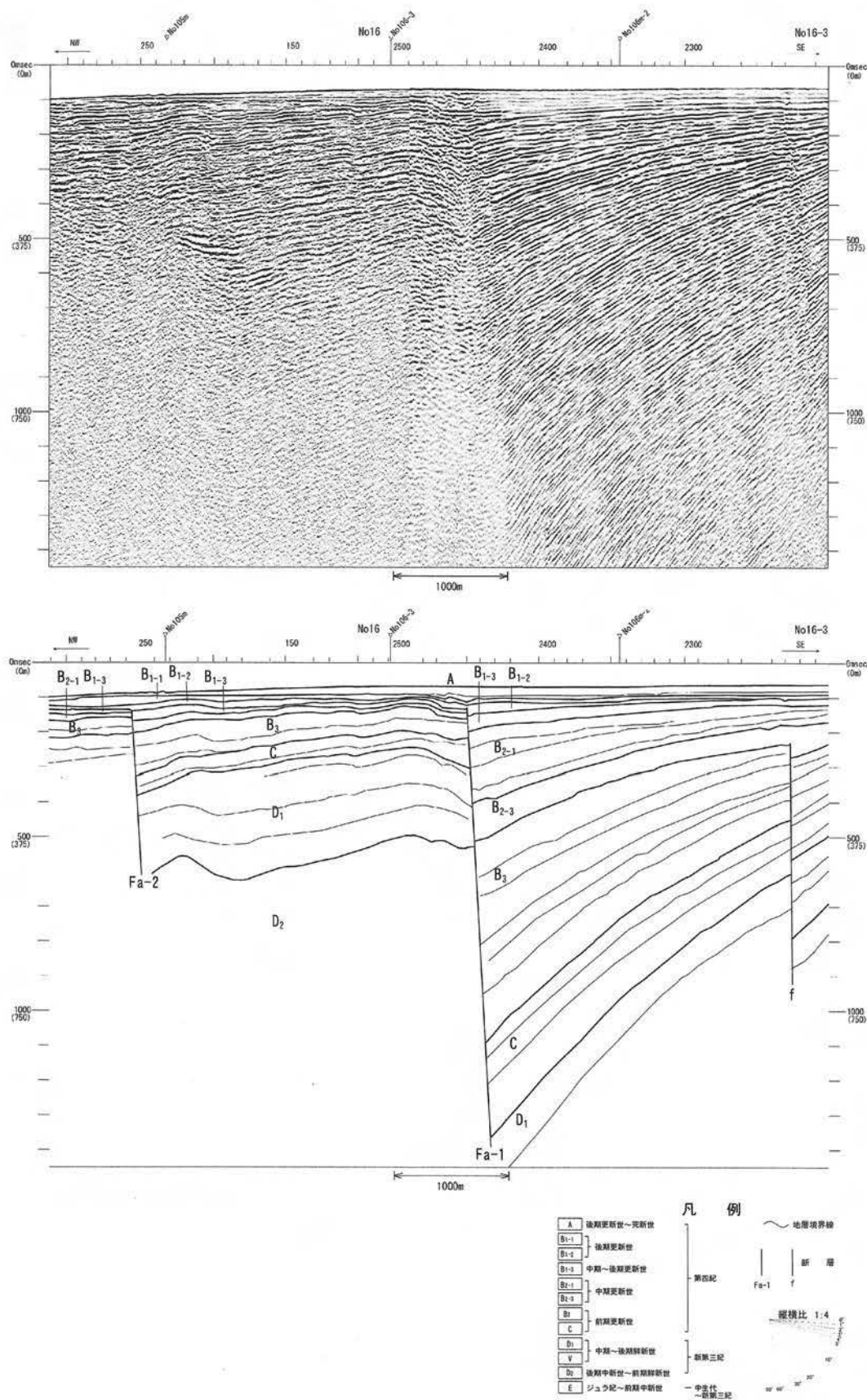
第1.2.3.2.2.66図(2) F-A断層の音波探査記録・海底地質断面図(No16測線)
