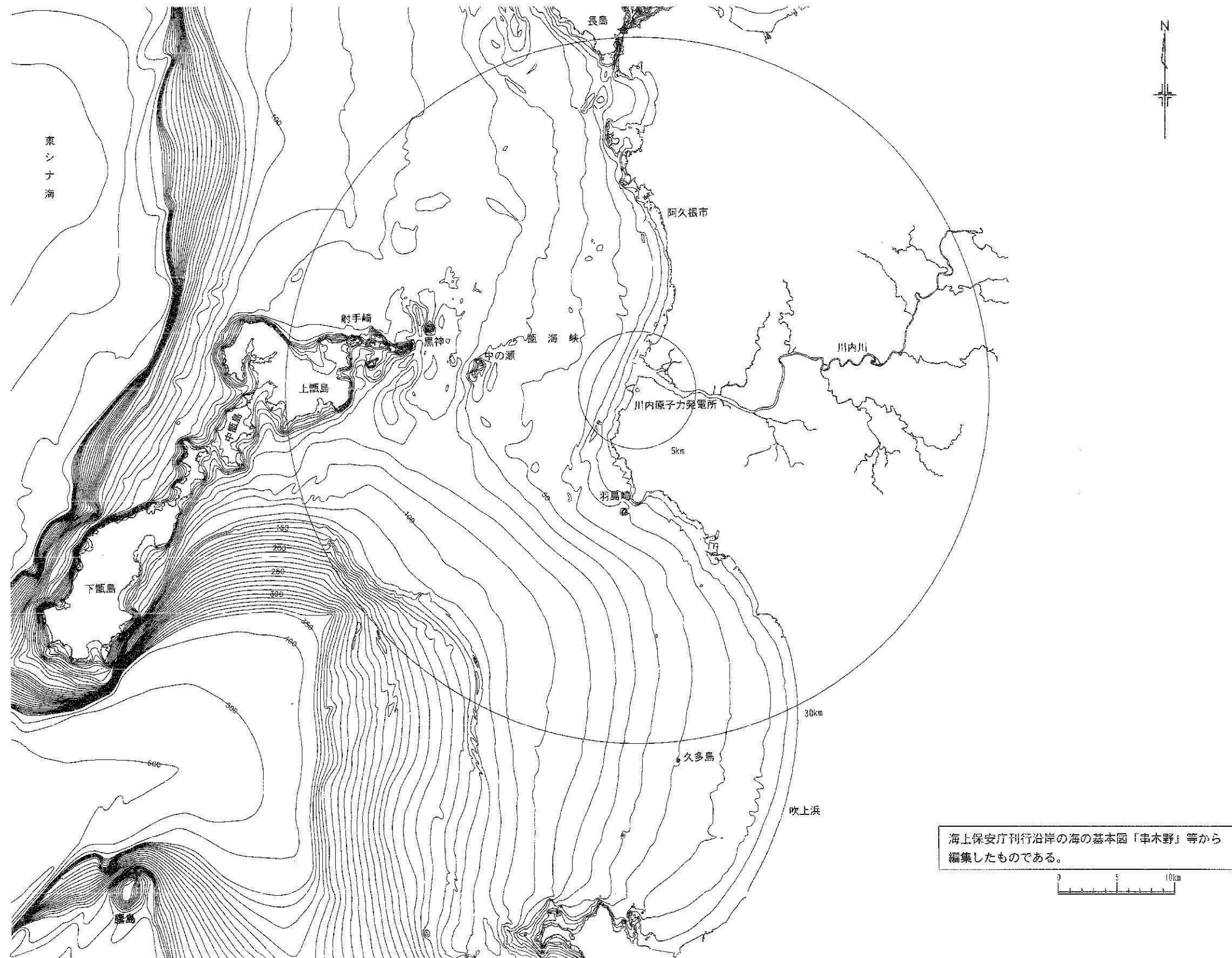
第1.2.3.2.2.60図 敷地前面海域の海底地形図
