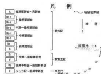
第1.2.3.2.2.71図(3) F-F断層の音波探査記録・海底地質断面図(s05測線)
