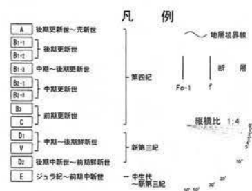
第1.2.3.2.2.68図(5) F-C断層の音波探査記録・海底地質断面図(s25測線)
