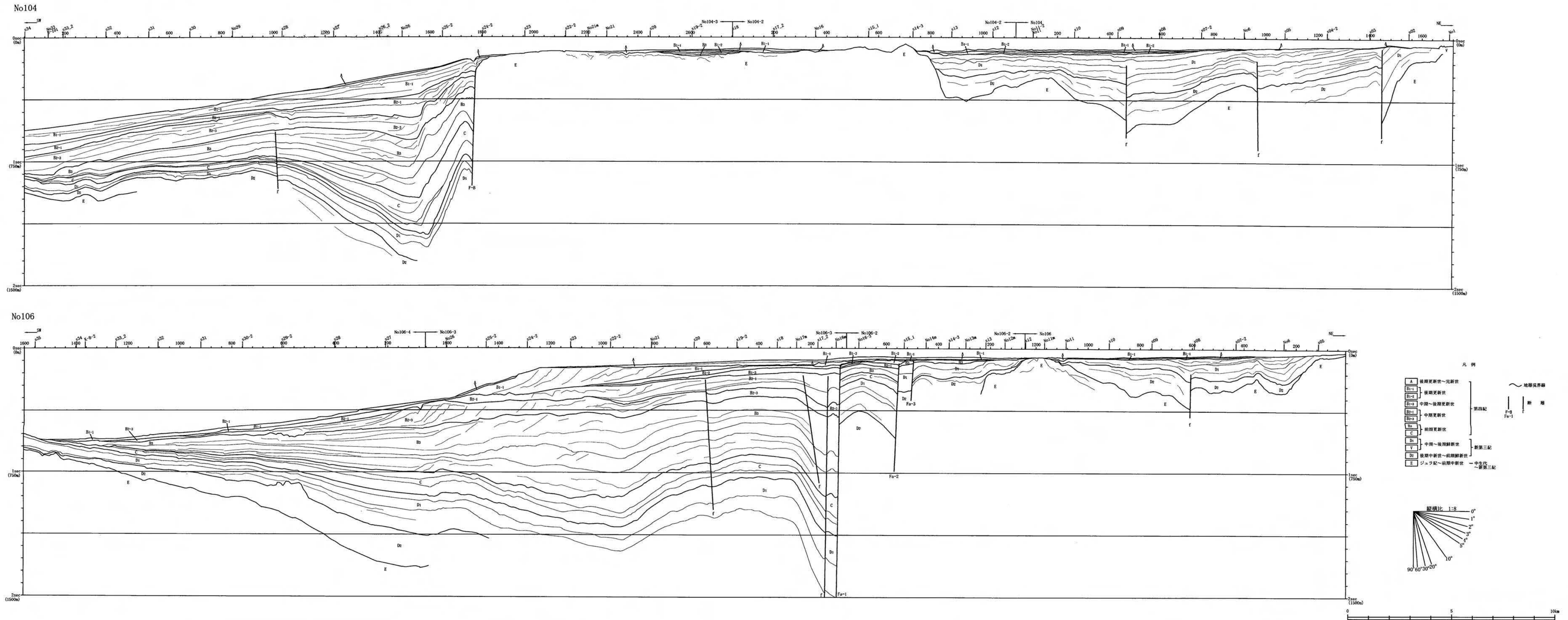
第1.2.3.2.2.62図(4) 敷地前面海域の海底地質断面図(その4)
