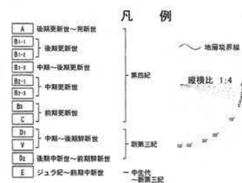
第1.2.3.2.2.71図(4) F-F断層の音波探査記録・海底地質断面図(s14測線)
