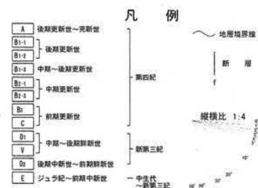
第1.2.3.2.2.66図(4) F-A断層の音波探査記録・海底地質断面図(s14測線)
