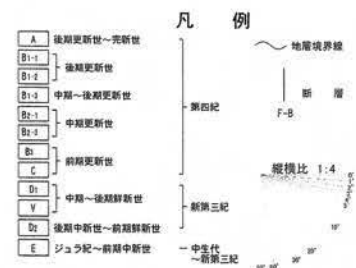
第1.2.3.2.2.67図(3) F-B断層の音波探査記録・海底地質断面図(s24測線)
