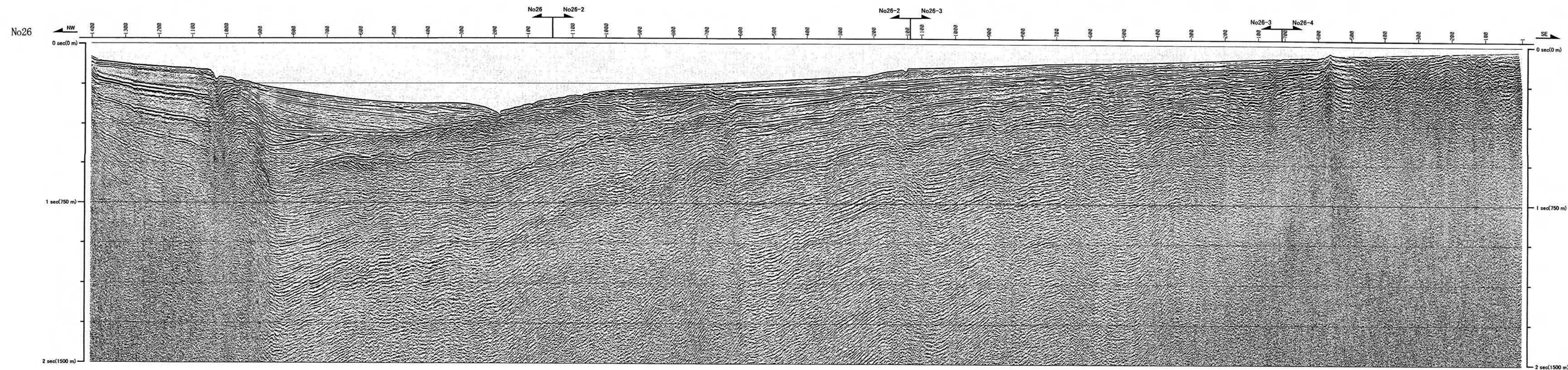
第1.2.3.2.2.63図(3) 敷地前面海域の音波探査記録(その3)
