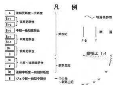
第1.2.3.2.2.69図(3) F-D断層の音波探査記録・海底地質断面図(No21測線)
