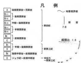
第1.2.3.2.2.67図(2) F-B断層の音波探査記録・海底地質断面図(No26測線)
