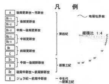
第1.2.3.2.2.70図(4) F-E断層の音波探査記録・海底地質断面図(No16測線)
