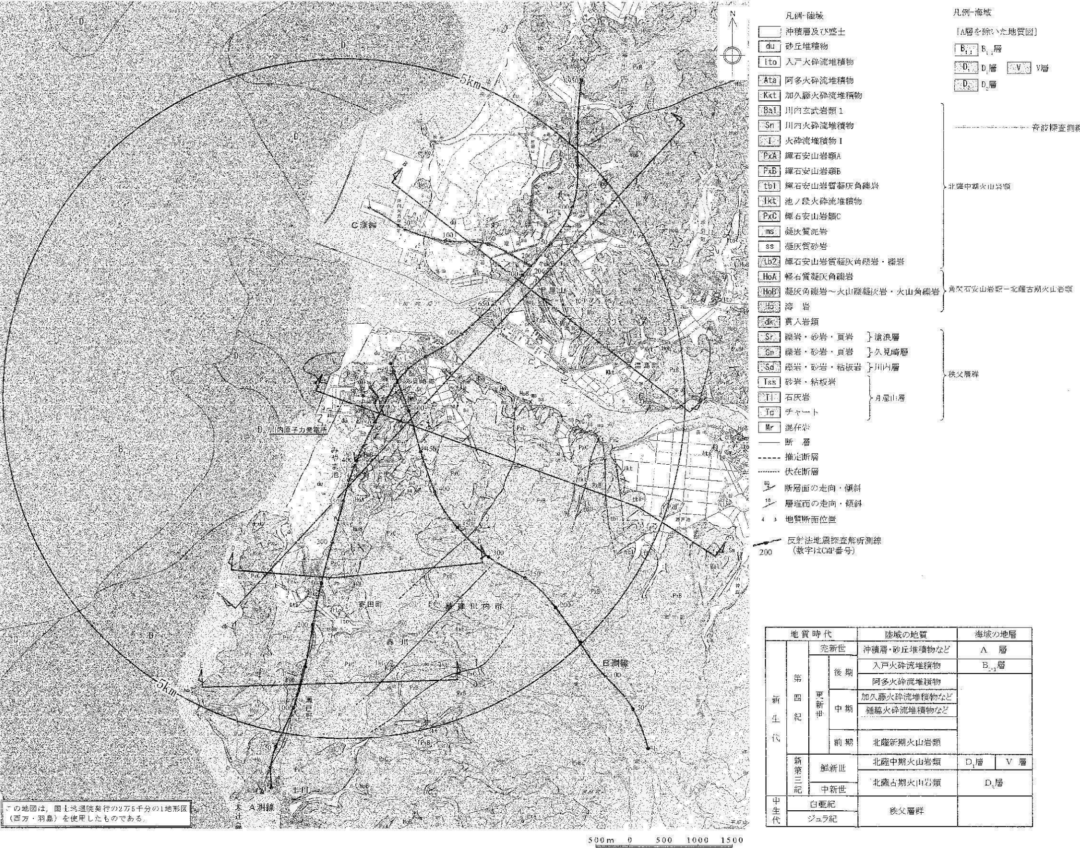
第1.2.3.2.3.2図 敷地近傍の地質図
