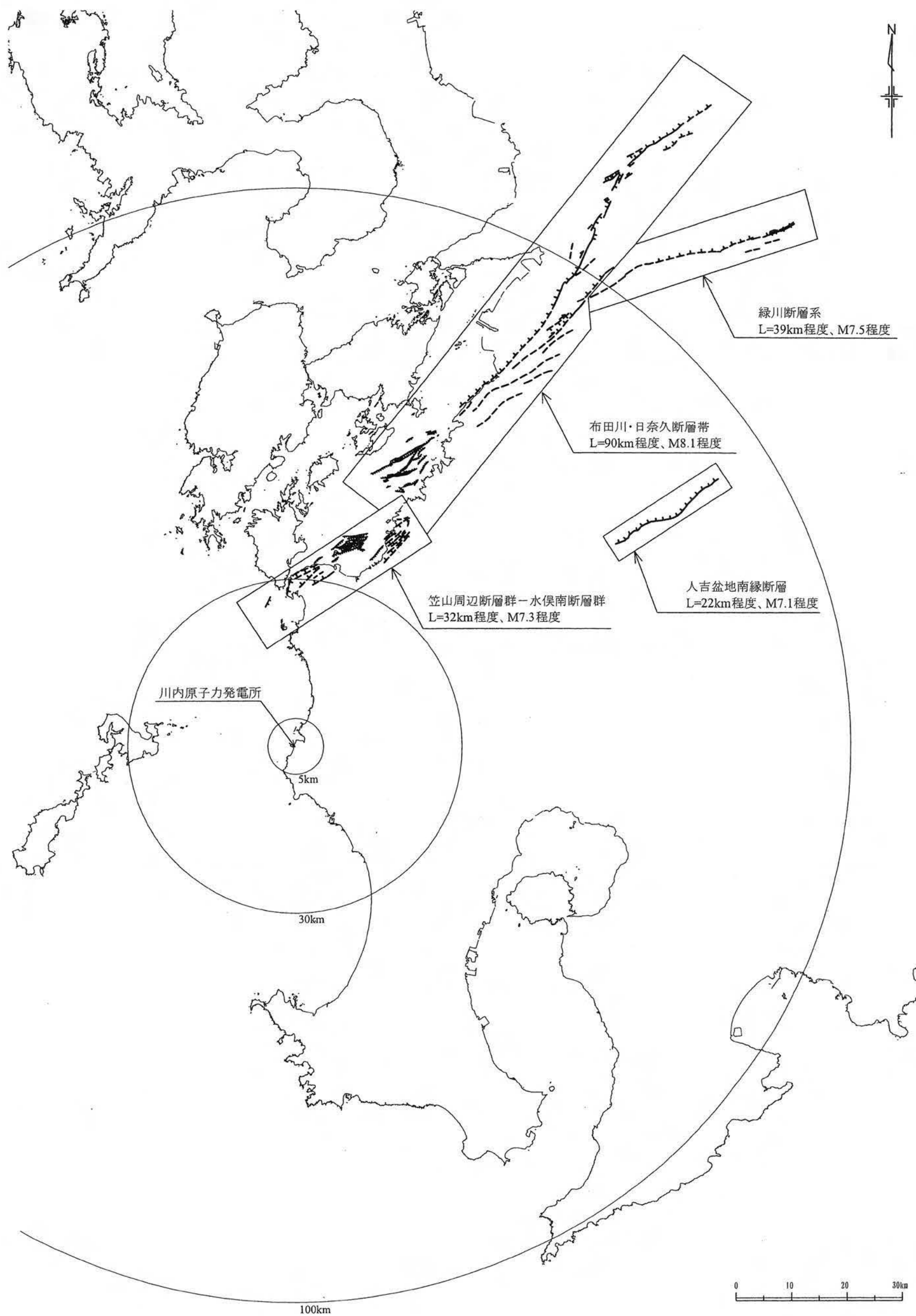
第1.2.3.2.2.59図 半径30km以遠の活断層分布図
