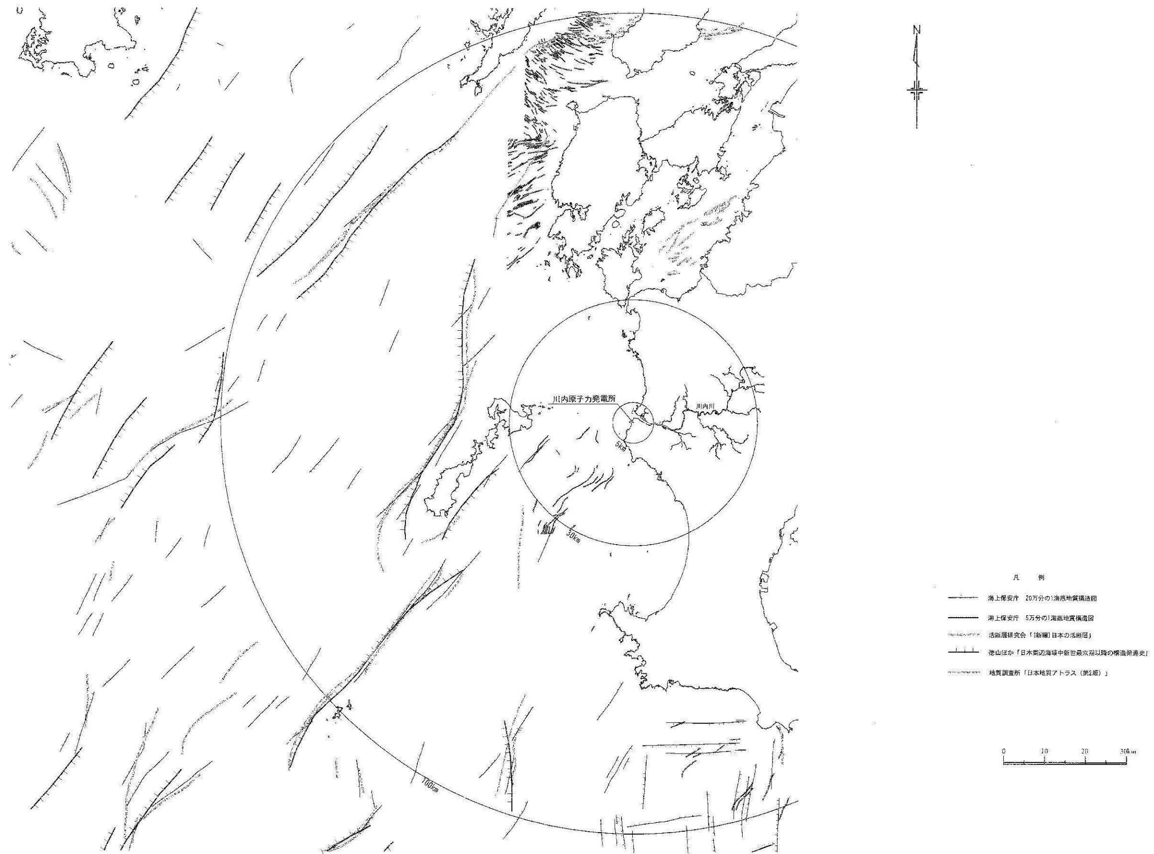
第1.2.3.2.2.64図 文献による敷地周辺海域の断層分布図
