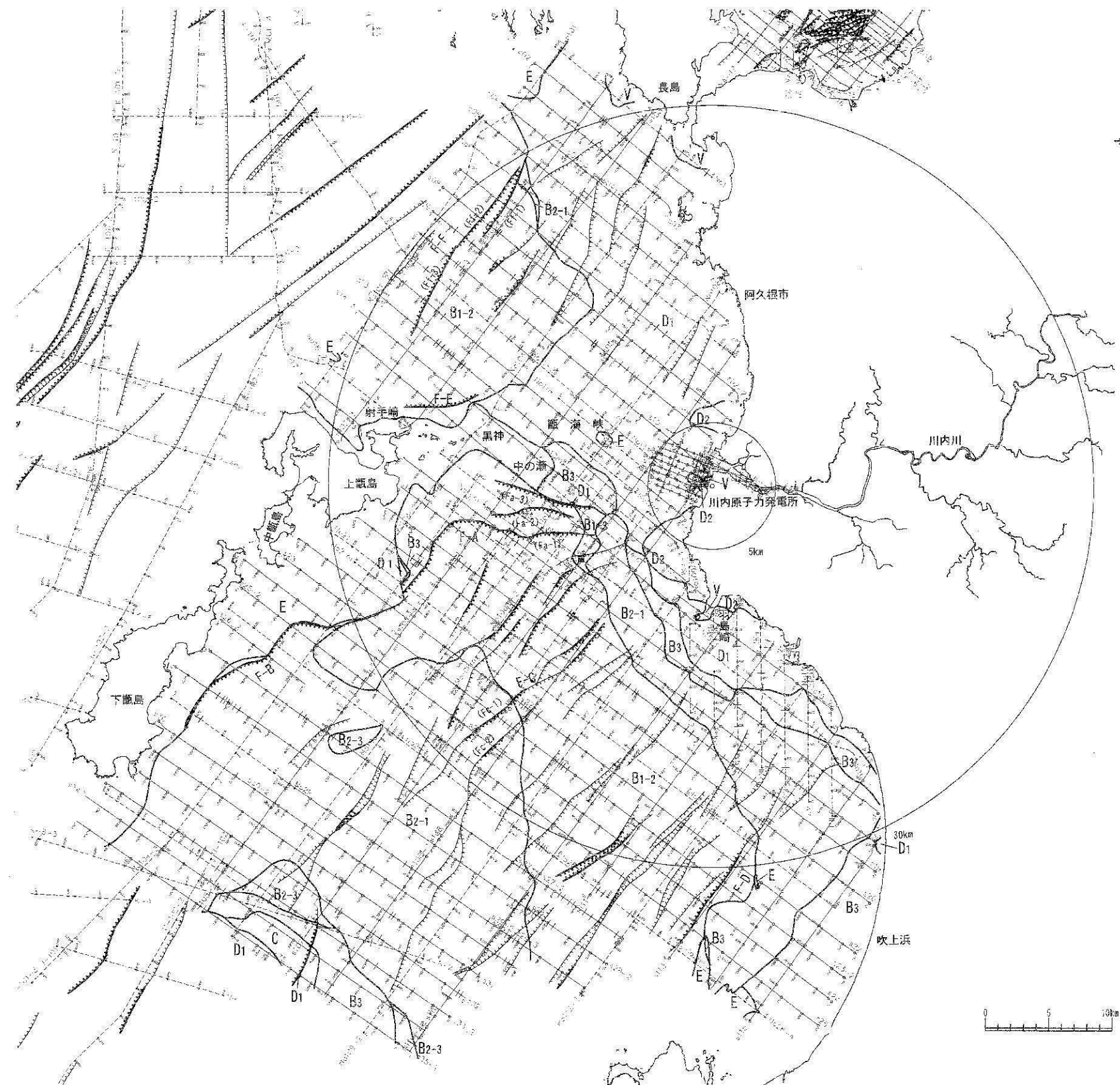
第1.2.3.2.2.61図 敷地前面海域の海底地質図
