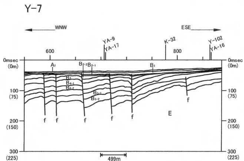
第1.2.3.2.2.73図(5) Fy-C断層群の音波探査記録・海底地質断面図(Y-7測線)
