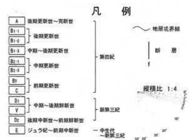
第1.2.3.2.2.70図(3) F-E断層の音波探査記録・海底地質断面図(s13測線)
