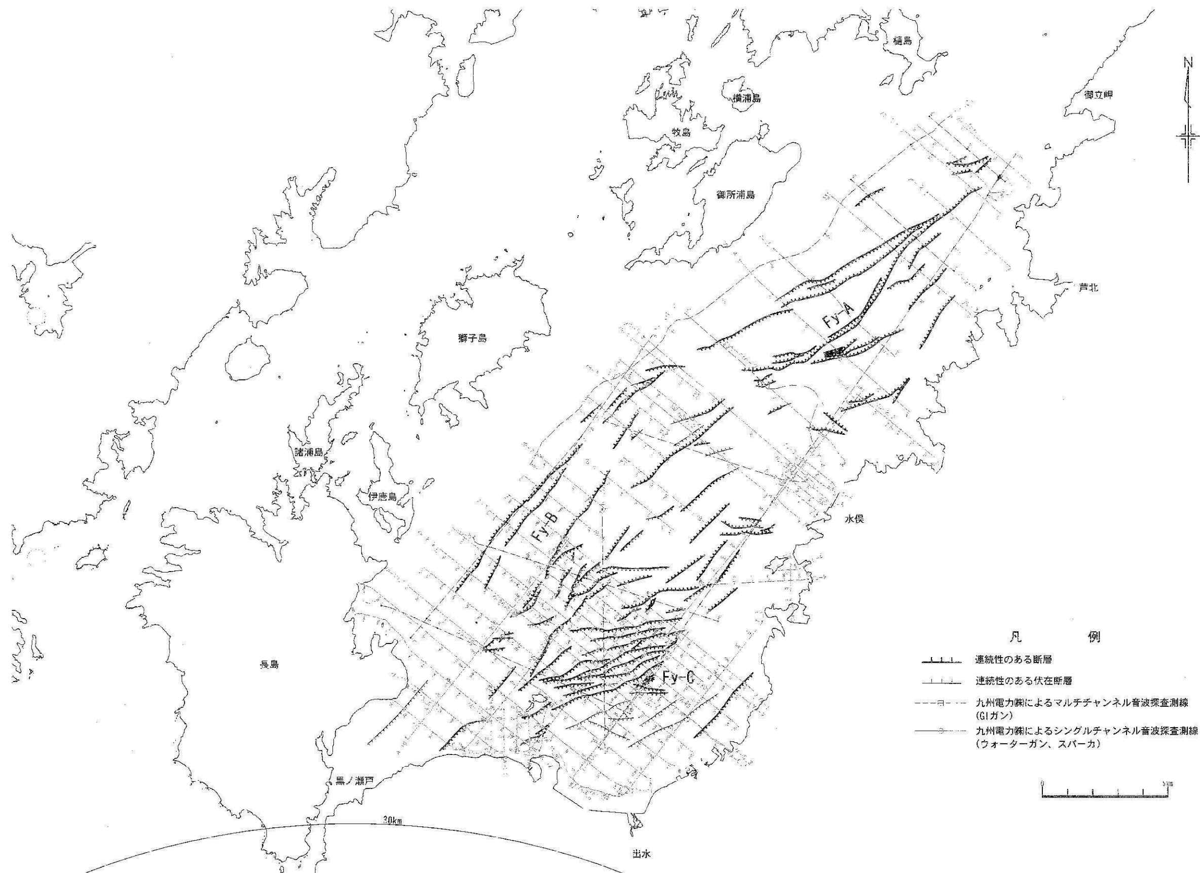
第1.2.3.2.2.73図(1) 八代海の断層分布図
