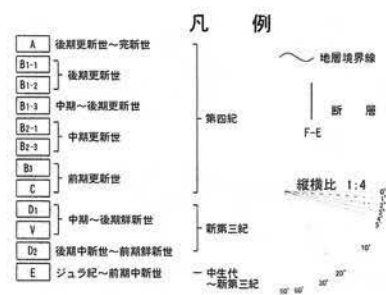
第1.2.3.2.2.70図(2) F-E断層の音波探査記録・海底地質断面図(s15測線)
