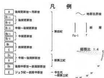
第1.2.3.2.2.68図(3) F-C断層の音波探査記録・海底地質断面図(s24測線)
