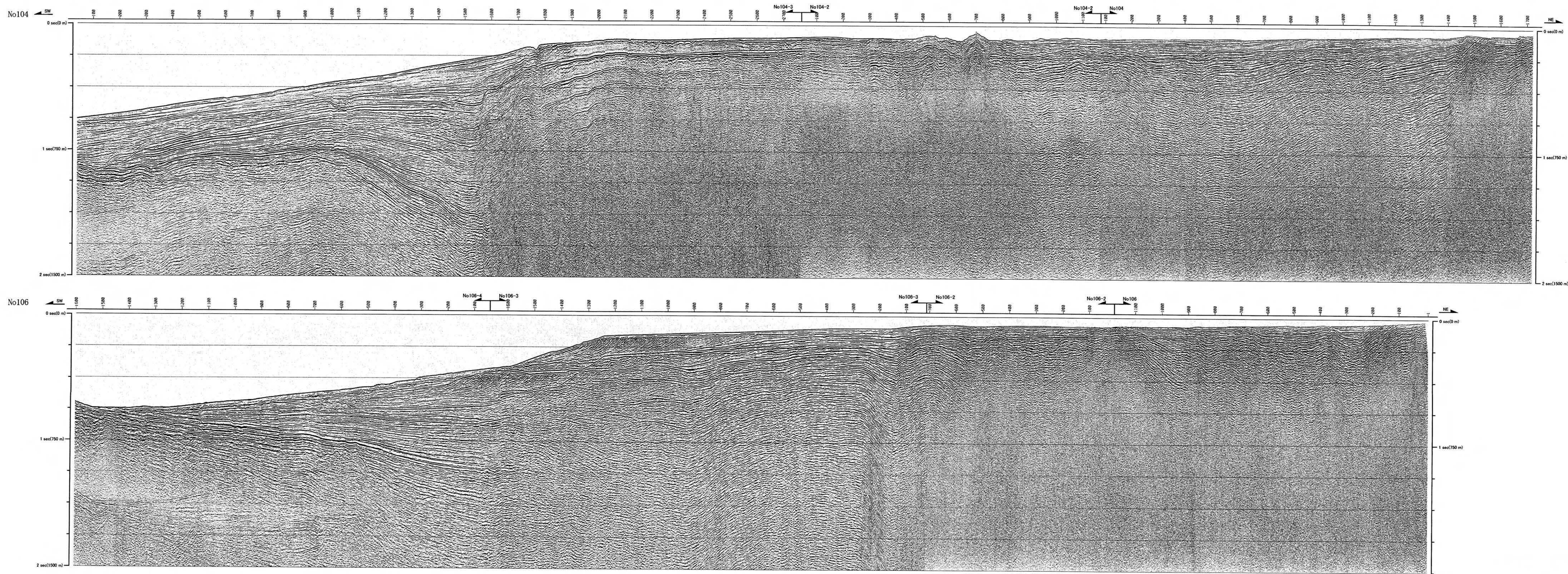
第1.2.3.2.2.63図(4) 敷地前面海域の音波探査記録(その4)
