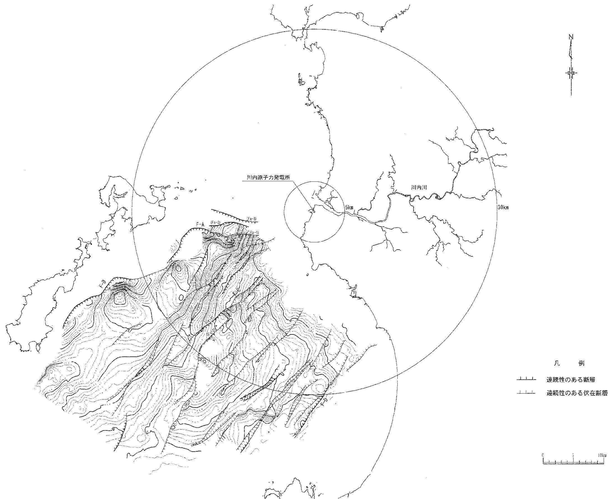
第1.2.3.2.2.65図 敷地前面海域のC層上面等深線図
