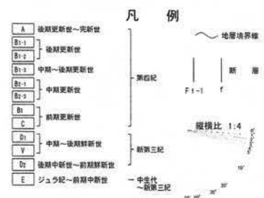
第1.2.3.2.2.71図(2) F-F断層の音波探査記録・海底地質断面図(s08測線)
