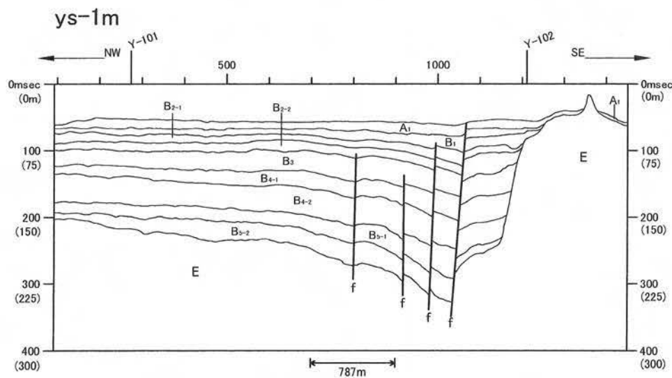
第1.2.3.2.2.73図(2) Fy-A断層群の音波探査記録・海底地質断面図(ys-1m測線)
