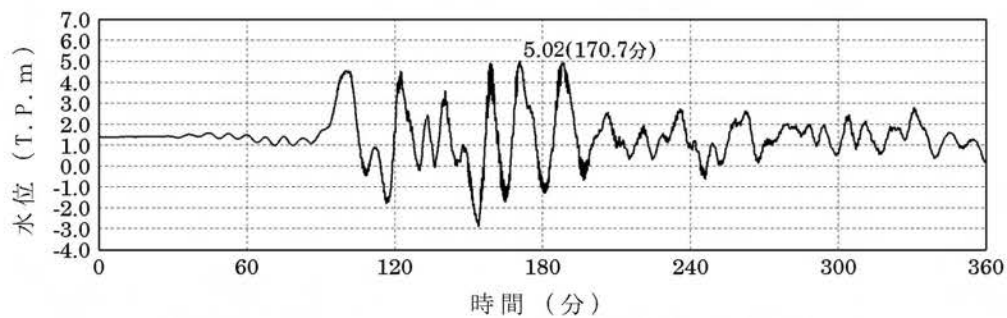
第 1.3.1.5.1 図 取水ピット時刻歴波形(上昇側)
