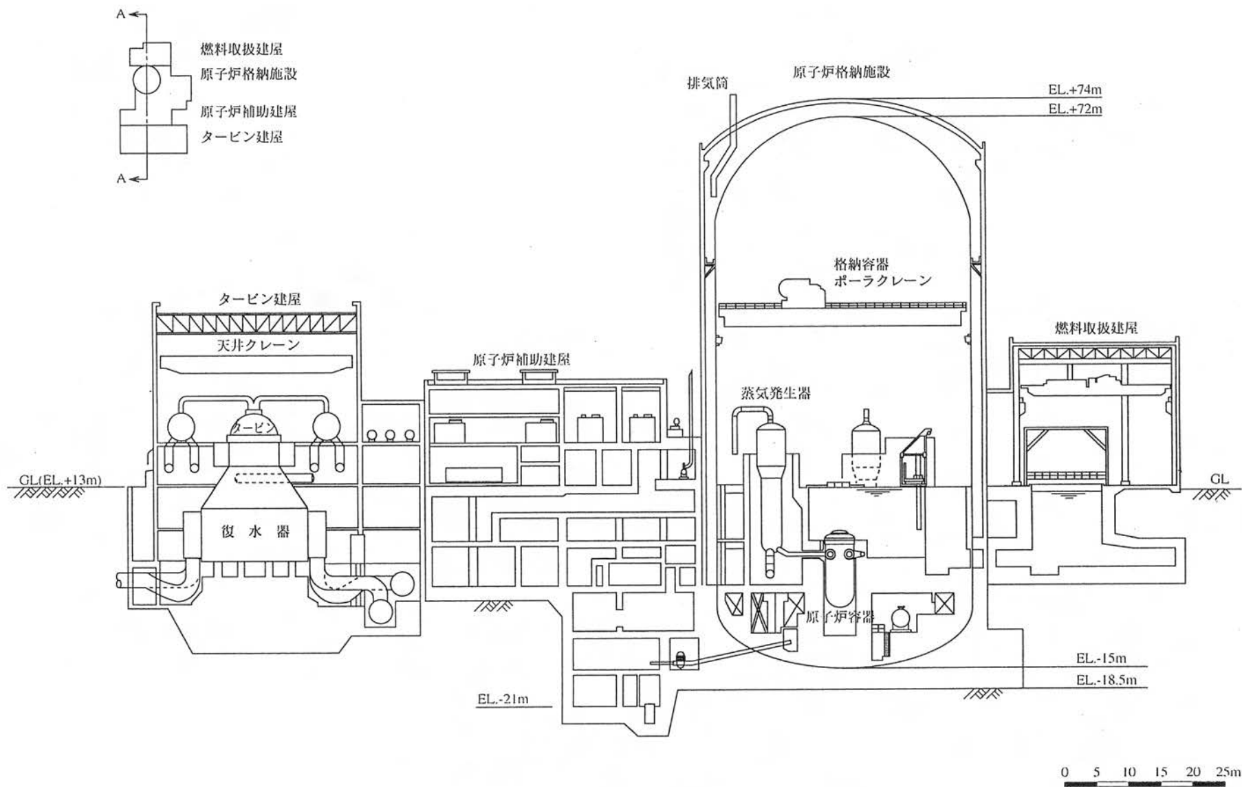
第1.3.2.5.6図 主要建屋断面図(A-A断面)
