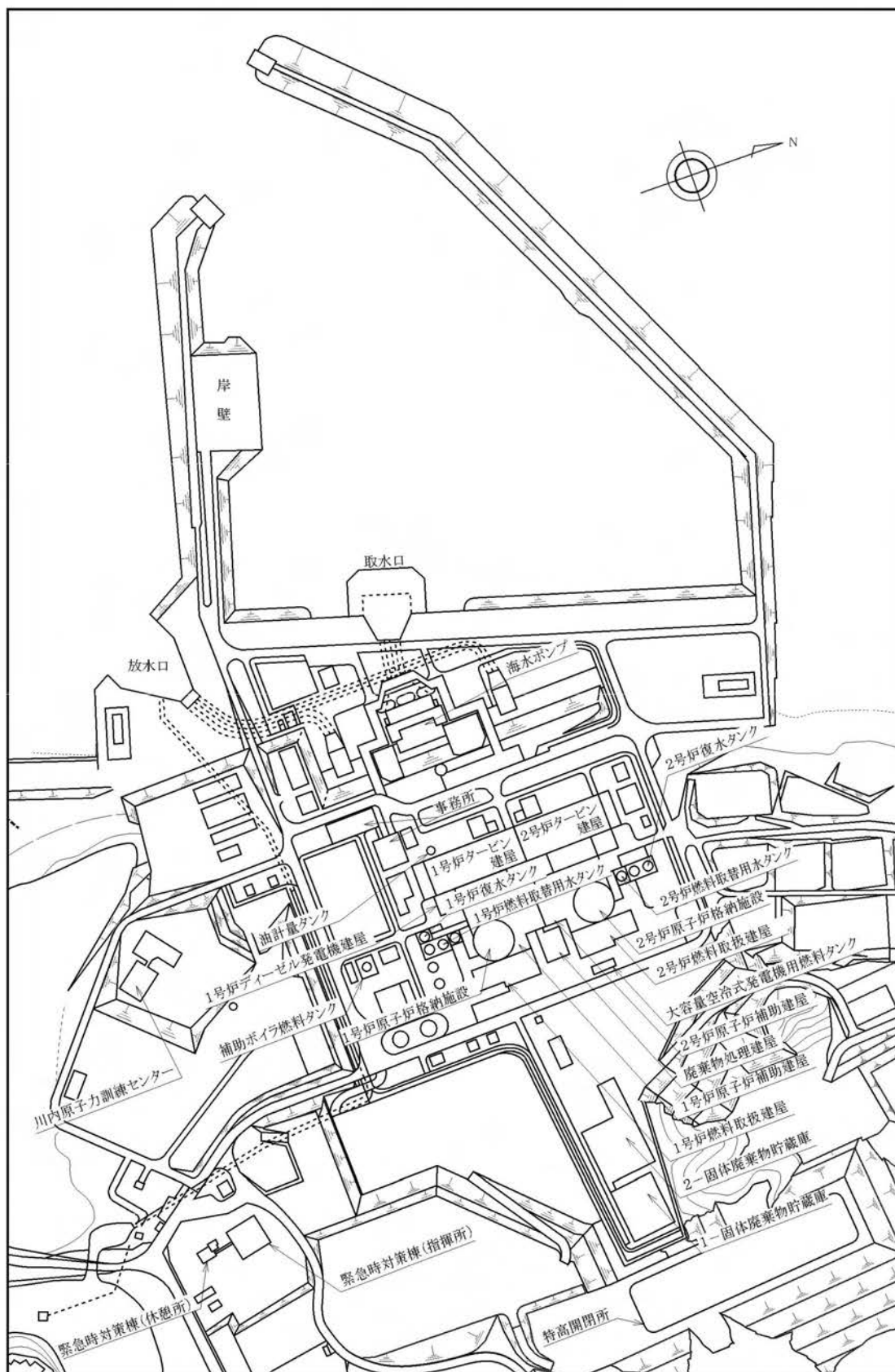
第 1.3.1.10.2 図 危険物タンク配置図
