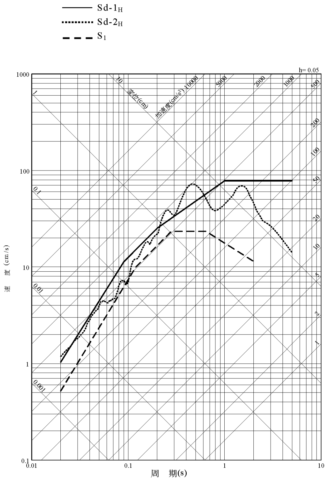
第 1.3.1.4.5 図 弾性設計用地震動と基準地震動S 1 の応答スペクトルの比較 (水平方向)
