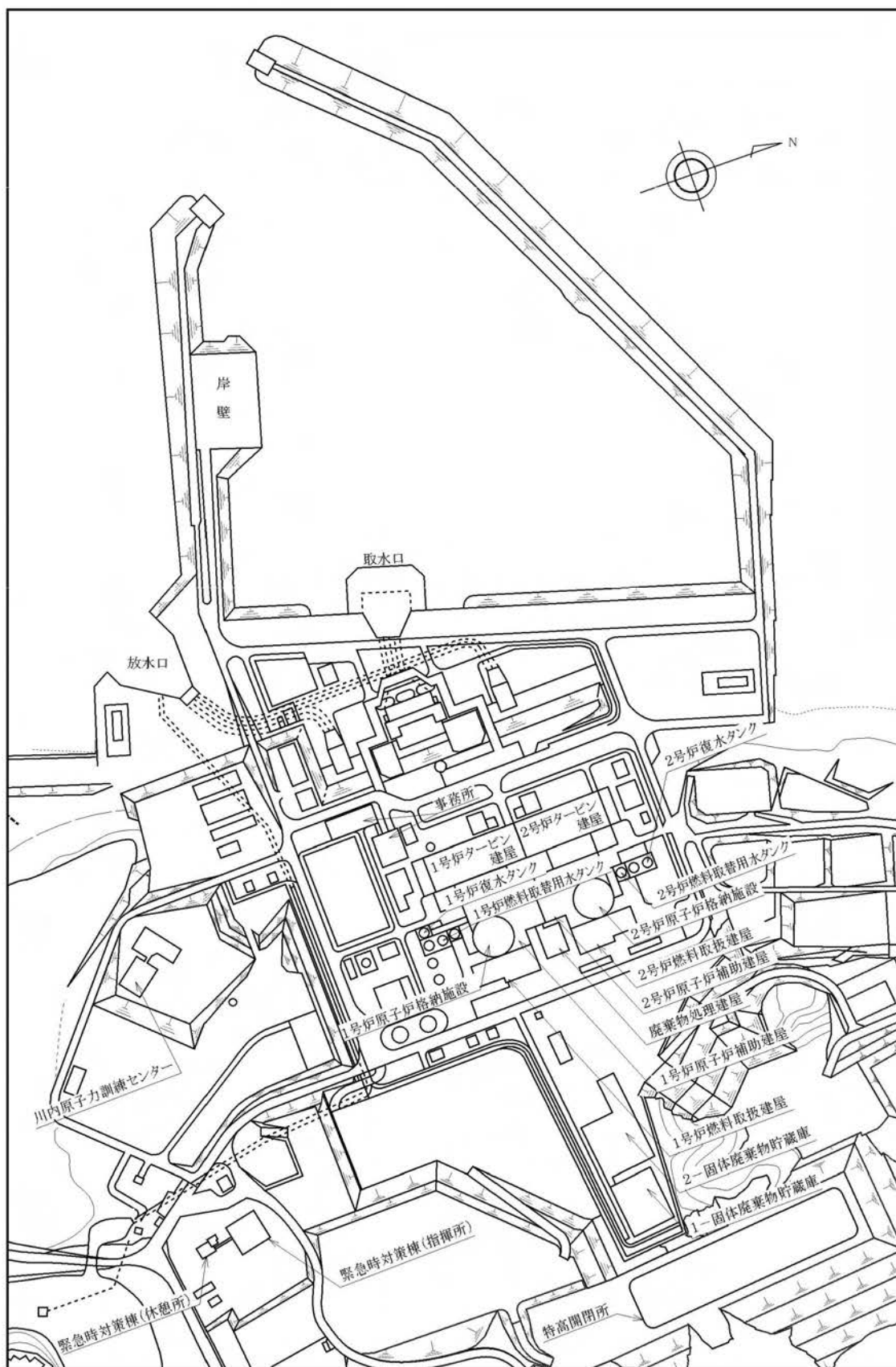
第1.3.2.4.1図 発電所全体配置図
