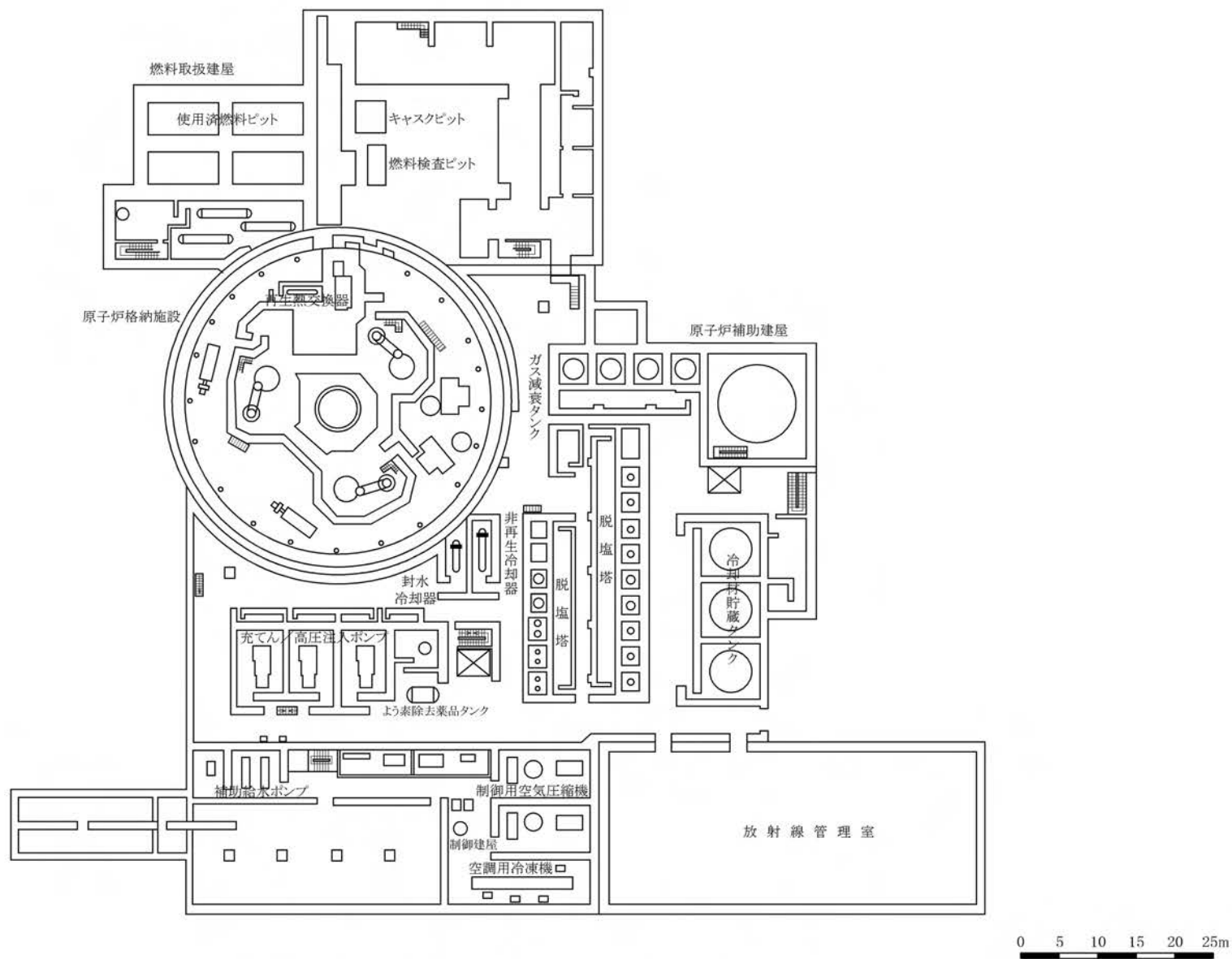
第1.3.2.5.2図 主要建屋平面図(地下2階)
