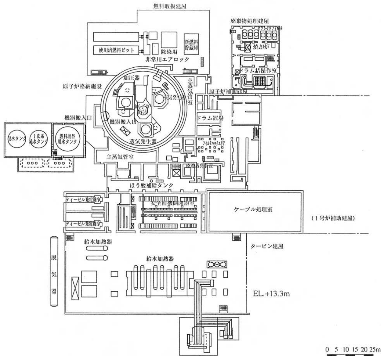
第1.3.2.5.4図 主要建屋平面図(1階)
