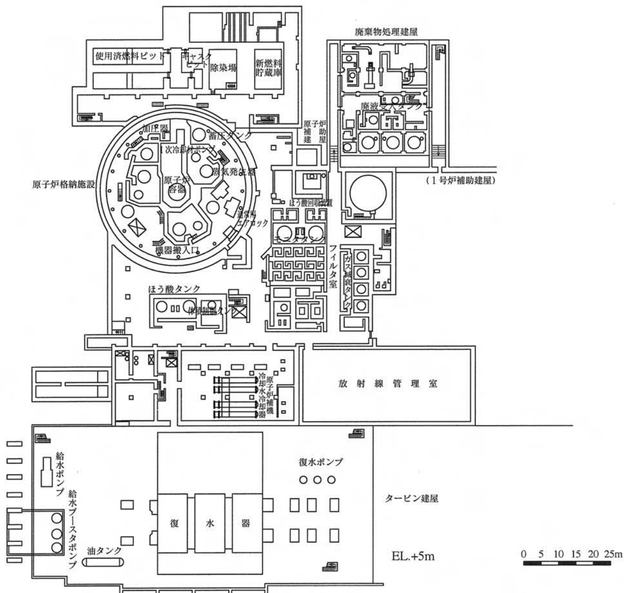
第1.3.2.5.3図 主要建屋平面図(地下1階)
