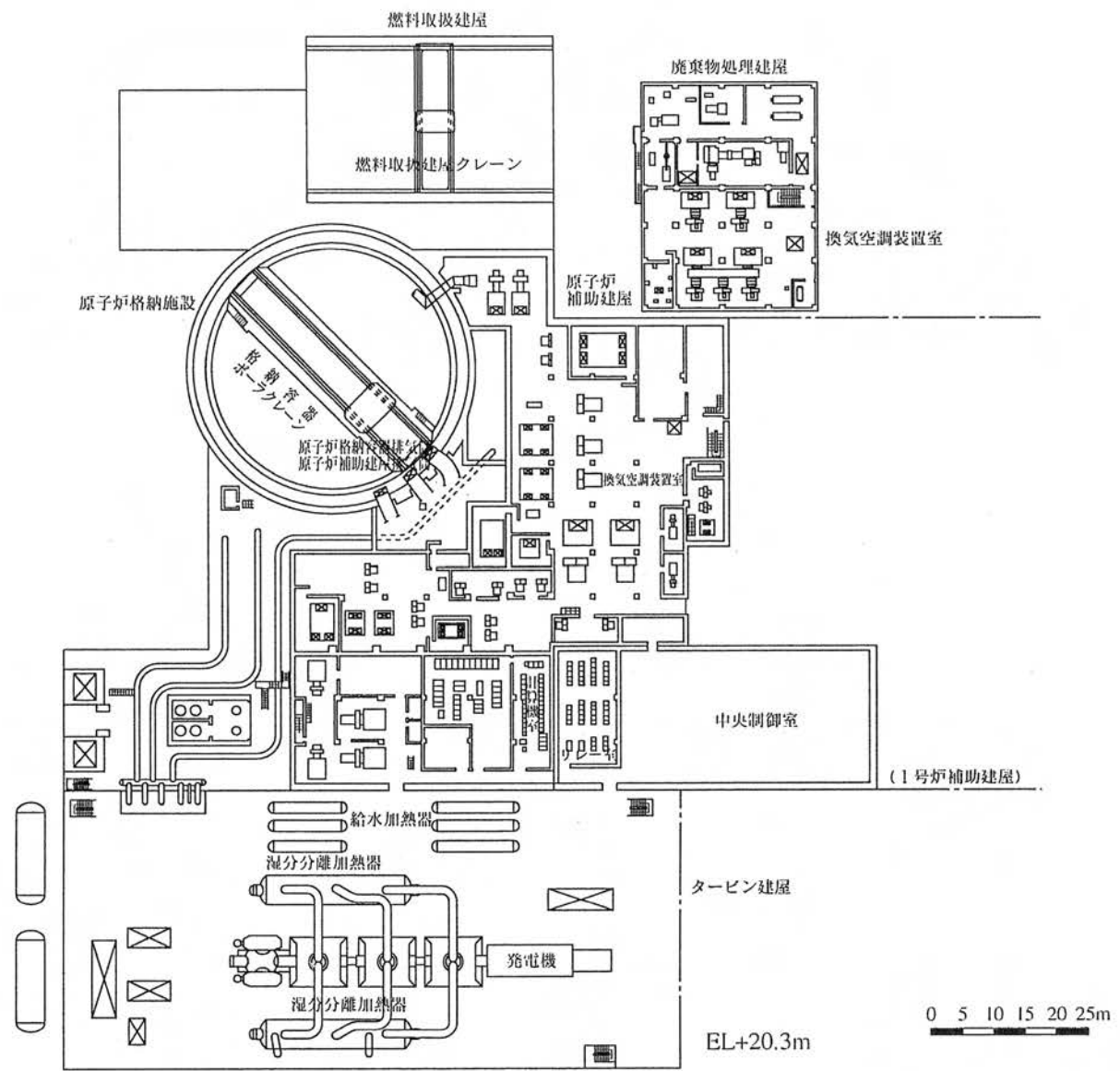
第1.3.2.5.5図 主要建屋平面図(2階)
