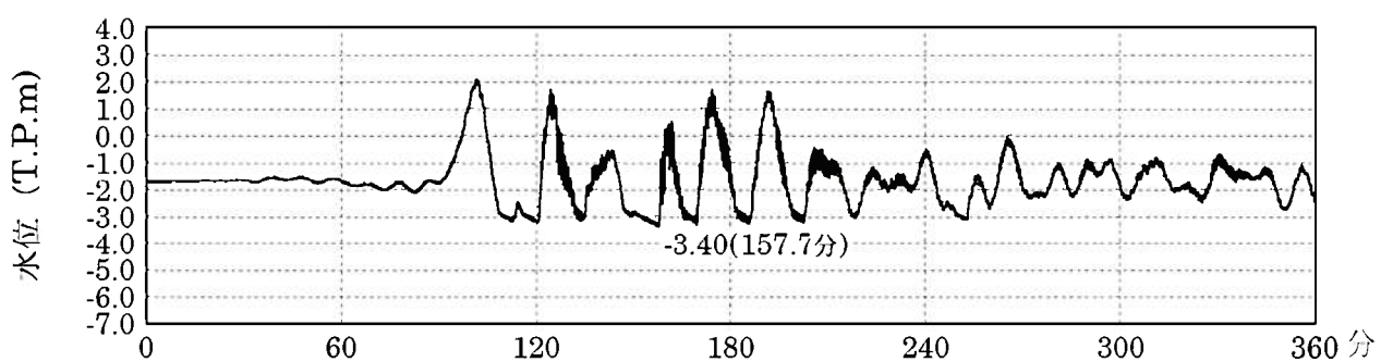
第1.2-26図(2) 取水ピットでの時刻歴波形
