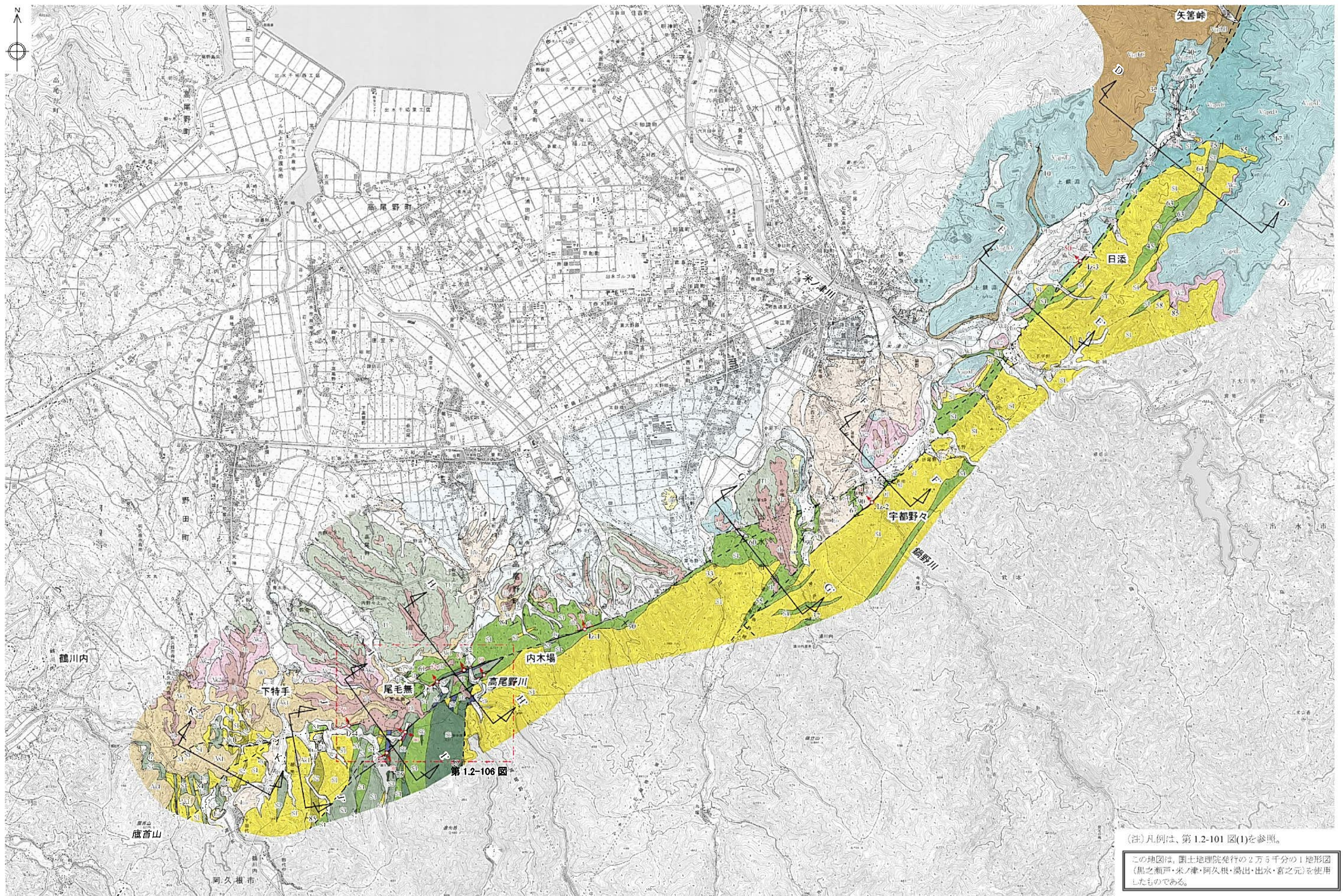
第1.2-101図(2) 出水断層系周辺の地質図(南部)
