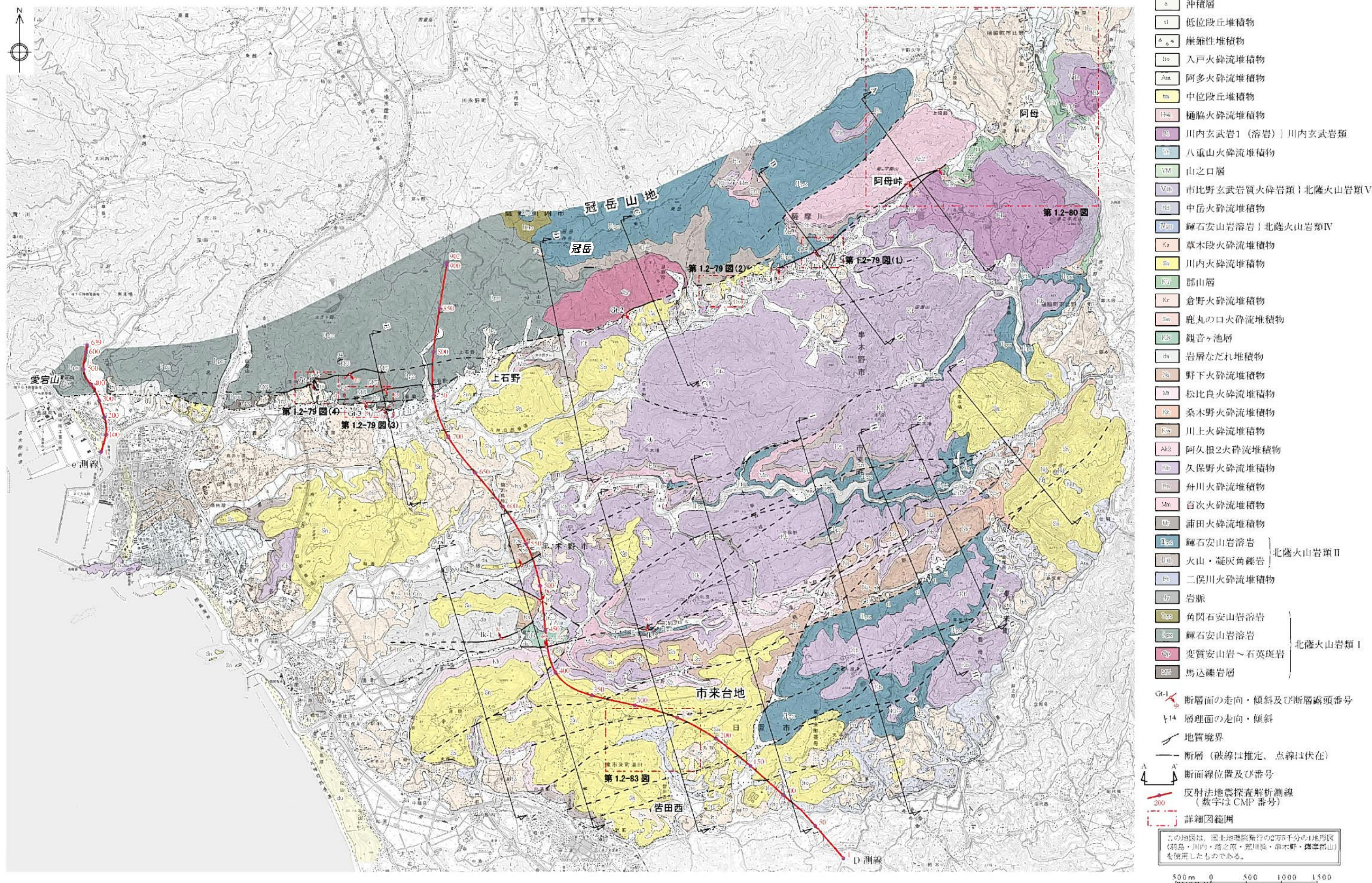
第1.2-74図 市来断層系周辺（五反田川断層含む）の地質図
