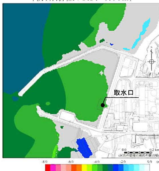
第1.2-23図(2) 基準津波の最大水位下降量分布
