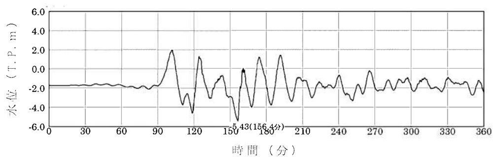
第1.3-4図 取水口時刻歴波形(下降側)
