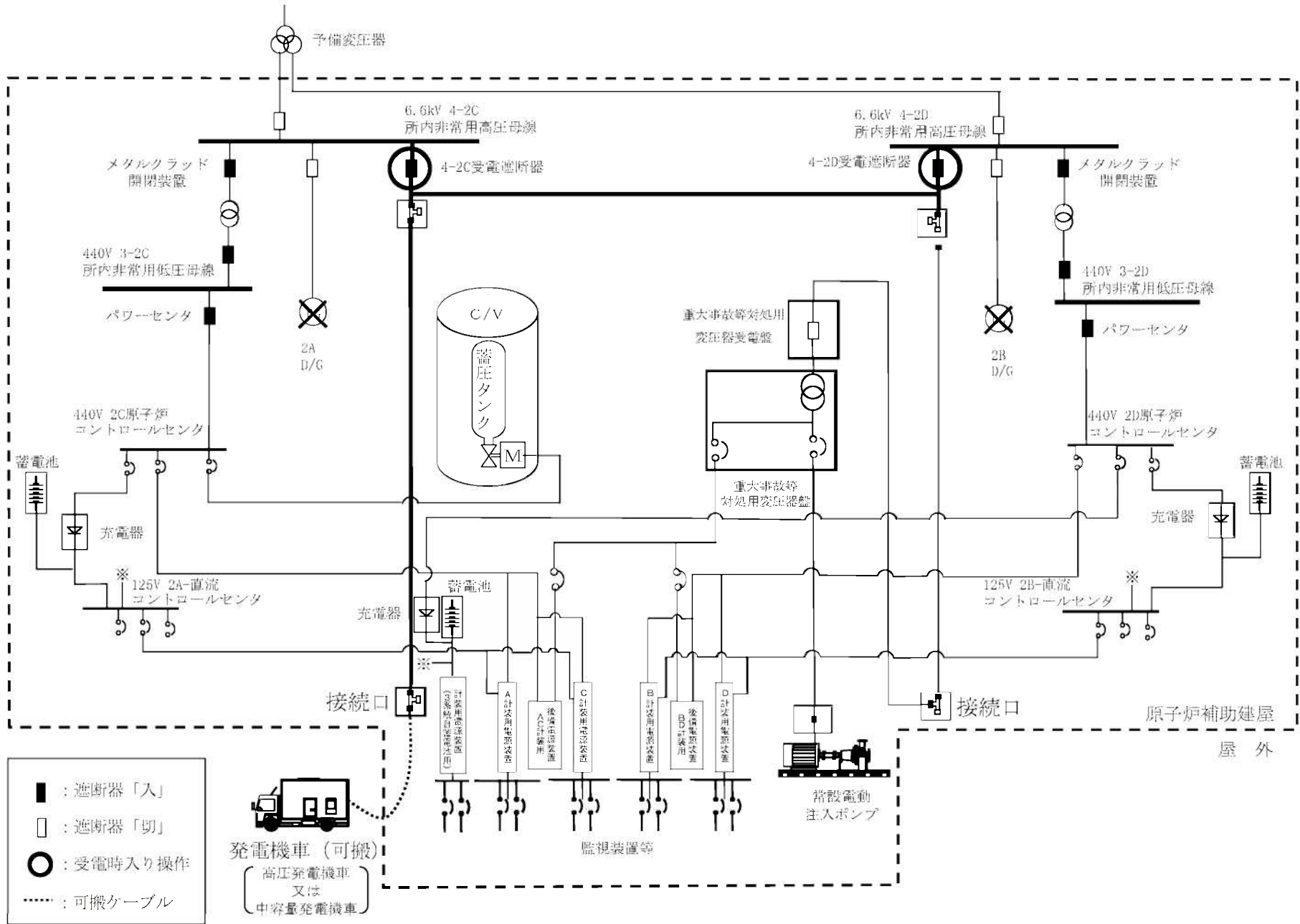
第1.8-3図 電源設備系統概要図(2)
