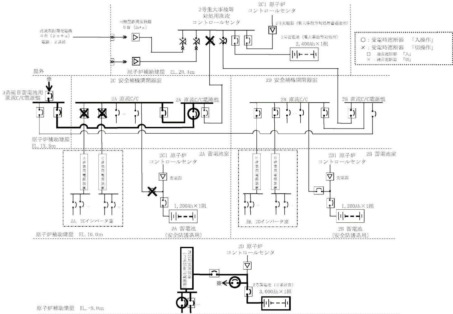
第 1.8-7 図 電源設備系統概要図 (5-1)
