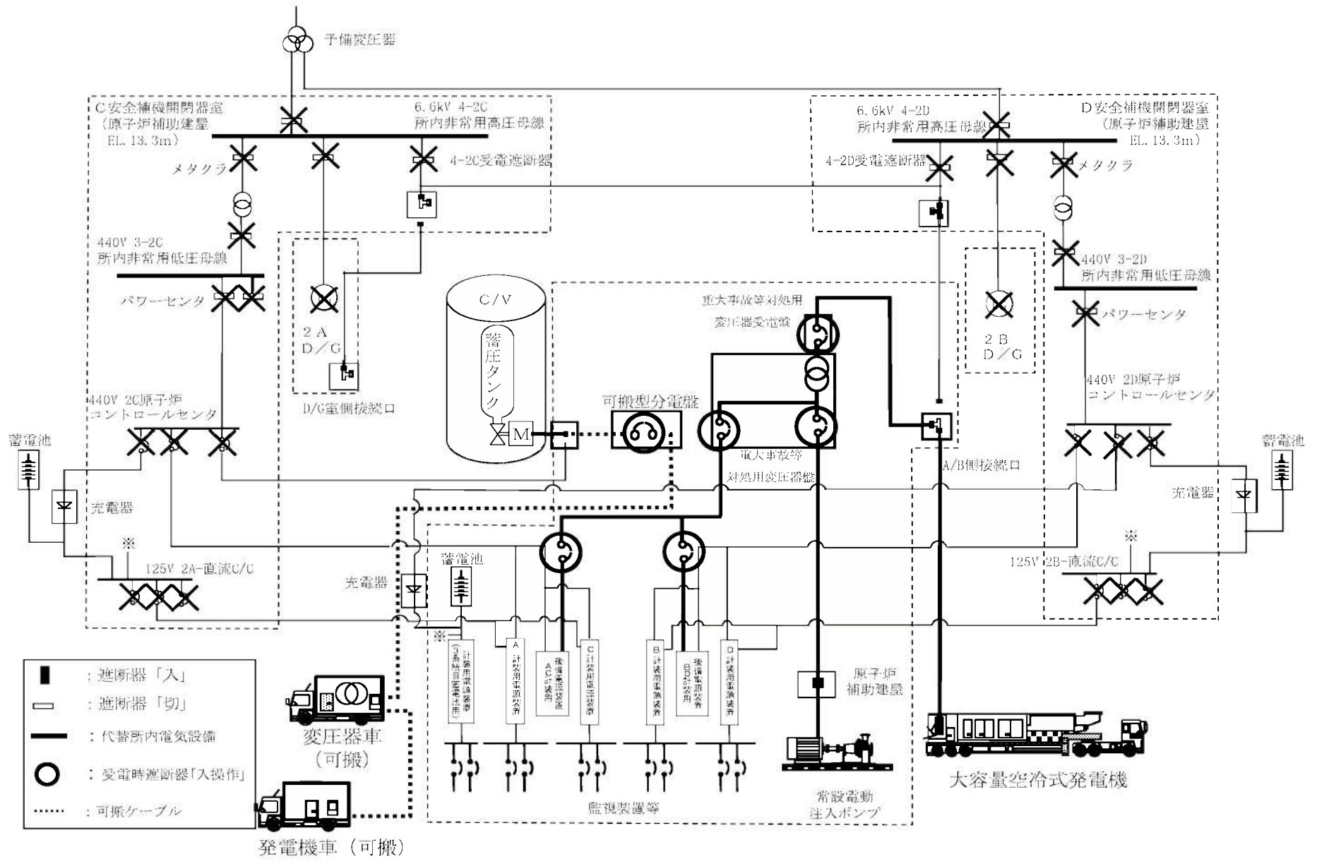
第1.8-8図 電源設備系統概要図(6)
