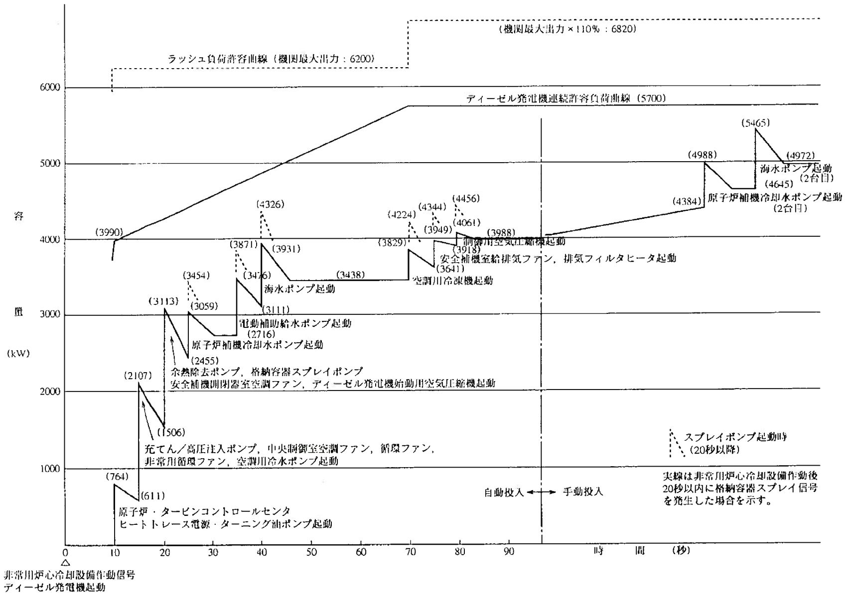
第1.8-11図 工学的安全施設作動時におけるディーゼル発電機の負荷曲線
