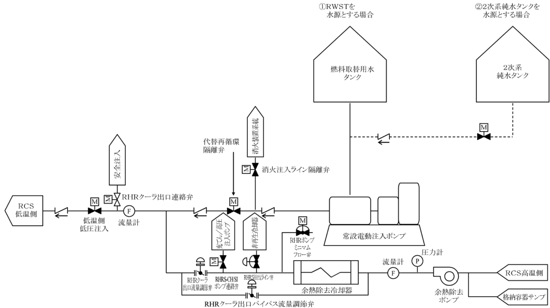
第3.1.4.2-34図 各影響緩和機能の系統概要図(津波:出力運転時炉心損傷、運転停止時炉心損傷) (13/25)
