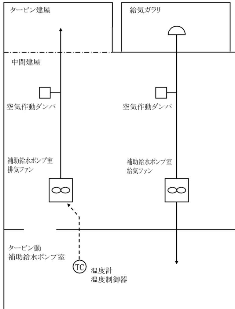
第3.1.4.2-34図 各影響緩和機能の系統概要図(津波:出力運転時炉心損傷) (21/25)
