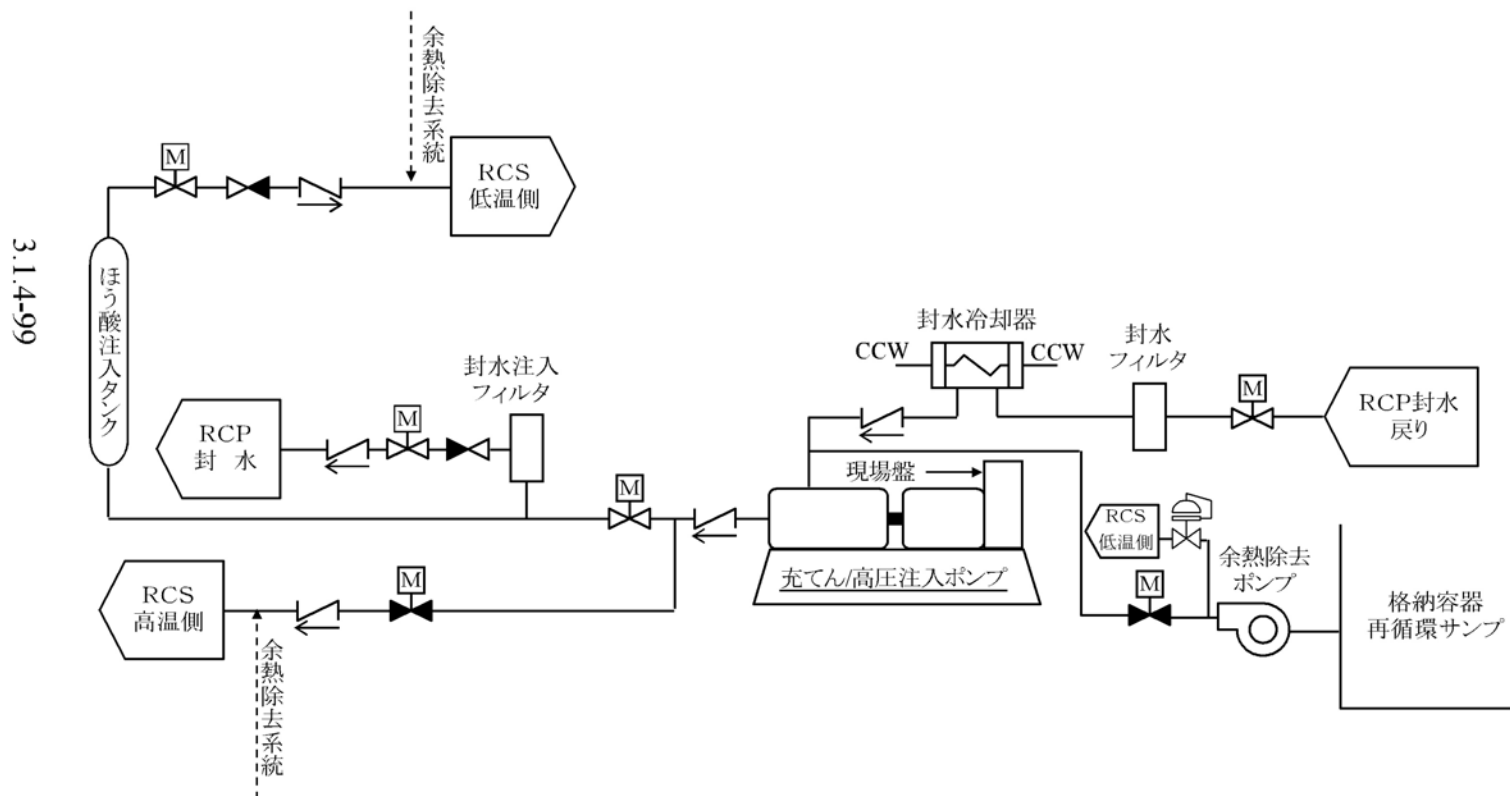
第3.1.4.2-14図 各影響緩和機能の系統概要図(地震:出力運転時炉心損傷)(20/34)
