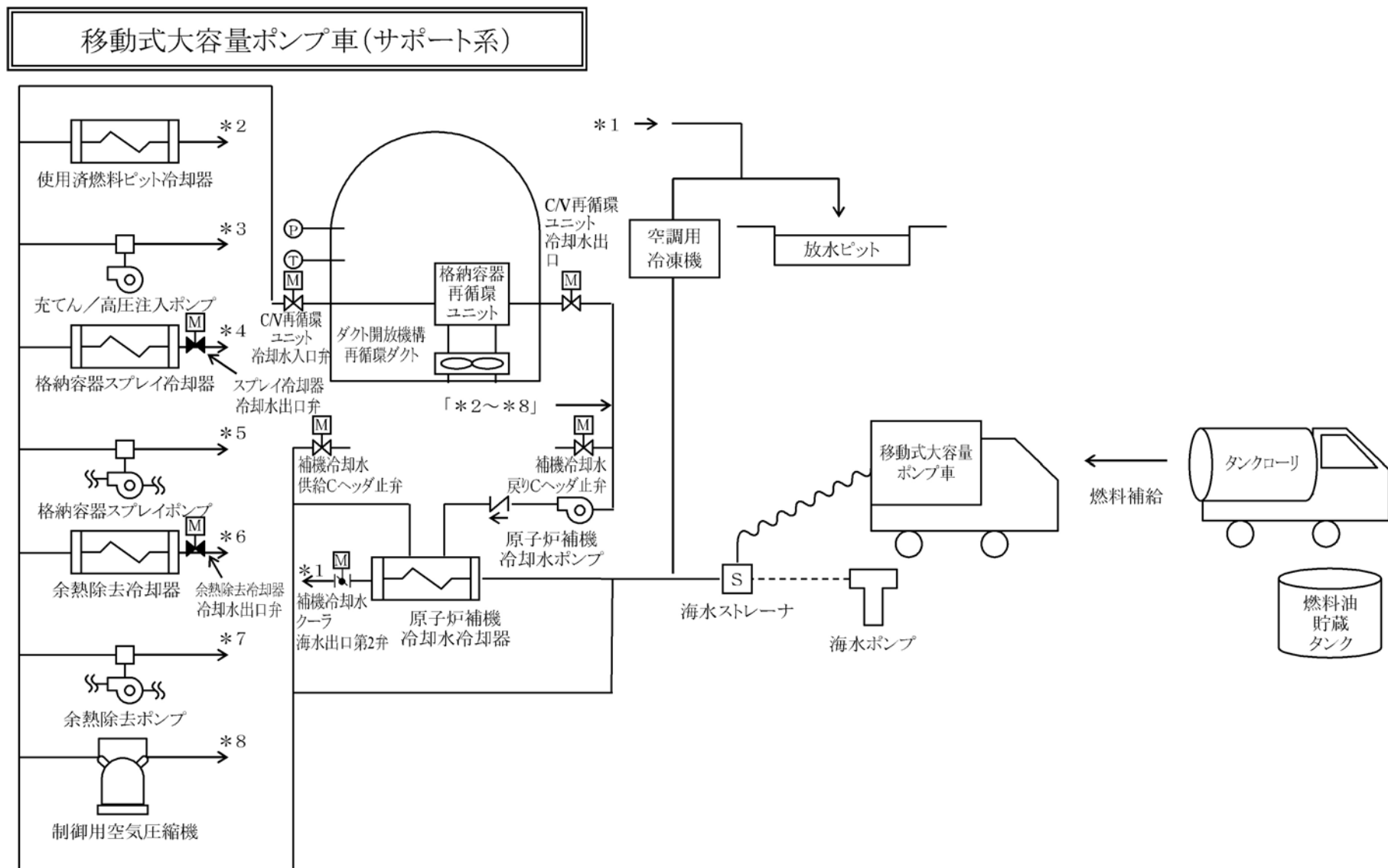
第3.1.4.2-34図 各影響緩和機能の系統概要図(津波:出力運転時炉心損傷、運転停止時炉心損傷、格納容器機能喪失) (20/25)
