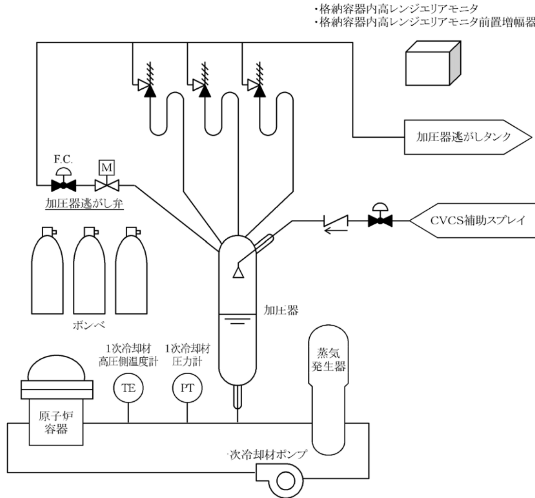
第3.1.4.2-14図 各影響緩和機能の系統概要図(地震:格納容器機能喪失)(15/34)
