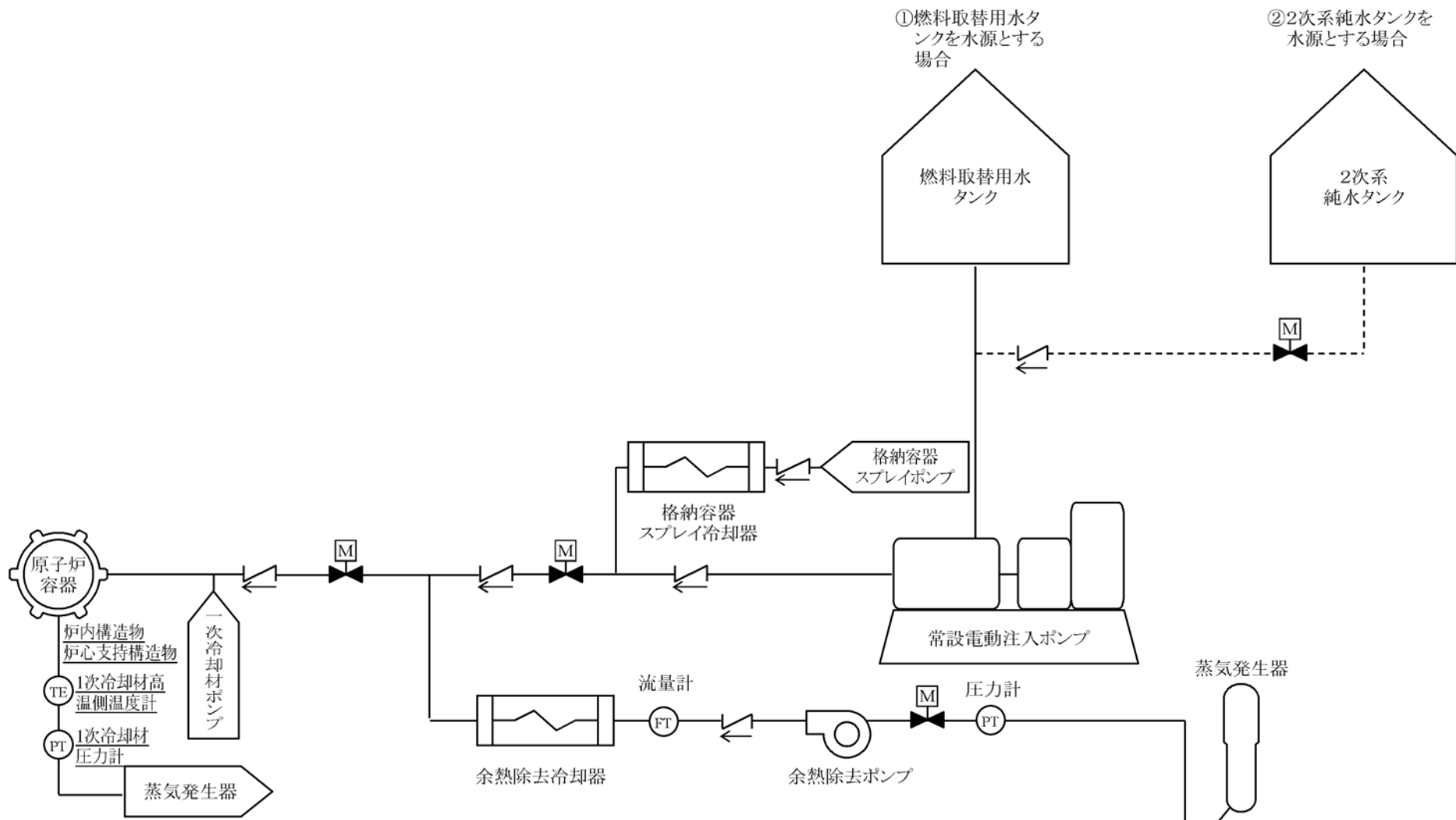
第3.1.4.2-14図 各影響緩和機能の系統概要図(地震:出力運転時炉心損傷、運転停止時炉心損傷)(8/34)
