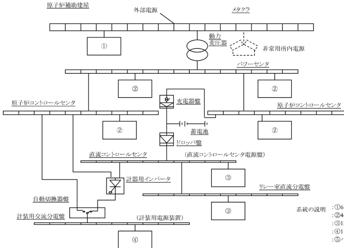
第3.1.4.2-14図 各影響緩和機能の系統概要図
