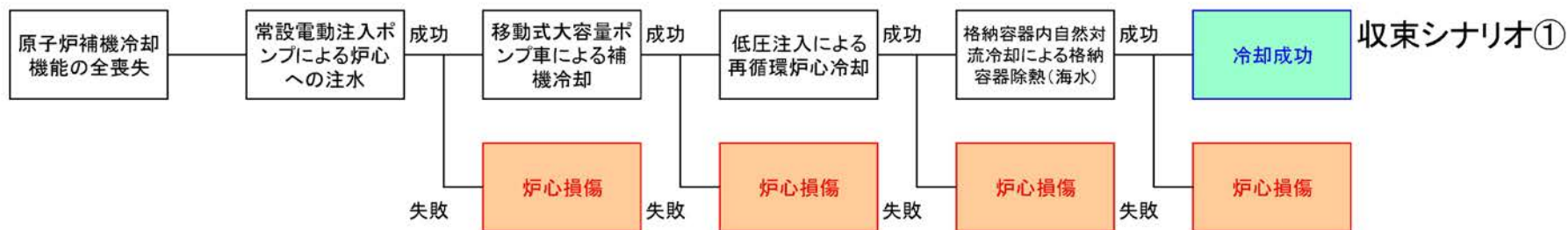
第 3.1.4.2-20 図 各起因事象における収束シナリオ(津波:運転停止時炉心損傷(区分 1))
