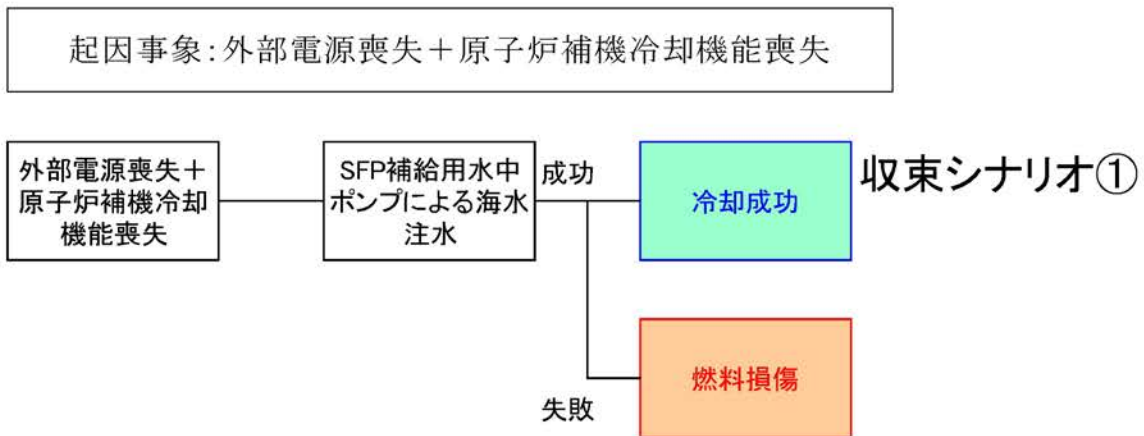
第 3.1.4.2-27 図 各起因事象における収束シナリオ (津波: SFP 燃料損傷 (区分 2))
