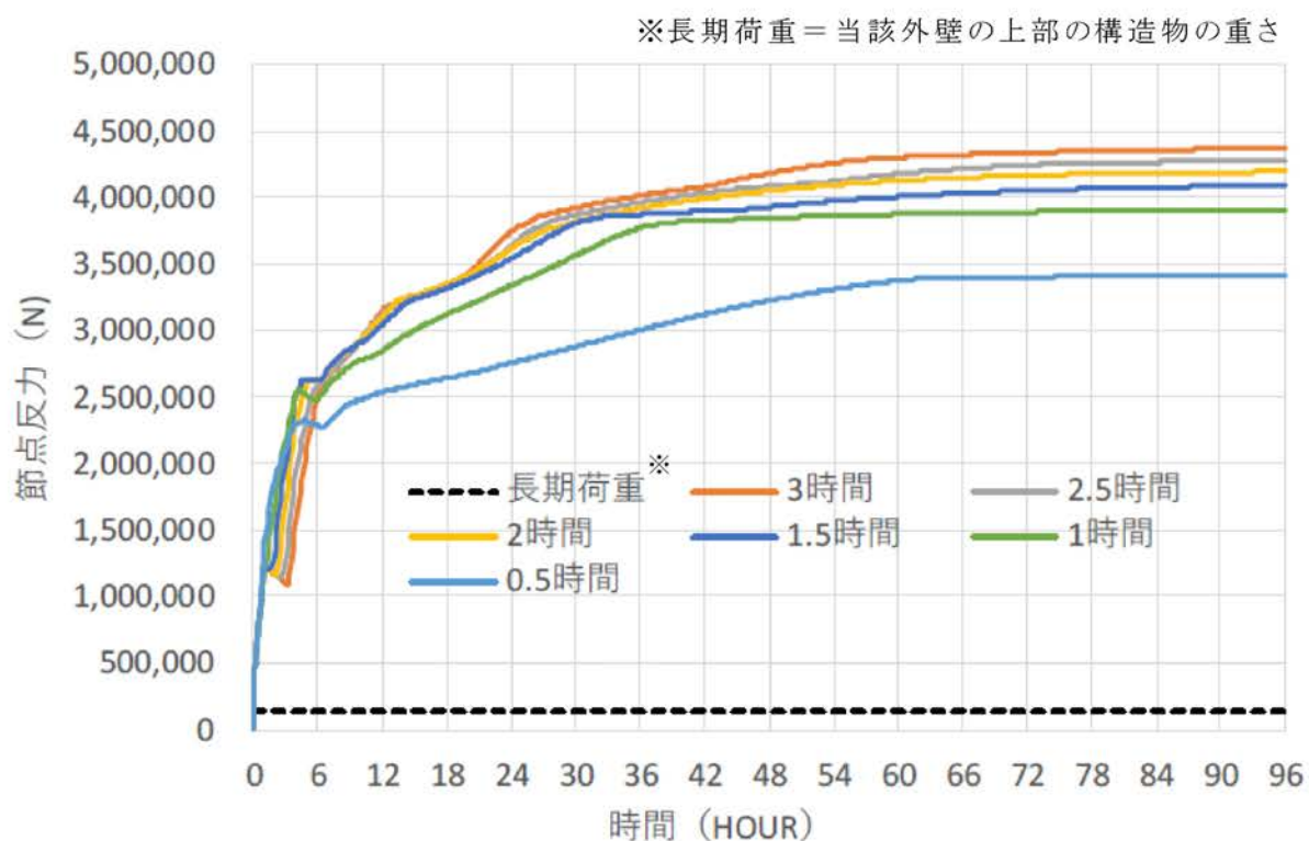
第 3.1.4.4-14 図 FEM 解析による火災影響評価結果 (節点反力経時変化)
