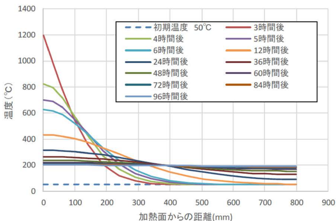
第 3.1.4.4-13 図 評価対象外壁における温度分布 (燃焼継続 3 時間)
