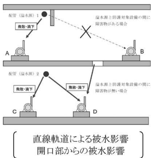
第 3.1.4.4-3 図 被水影響範囲の考え方
