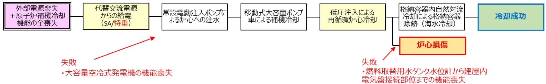
第 3.1.4.5-3 図 落雷評価における評価シナリオ (炉心 (停止時))
