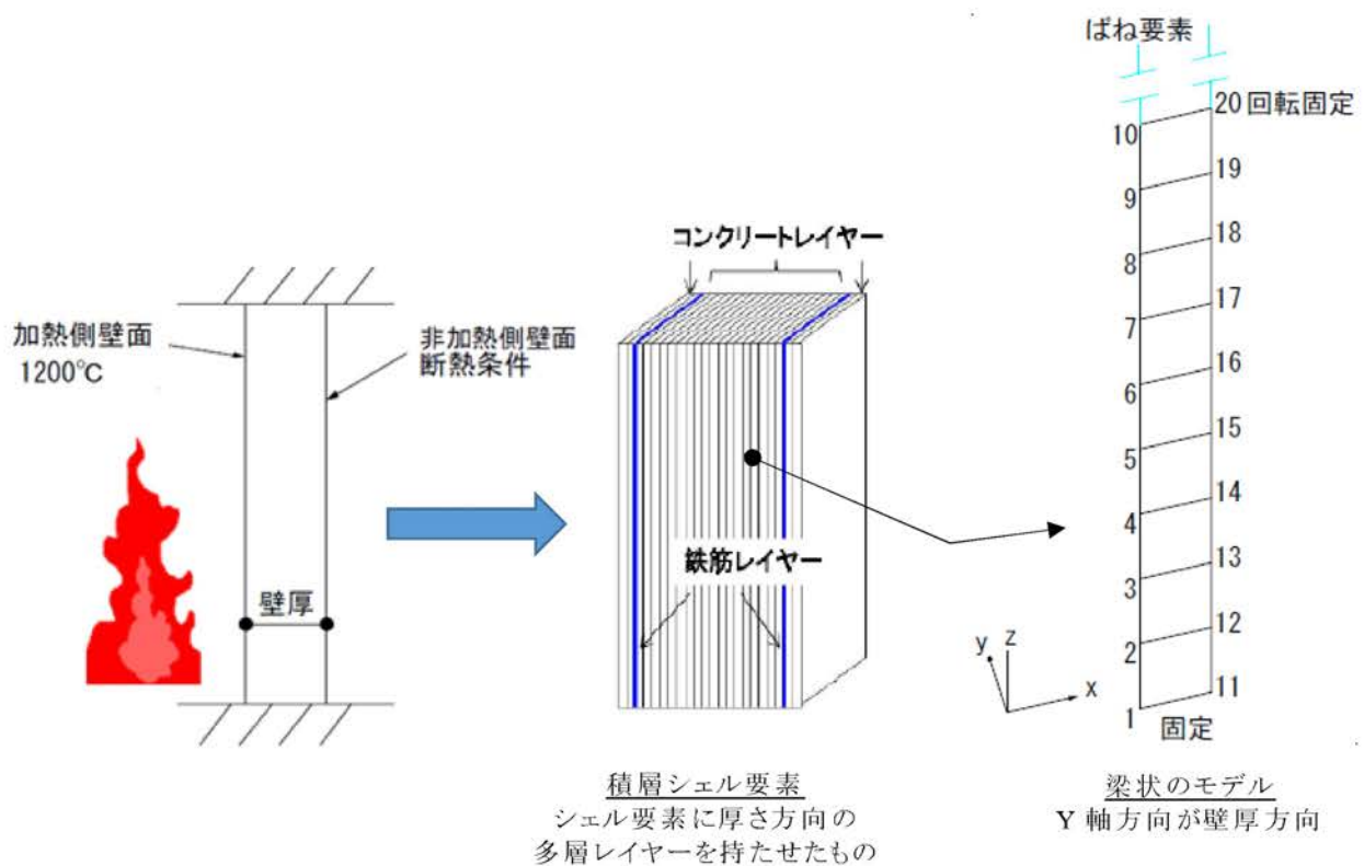
第 3.1.4.4-12 図 計算モデル(境界条件及び温度条件)
