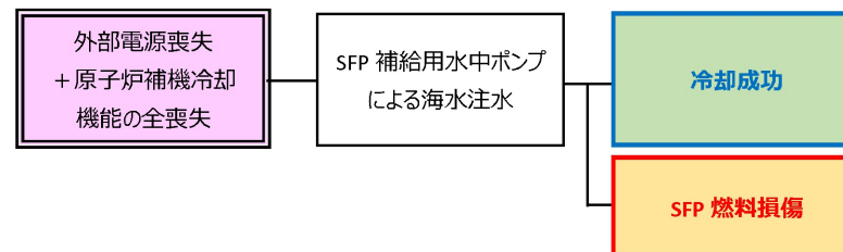
第 3.1.4.5-4 図 落雷評価における評価シナリオ (SFP)
