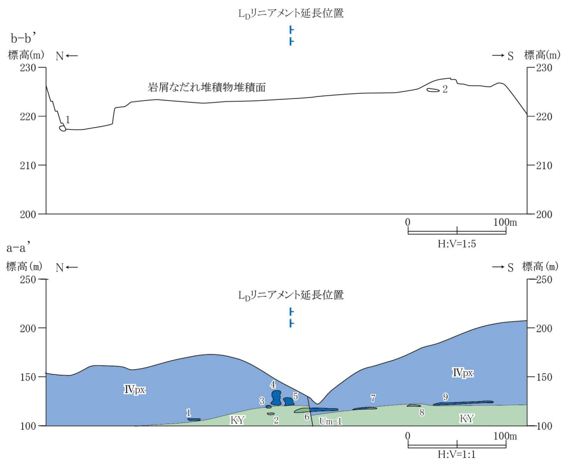
第 7. 3. 2. 24 図 ルートマップ及び地形・地質断面図(薩摩川内市八重付近)
