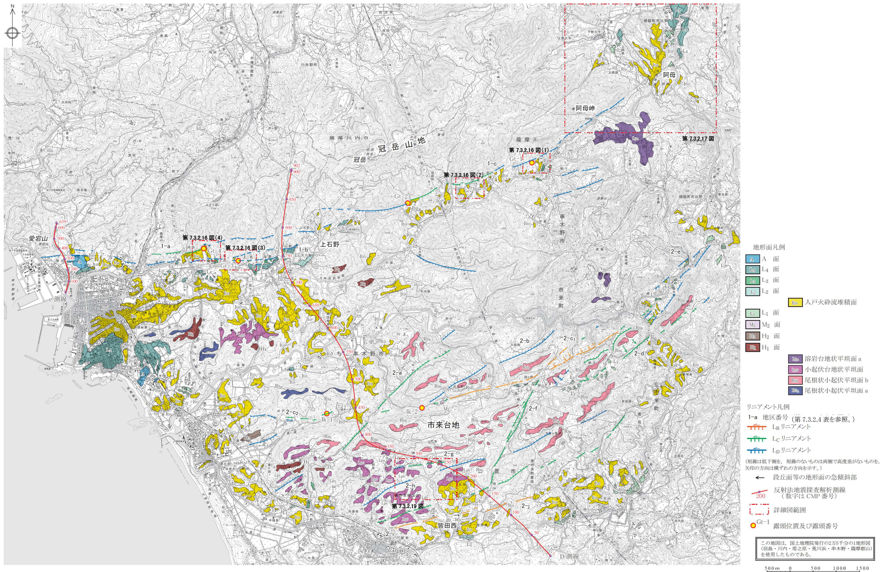
第 7.3.2.10 図 市来断層系周辺 (五反田川断層含む) の空中写真判読図
