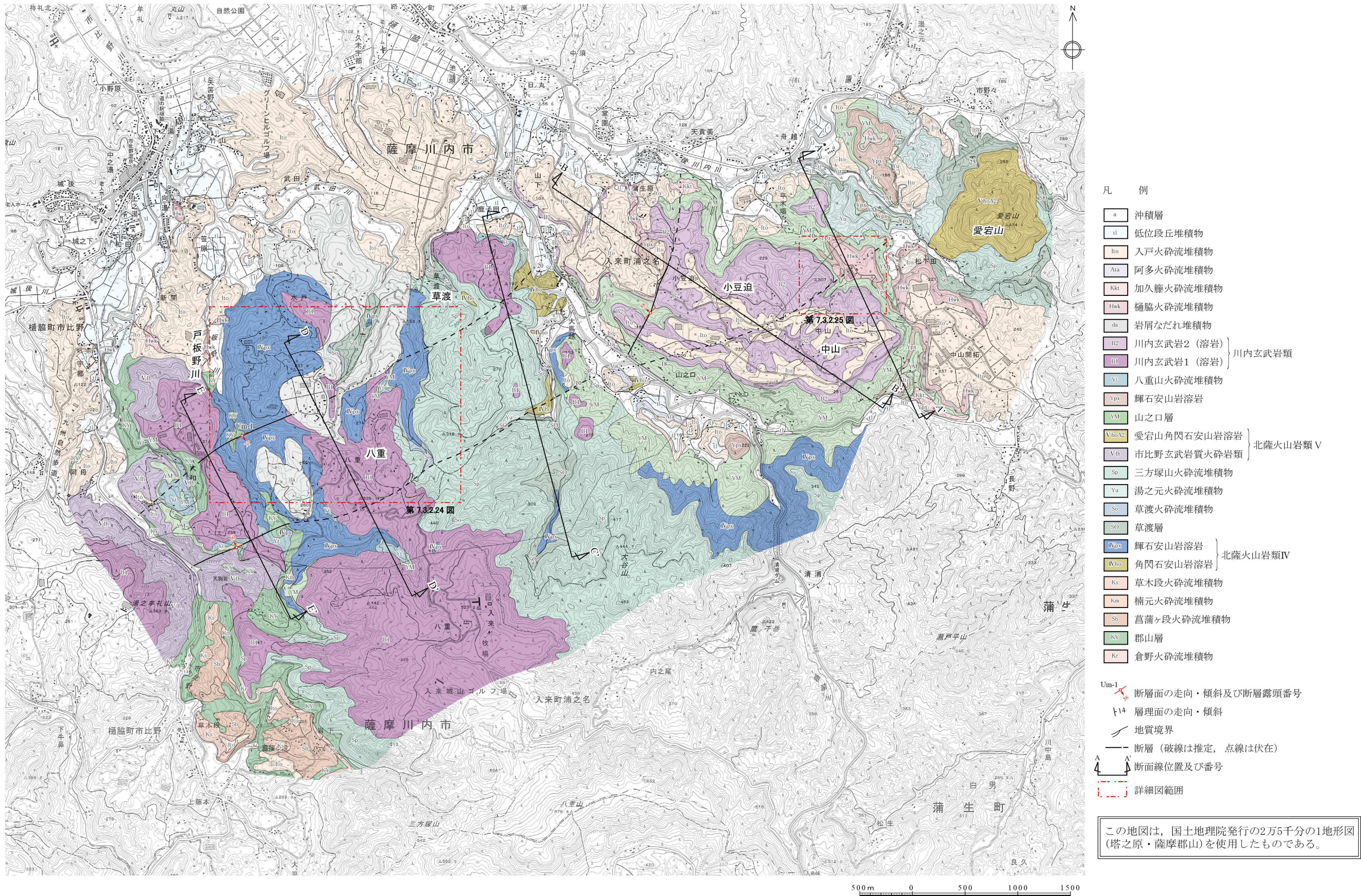
第 7.3.2.21 図 浦之名断層系周辺の地質図
