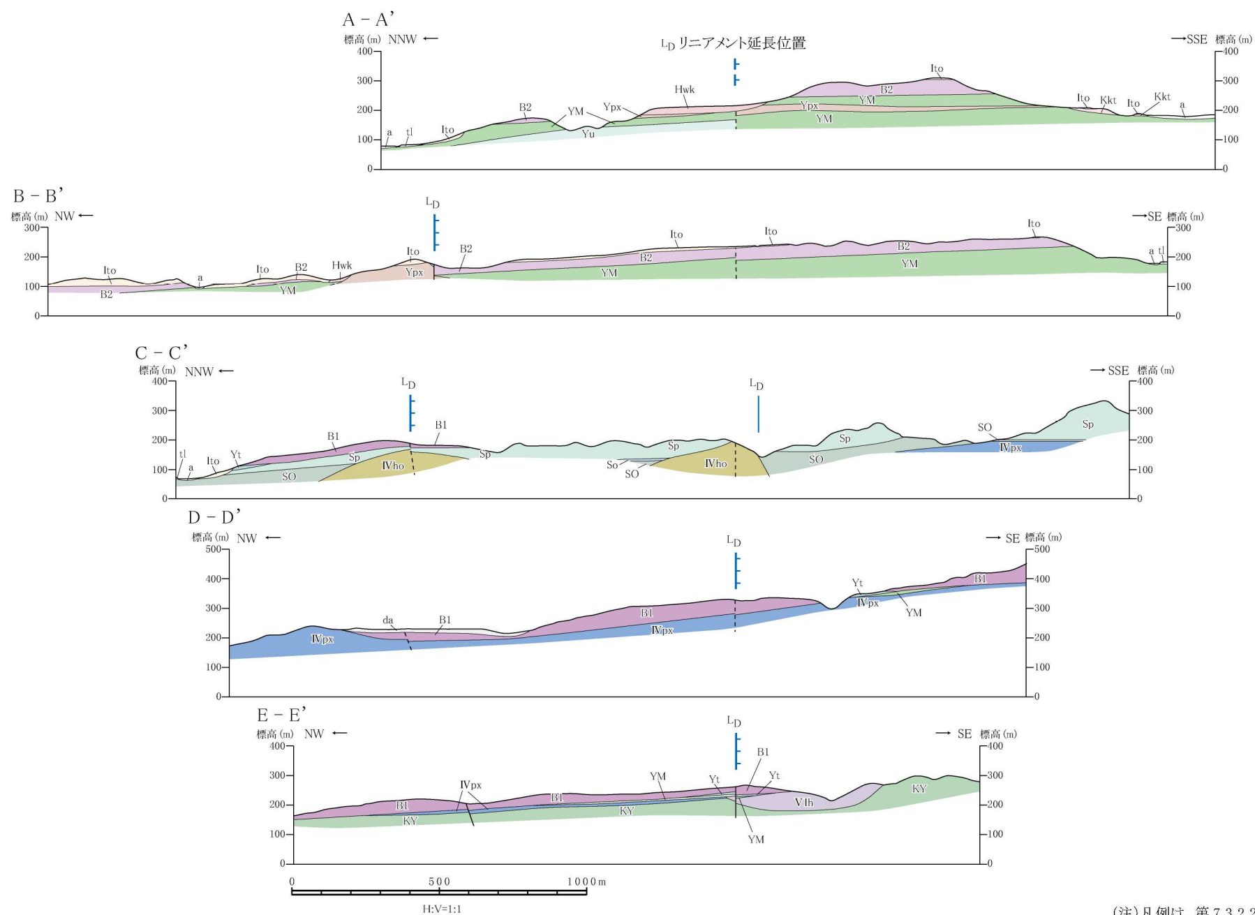
第 7.3.2.22 図 浦之名断層系周辺の地質断面図
