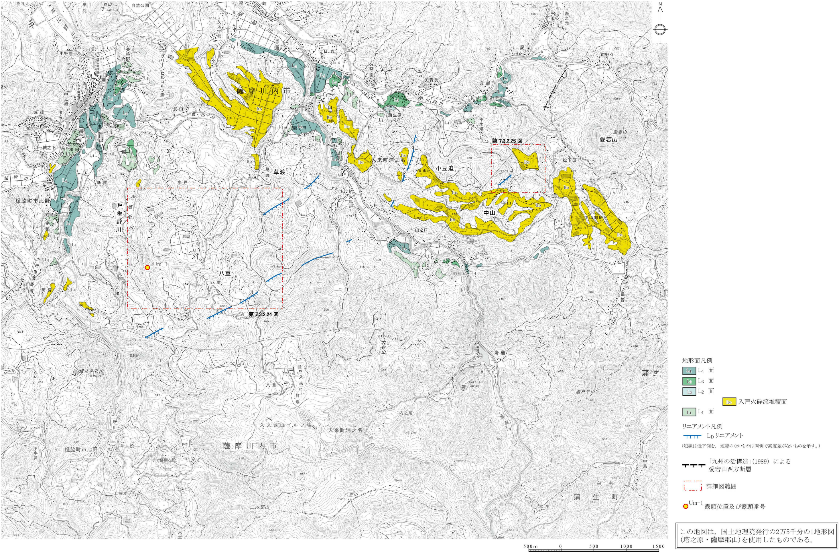
第 7.3.2.20 図 浦之名断層系周辺の空中写真判読図
