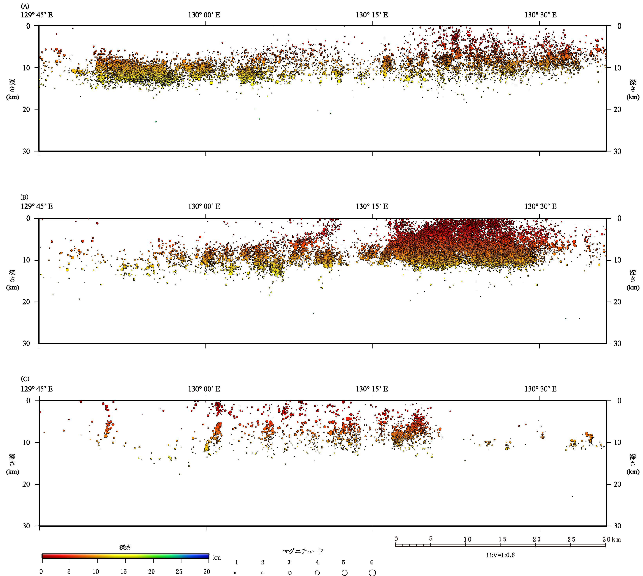
第 7.3.2.9 図(2) 敷地周辺の微小地震分布断面図
