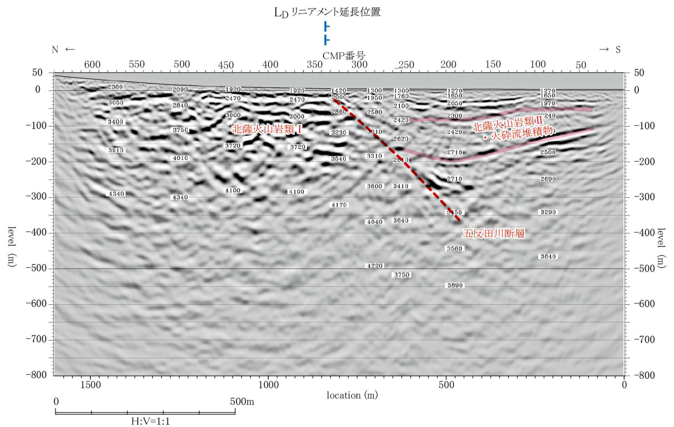
第 7.3.2.14 図(2) 反射法地震探査による深度断面とその解釈 (e 測線)
