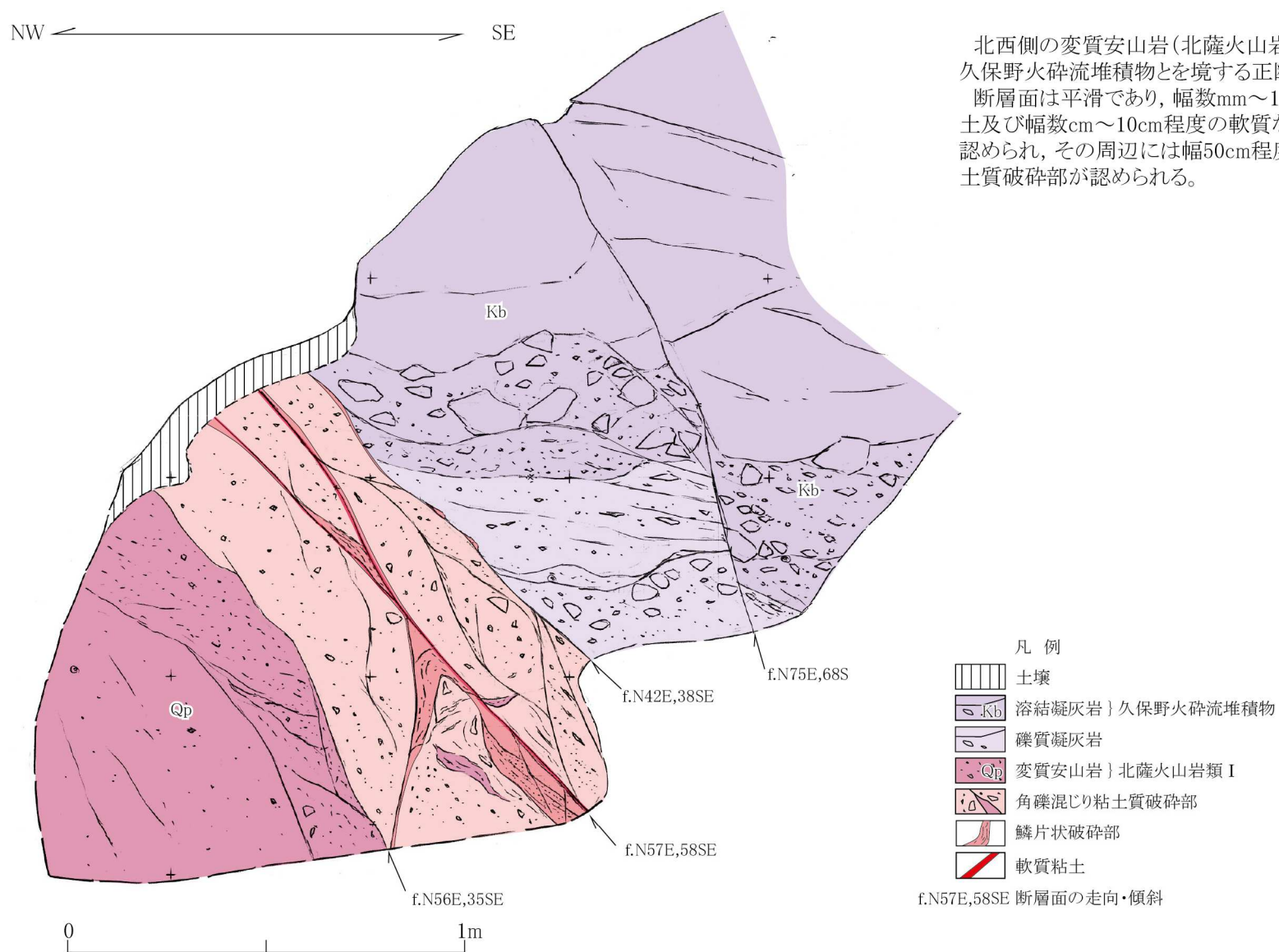
第 7. 3. 2. 15 図(2) 露頭スケッチ (Loc.Gt-2, いちき串木野市八牟礼)
