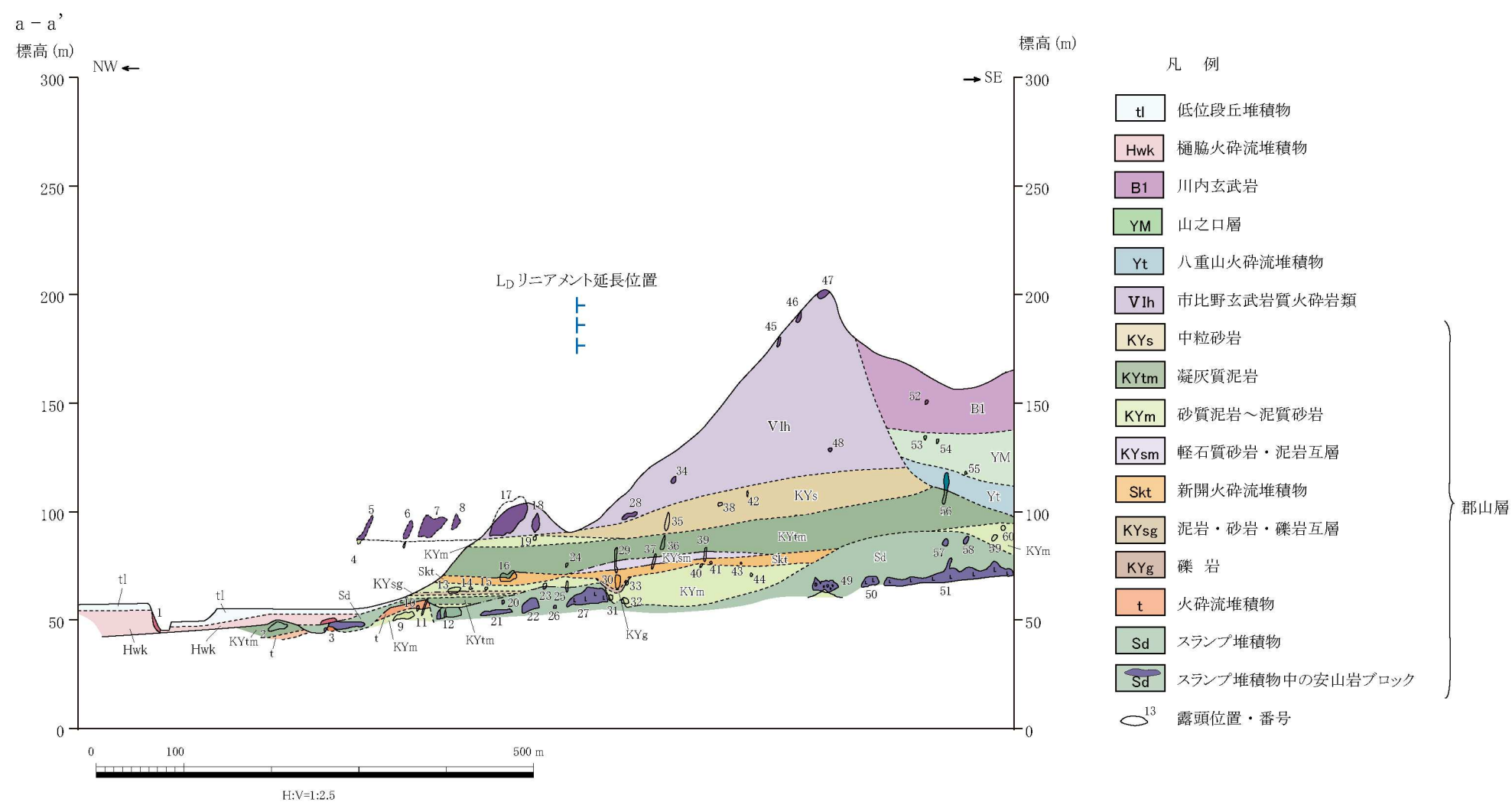
第 7.3.2.17 図 ルートマップ・地質断面図（薩摩川内市阿母付近）
