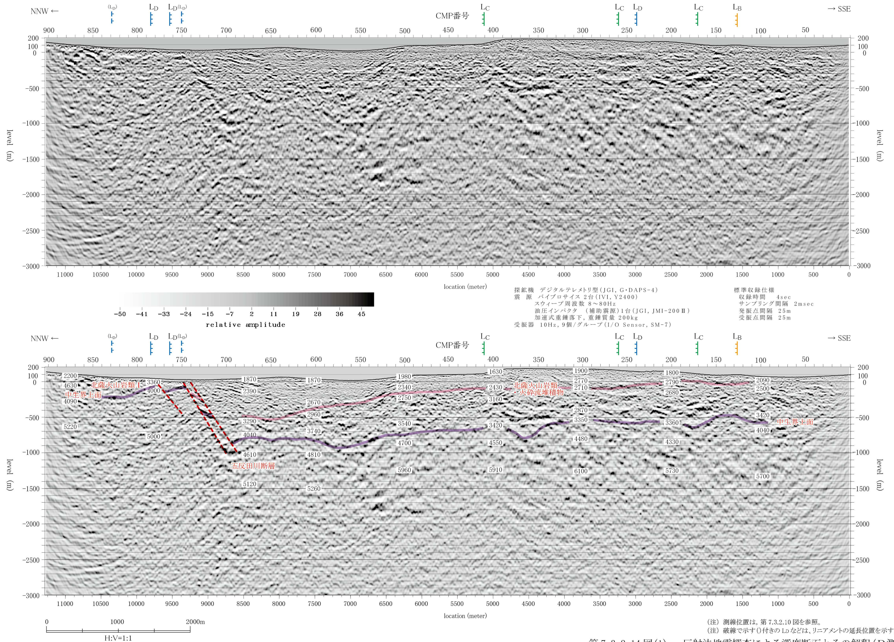
第 7.3.2.14 図(1) 反射法地震探査による深度断面とその解釈 (D測線)
