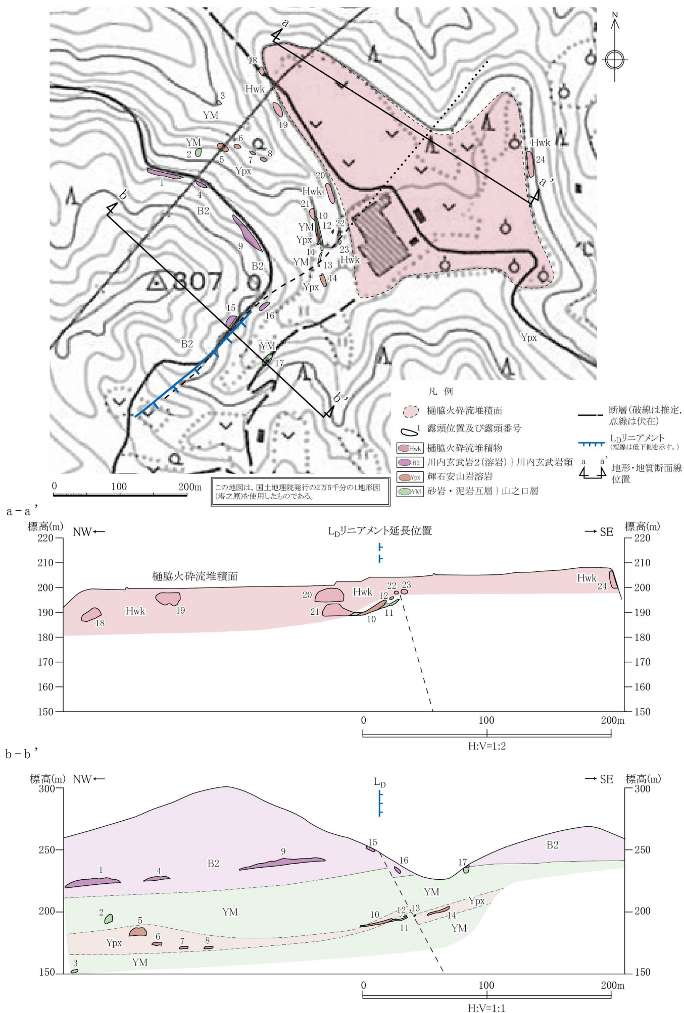
第 7.3.2.25 図 ルートマップ及び地形・地質断面図(薩摩川内市中山北方付近)
