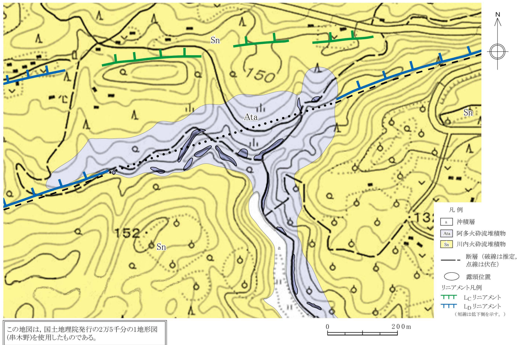
第 7.3.2.19 図 ルートマップ (日置市皆田西北方付近)
