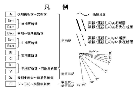
第7.3.2.99図 (2) F-A断層の音波探査記録断面図 (No.17m測線)
