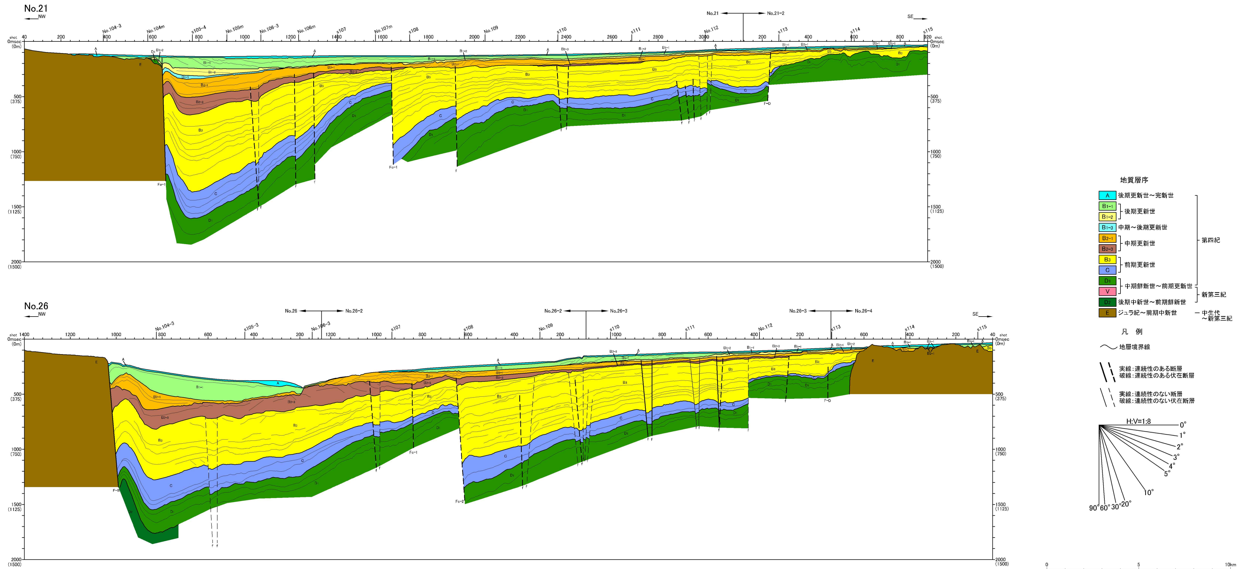
第7.3.2.94図 (2) 敷地前面海域の海底地質断面図 (その2)
