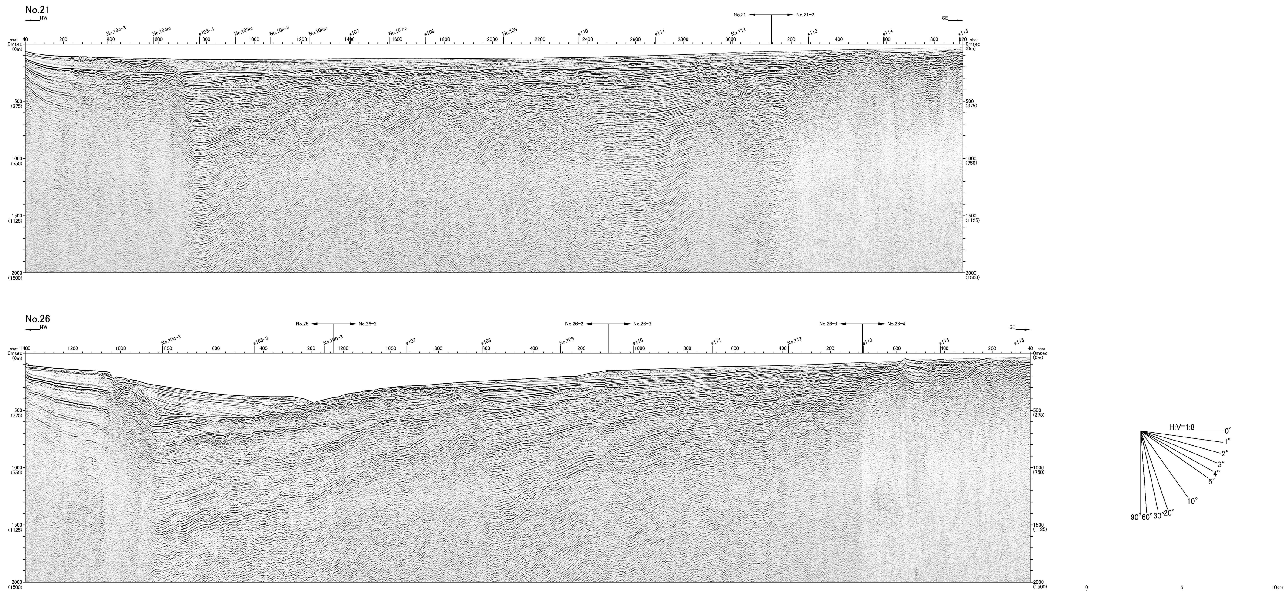
第7.3.2.95図 (2) 敷地前面海域の反射断面図 (その2) 6-7-3-284
