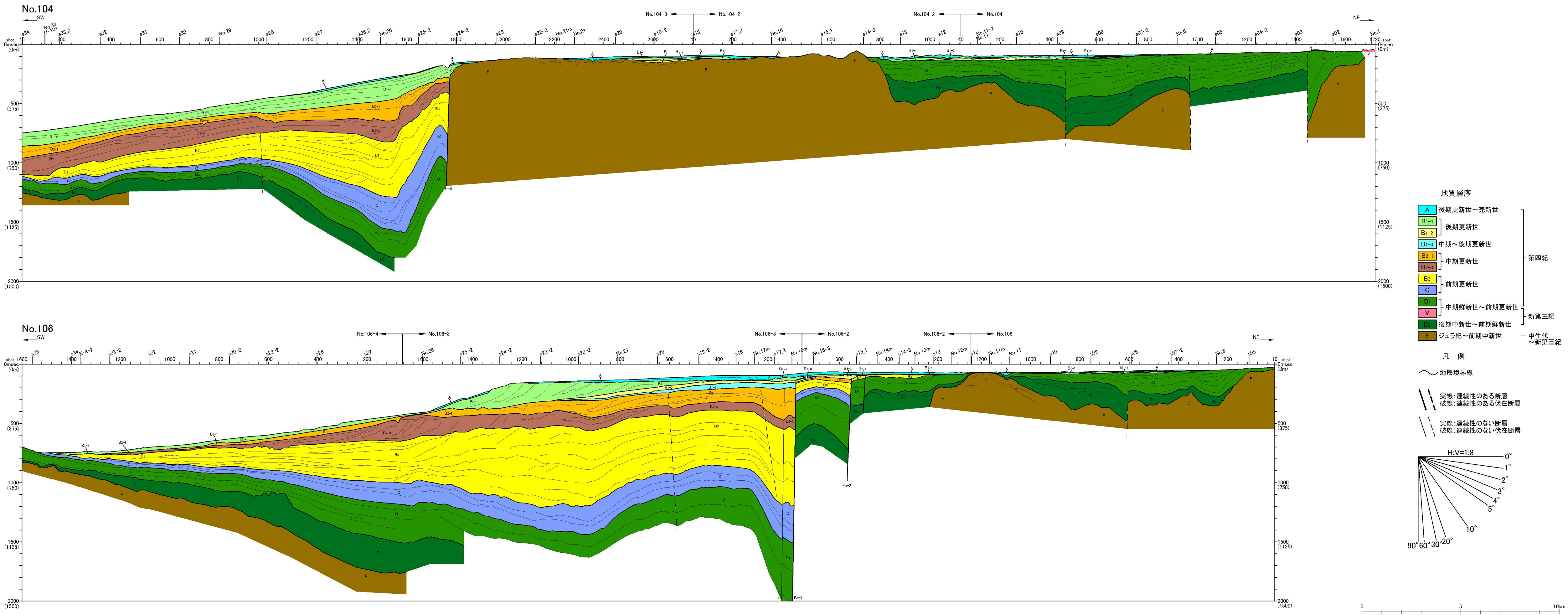
第7.3.2.94図 (3) 敷地前面海域の海底地質断面図 (その3)
