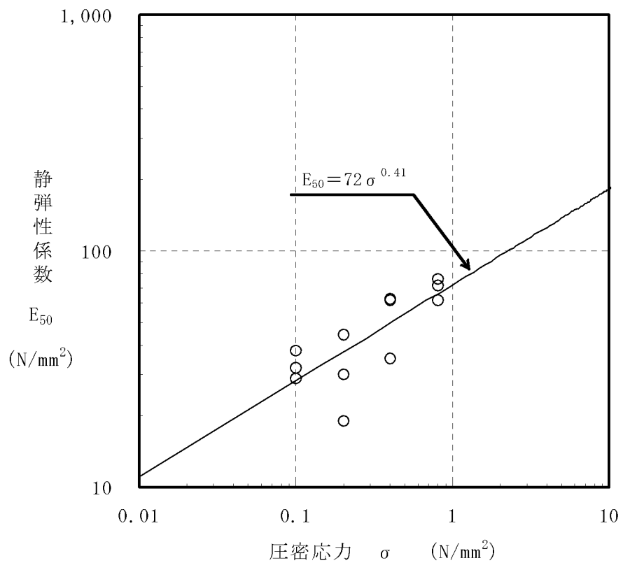
第 7.3.5.19 図 三軸圧縮試験結果（粘板岩 D 級）（静的変形特性）
