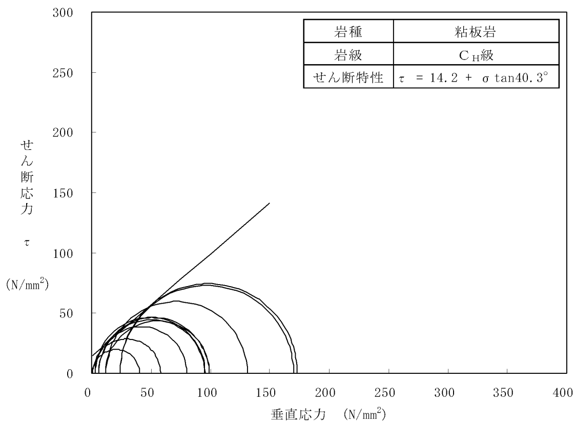
第 7.3.5.15 図 (3) 三軸圧縮試験結果 (粘板岩 C H 級)
