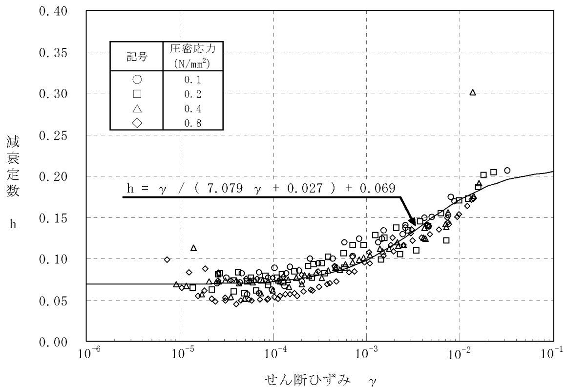
第 7.3.5.23 図 繰返し三軸試験結果（粘板岩 D 級）（減衰特性）
