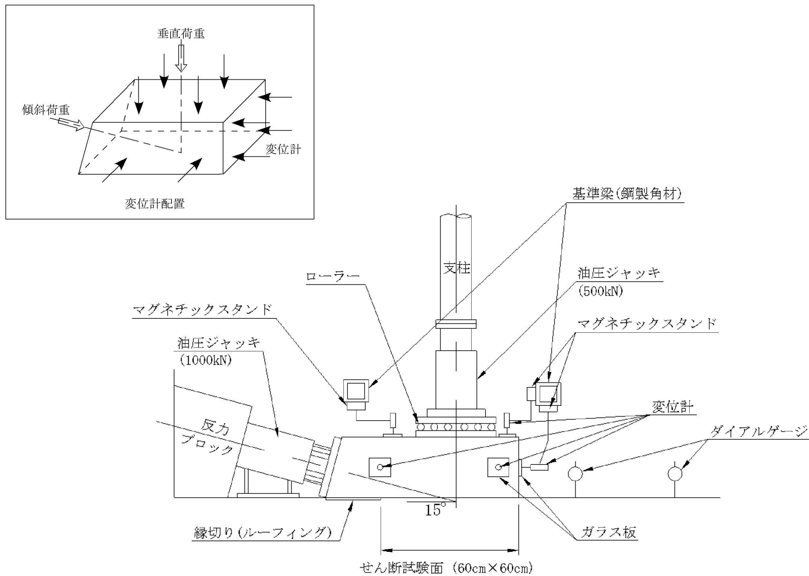
第 7.3.5.4 図 (2) ブロックせん断試験装置概略図 (ST-2 及び ST-4)
