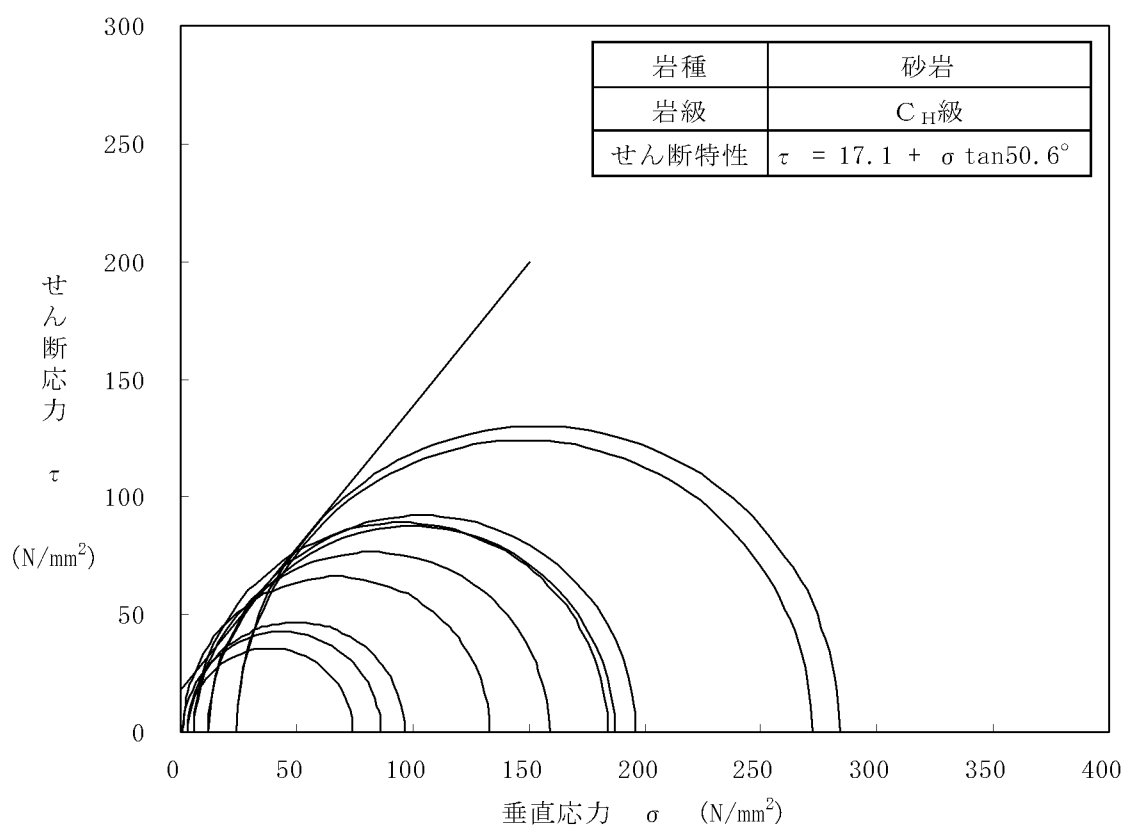
第 7.3.5.15 図 (2) 三軸圧縮試験結果 (砂岩 C H 級)
