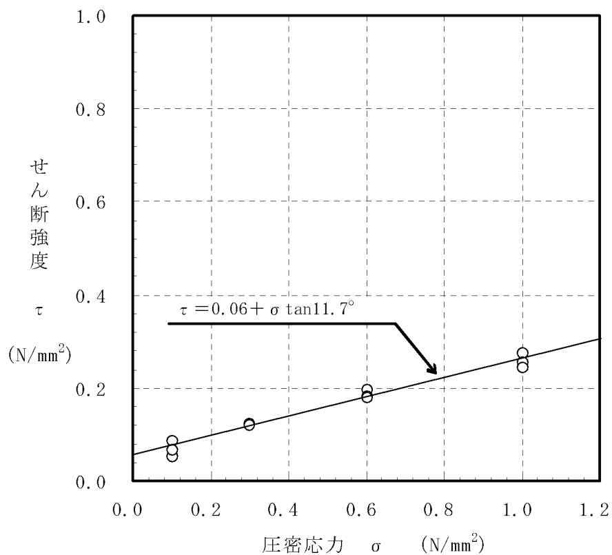
第 7.3.5.20 図 三軸圧縮試験結果（断層内物質（凝灰質粘土状）） （強度特性）
