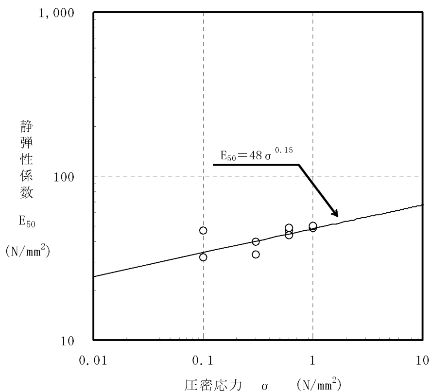
第 7.3.5.21 図 三軸圧縮試験結果（断層内物質（凝灰質粘土状）） （静的変形特性）
