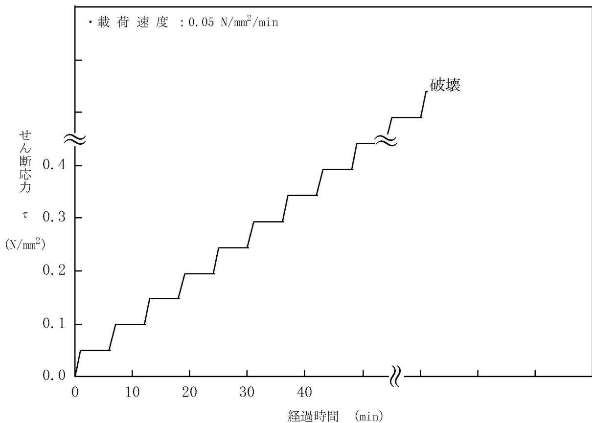
第 7.3.5.5 図 (2) ブロックせん断試験載荷パターン (ST-2 及び ST-4)
