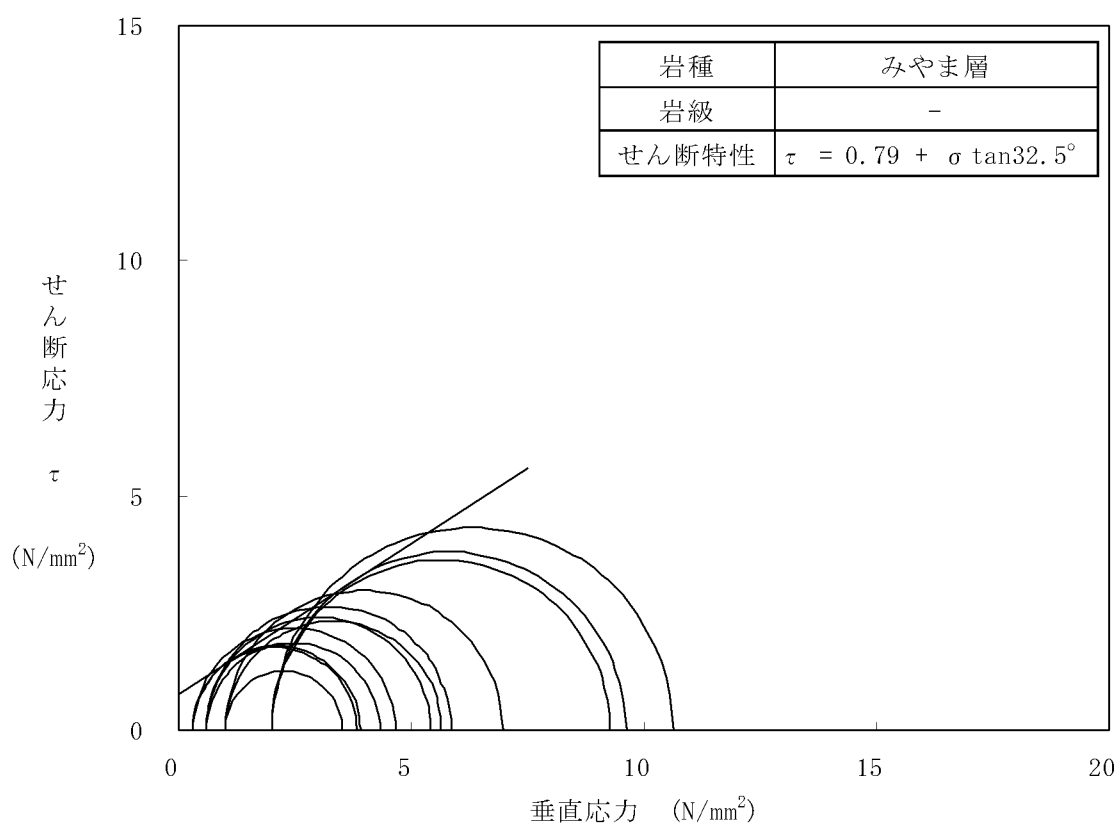
第 7.3.5.15 図 (4) 三軸圧縮試験結果 (みやま層)
