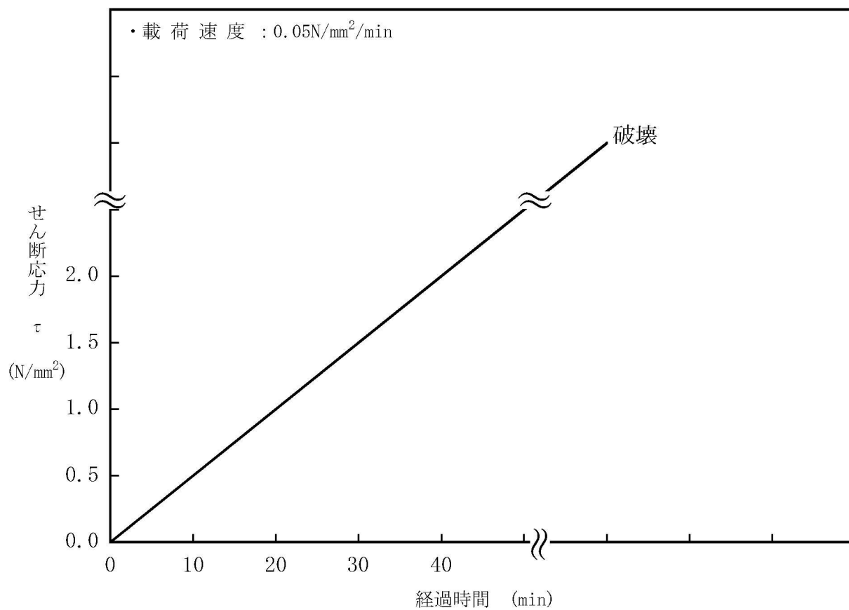
第 7.3.5.5 図 (1) ブロックせん断試験載荷パターン (地上部)
