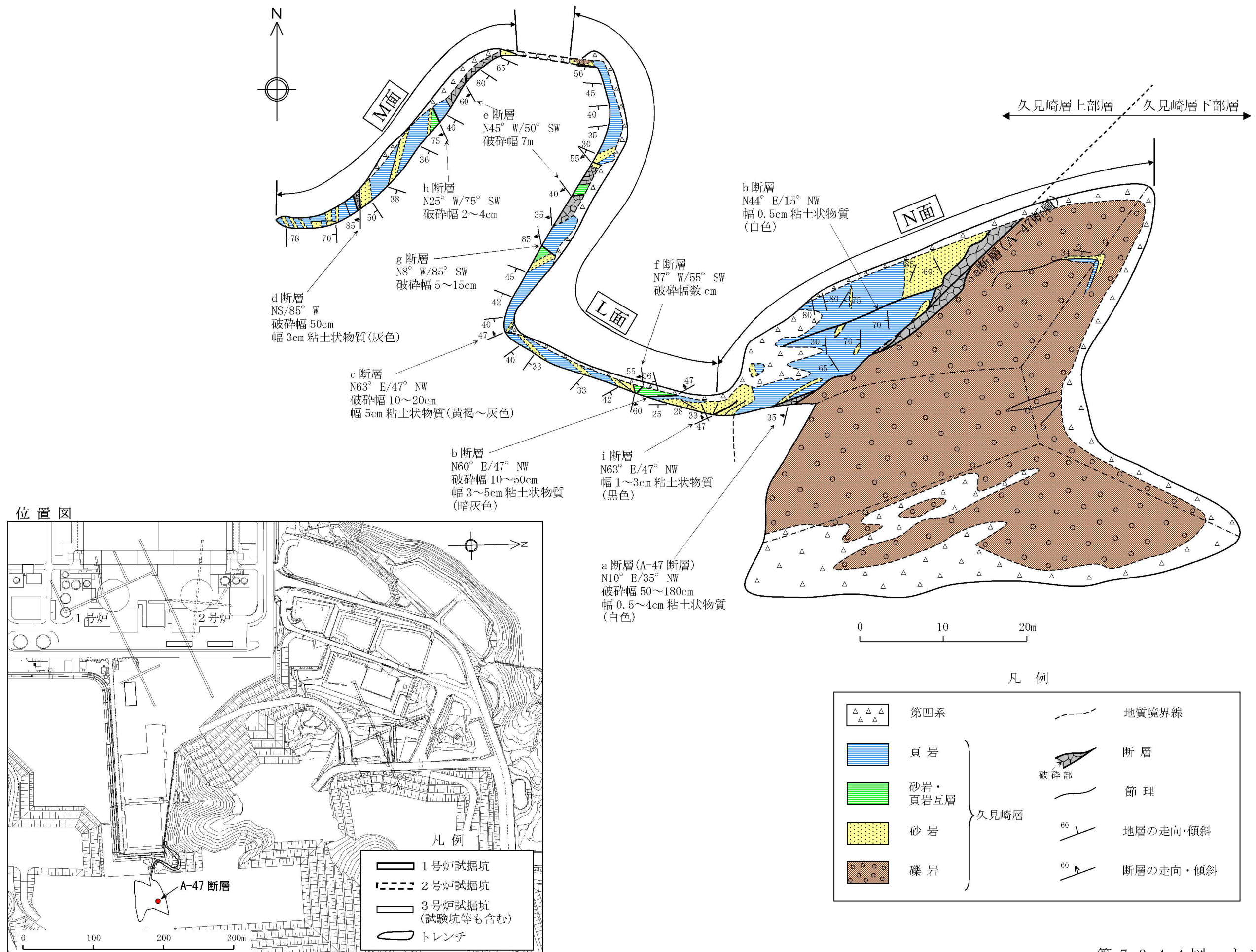
第 7.3.4.4 図 トレンチ平面図
