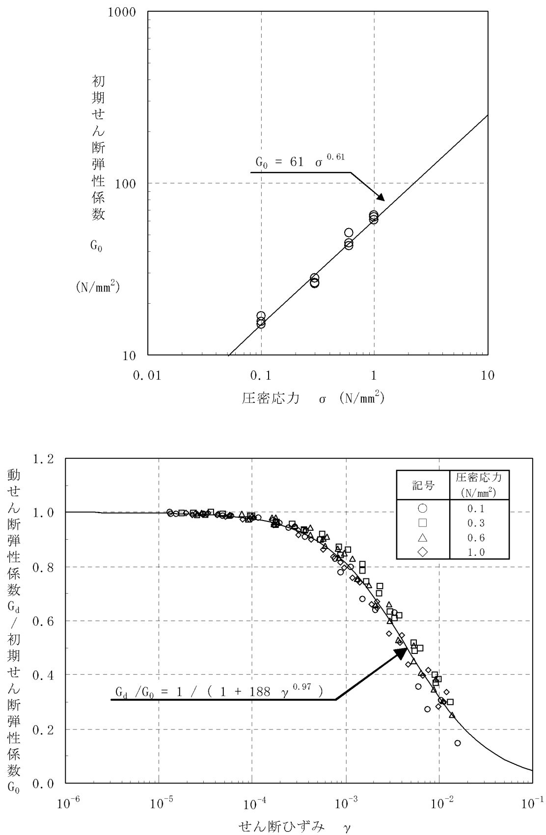
第 7.3.5.24 図 繰返し三軸試験結果（断層内物質（凝灰質粘土状）） （動の変形特性）
