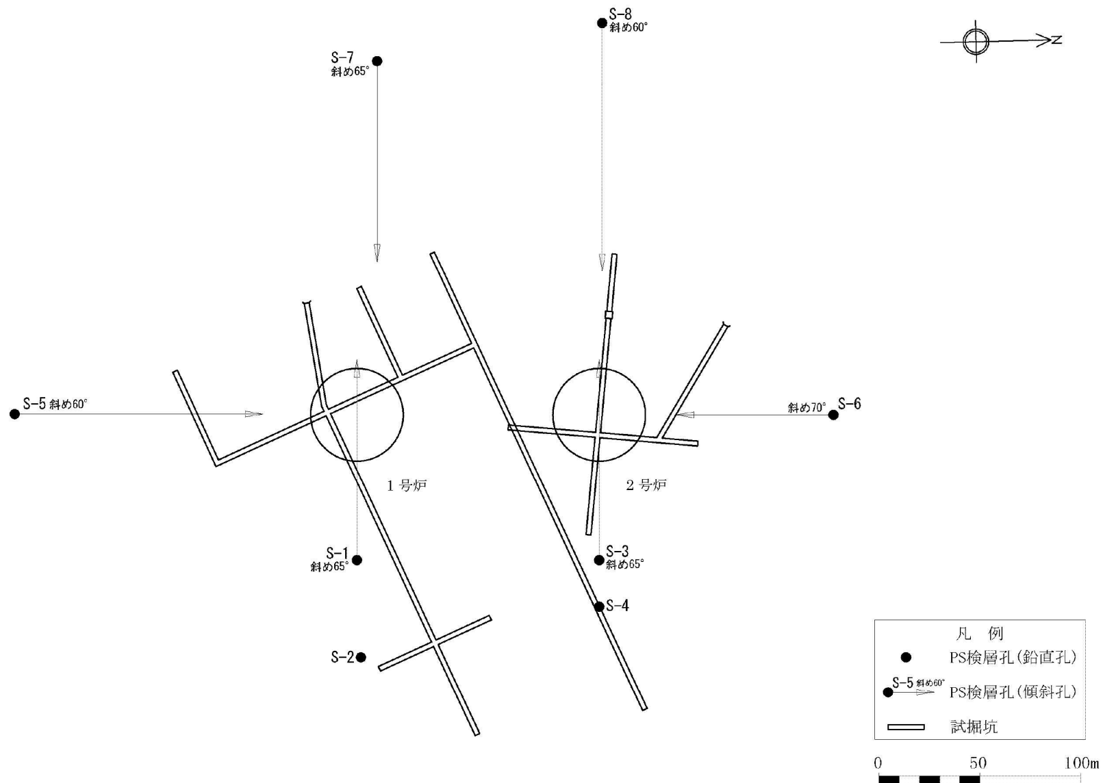
第 7.3.5.6 図 P S 検層位置図
