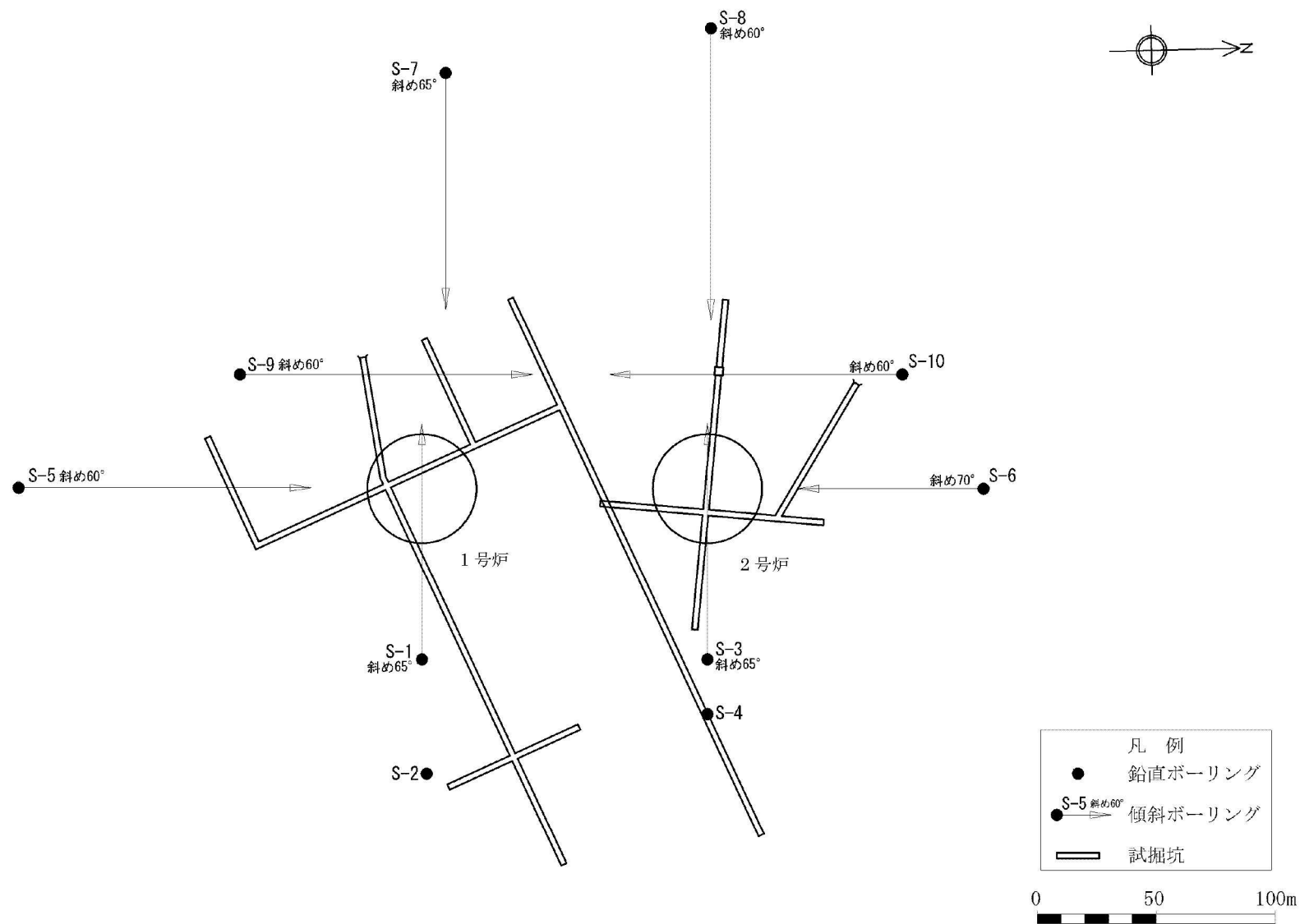
第 7.3.5.2 図 岩石試験試料採取位置図
