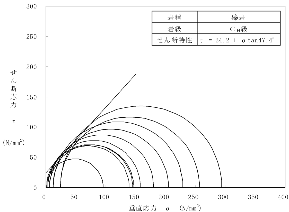
第 7.3.5.15 図 (1) 三軸圧縮試験結果 (礫岩 C H 級)
