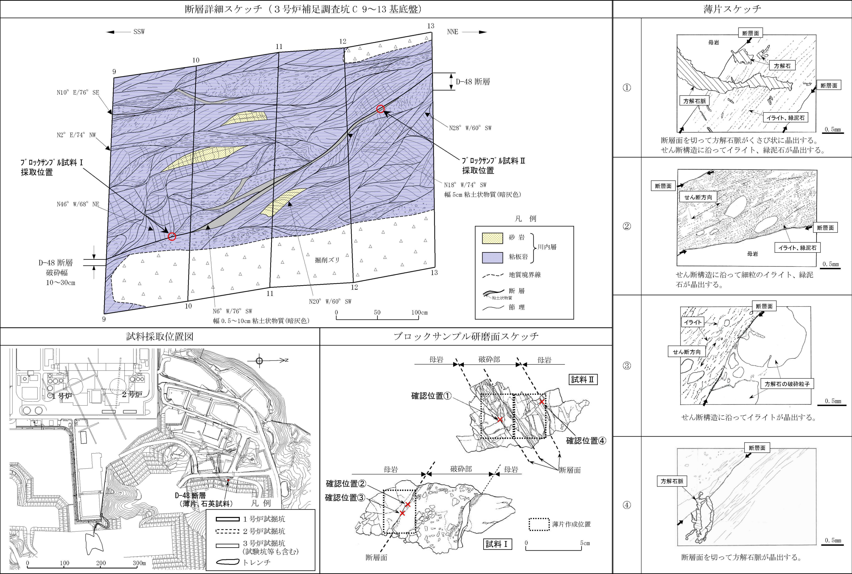
第 7. 3. 4. 6 図 (3) 断層詳細スケッチ・薄片観察結果（D－48 断層） 6－7－3－368
