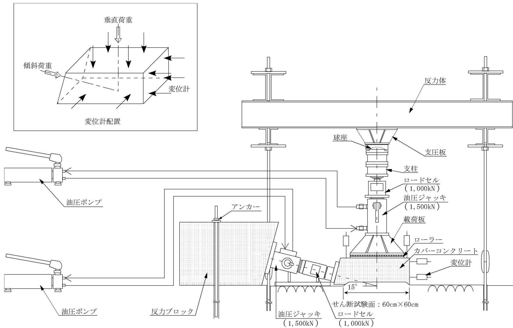
第 7.3.5.4 図 (1) ブロックせん断試験装置概略図 (地上部)
