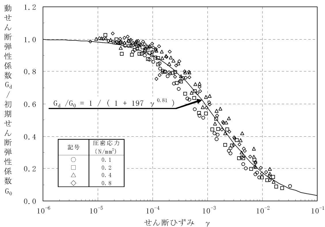
第 7.3.5.22 図 繰返し三軸試験結果（粘板岩 D 級）（動的変形特性）
