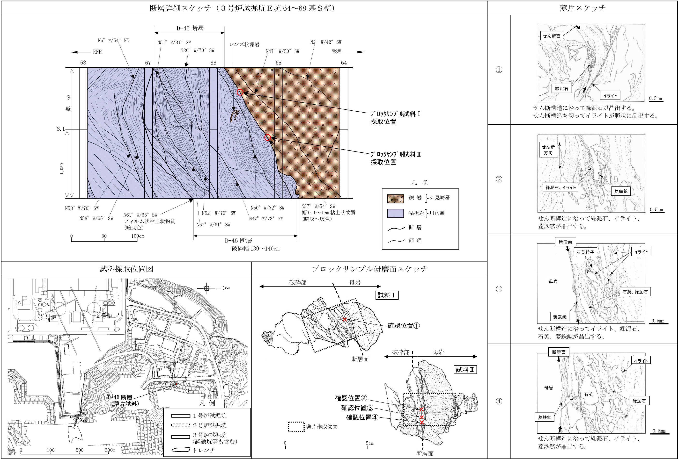
第 7. 3. 4. 6 図(2) 断層詳細スケッチ・薄片観察結果（D－46断層） 6－7－3－367
