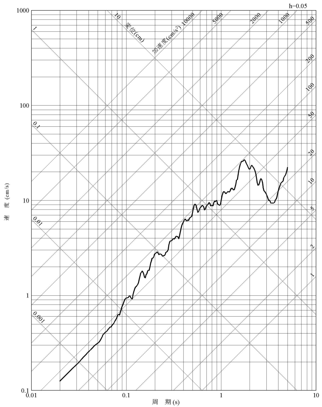
第 7.5.7.5 図 琉球海溝におけるプレート間地震 ( M_w 9.1 ) の応答スペクトル (鉛直方向)
