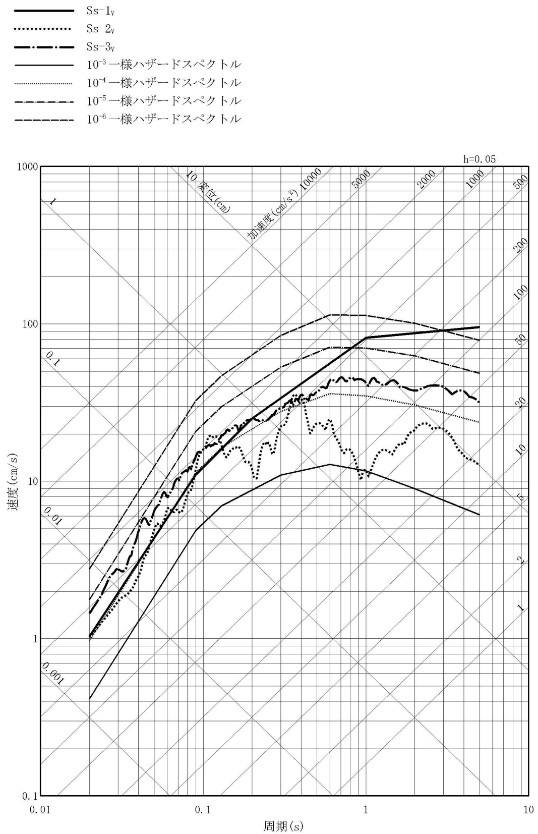
第 7. 5. 6. 70 図 基準地震動の応答スペクトル及び解放基盤表面における地震動の一様ハザードスペクトル (鉛直方向)
