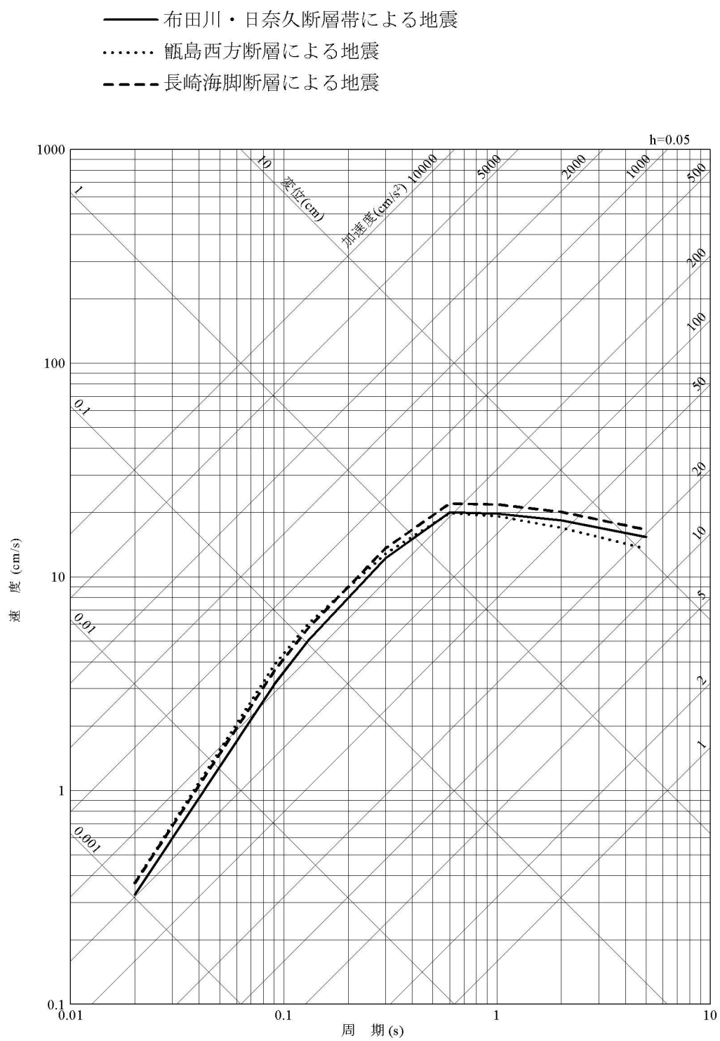
第 7.5.7.1 図 長大な活断層による地震の応答スペクトル (水平方向)
