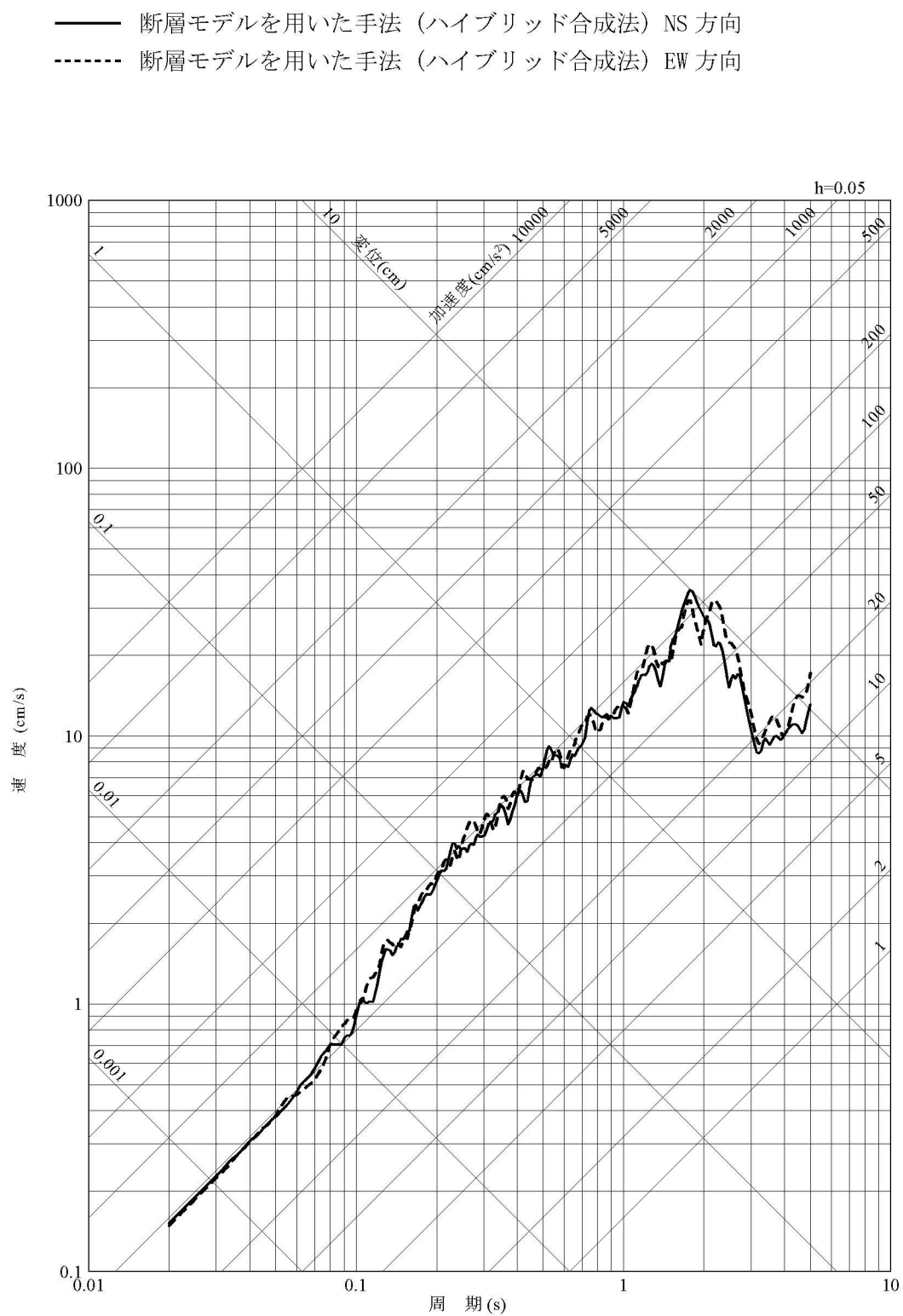
第 7.5.7.4 図 琉球海溝におけるプレート間地震 ( M_w 9.1 ) の応答スペクトル (水平方向)
