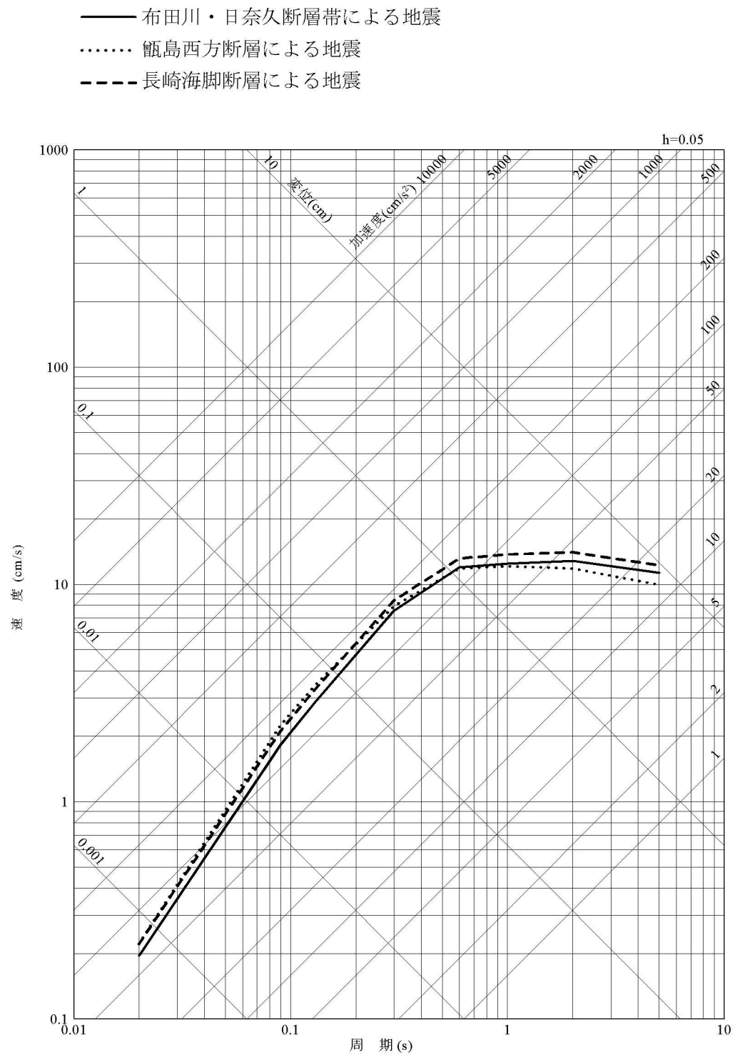
第 7.5.7.2 図 長大な活断層による地震の応答スペクトル (鉛直方向)
