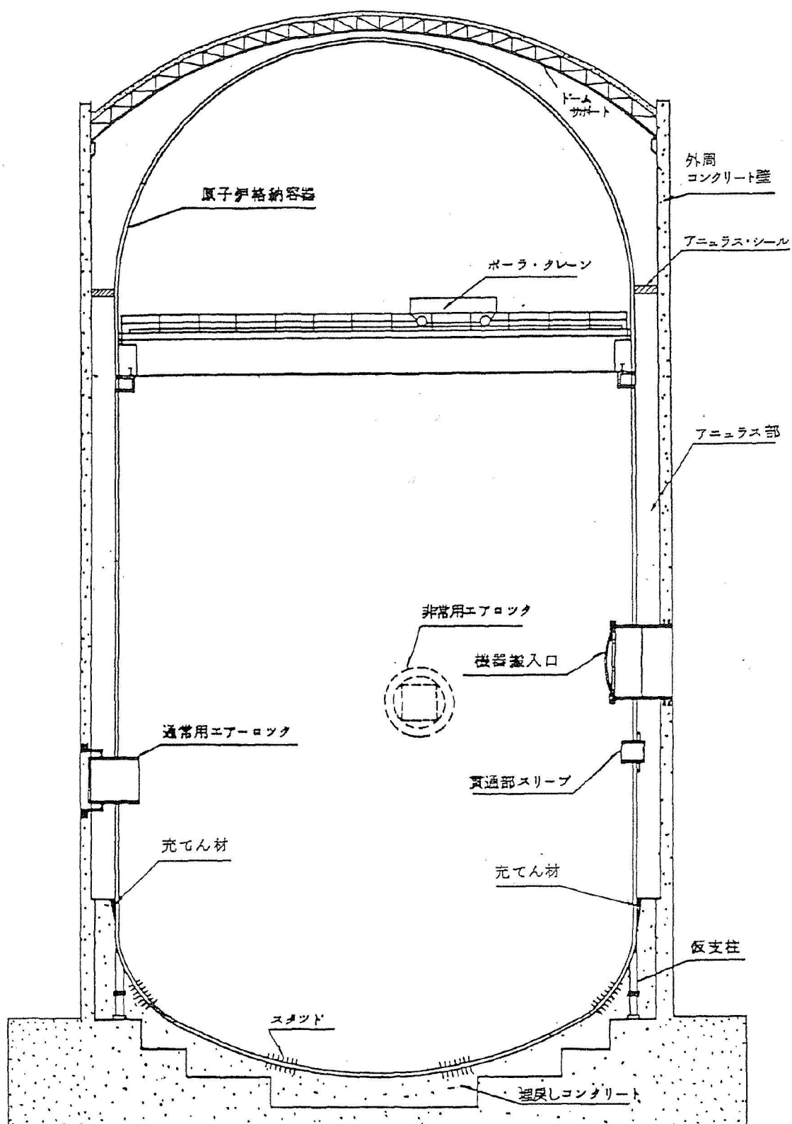
第1.1.1. a-16図 原子炉格納施設の構造概要図
