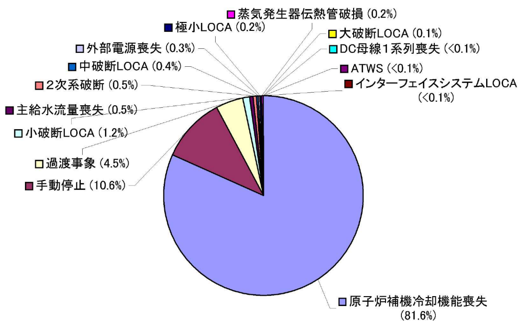
第1. 1. 1. h-1図 起因事象別炉心損傷頻度
