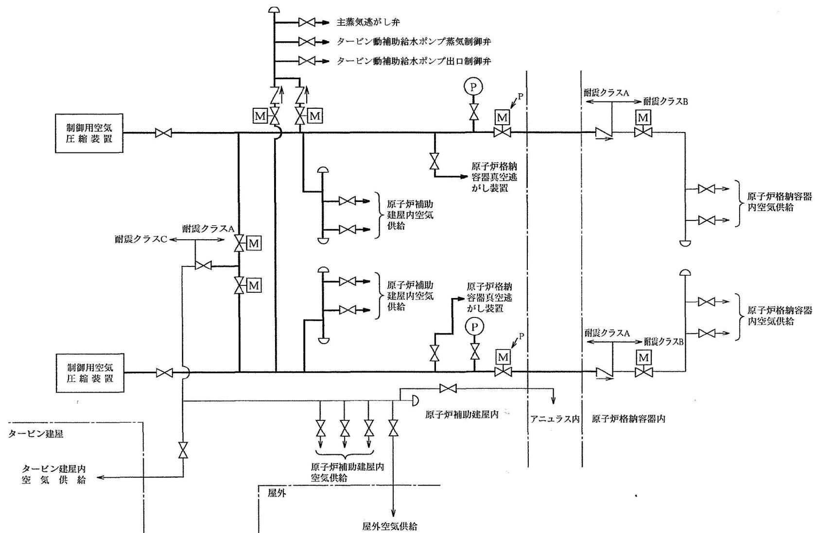
第1.1.1.a-14図 制御用空気設備系統説明図
