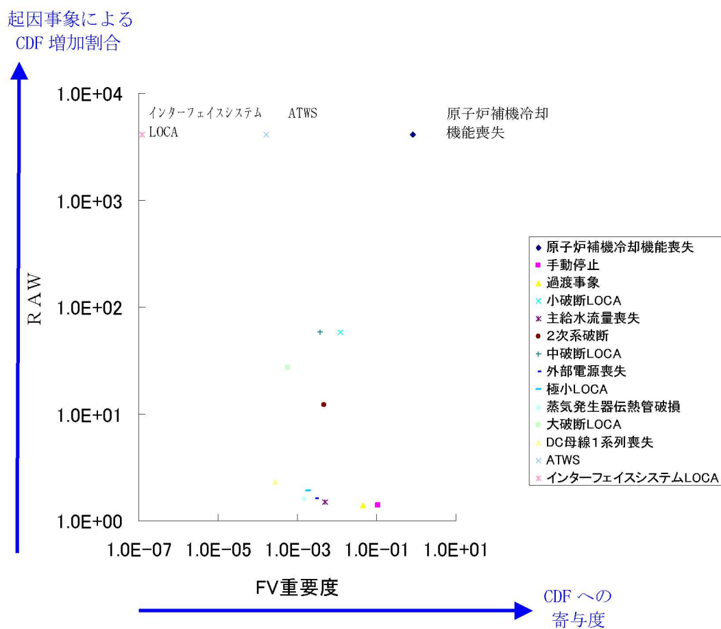
第1. 1. 1. h-2図 全炉心損傷頻度に対する重要度解析結果（起因事象）
