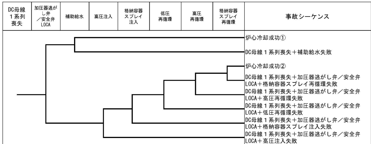
第1.1.1. d-1(n)図 DC母線 1 系列喪失イベントツリー
