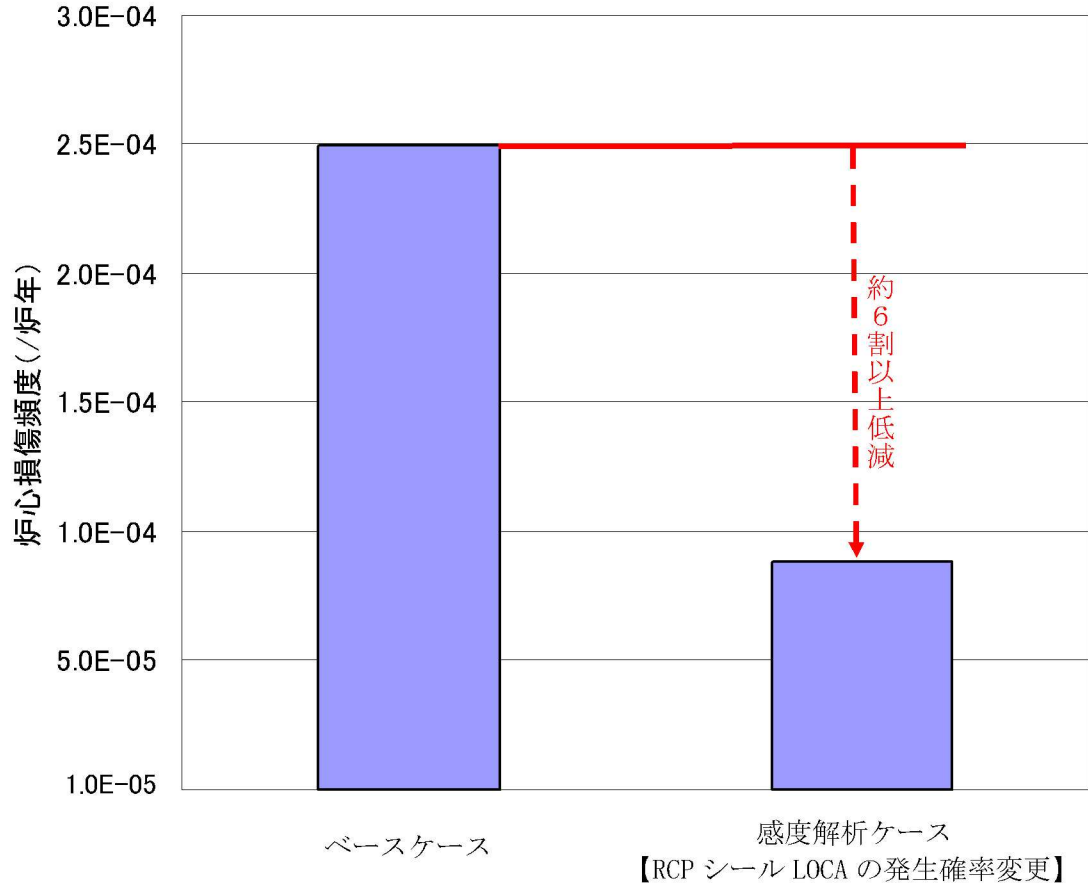
第1. 1. 1. h-6図 全炉心損傷頻度に対する感度解析結果【RCPシールLOCAの発生確率変更】
