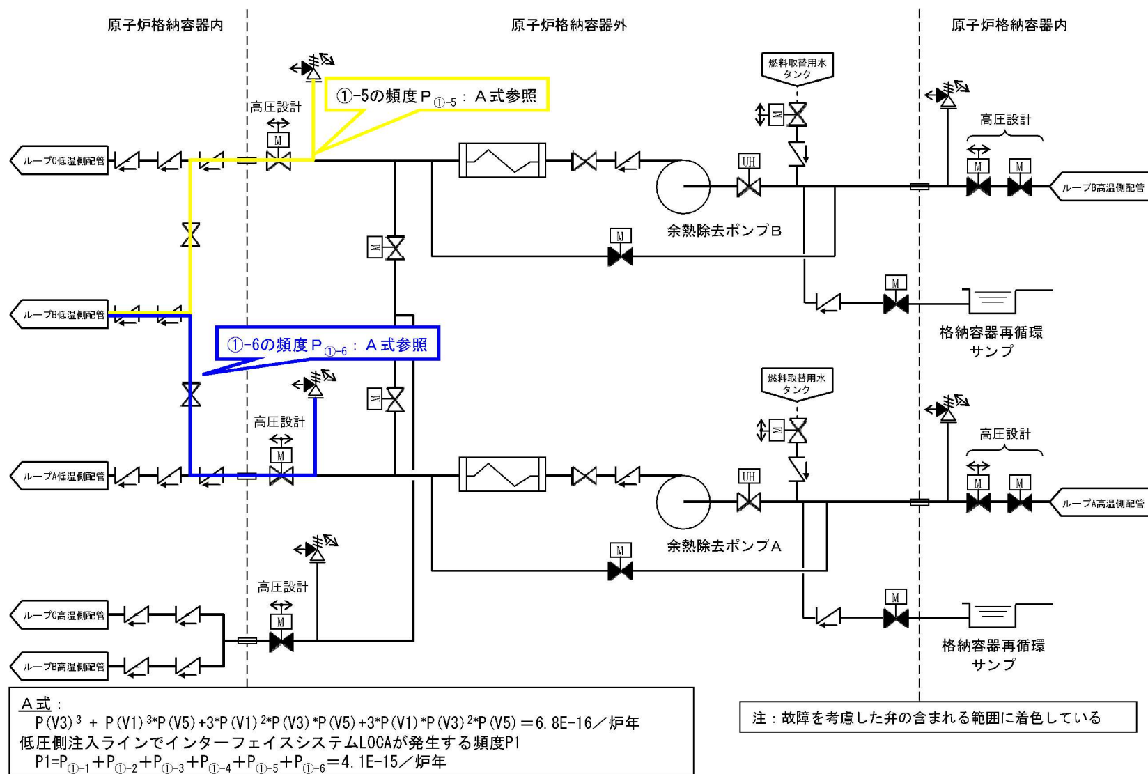
第1.1.1.b-3図 (2/4) インターフェイスシステムLOCAの想定
