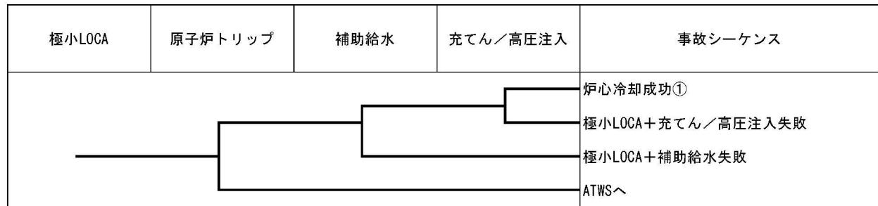
第1.1.1. d-1 (d) 図 極小LOCAイベントツリー
