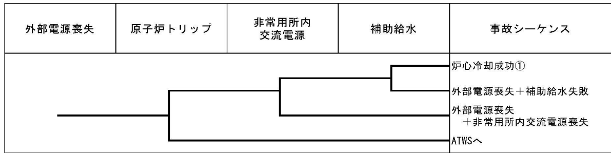
第1.1.1. d-1(h) 図 外部電源喪失イベントツリー
