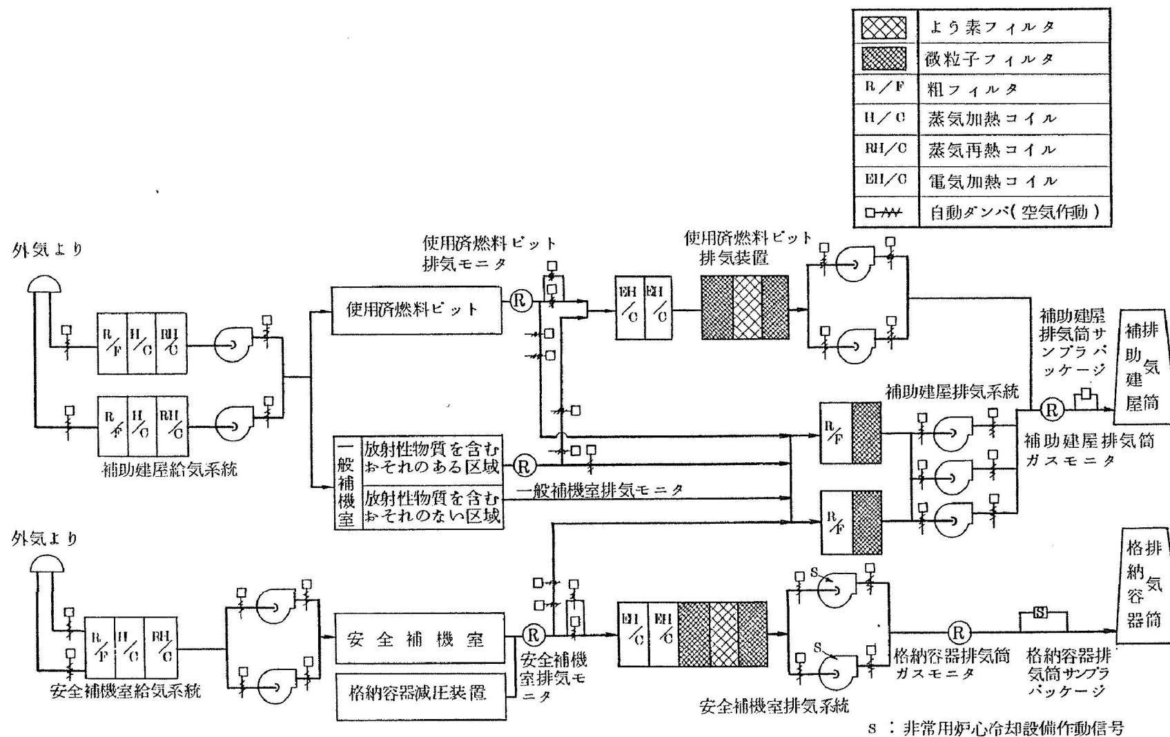
第1.1.1.a-13図 補助建屋換気空調設備系統説明図 (一般補機室及び安全補機室)
