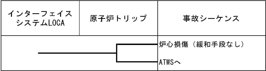
第1. 1. 1. d-1(e)図 インターフェイスシステムLOCAイベントツリー
