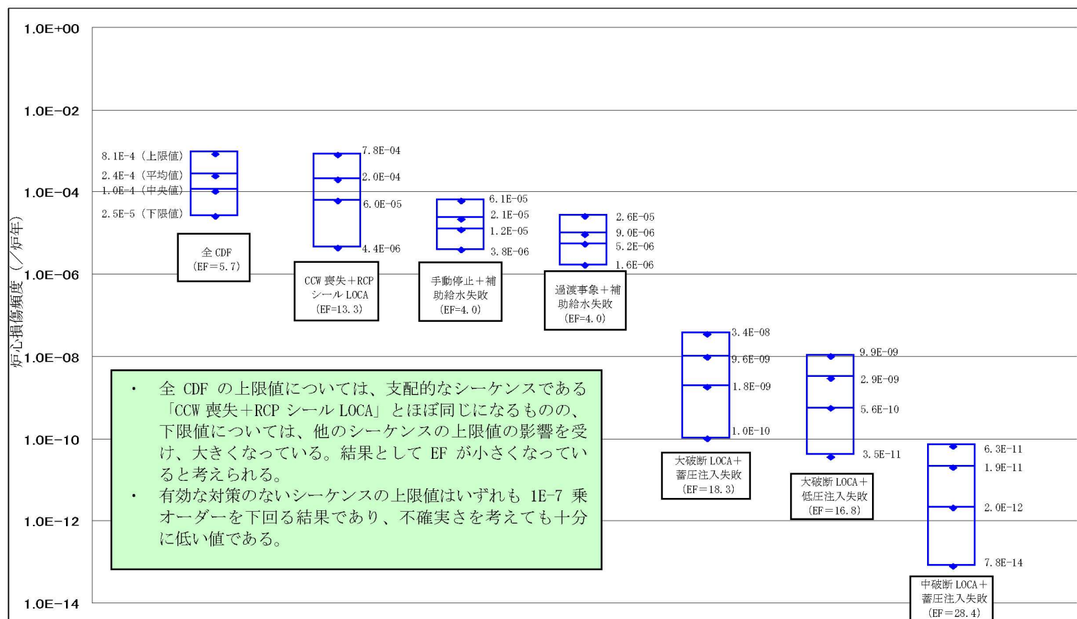
第1.1.1.h-5図 全炉心損傷頻度及び事故シーケンス別炉心損傷頻度に対する不確実さ解析結果
