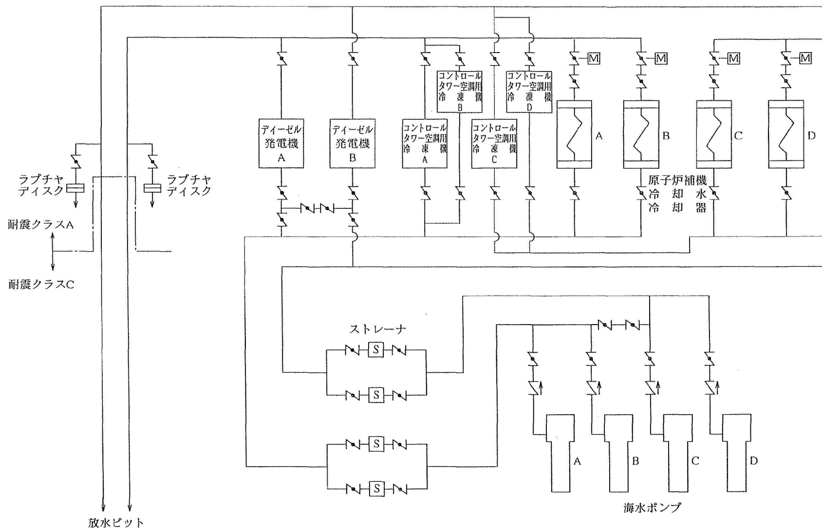
第1.1.1. a-12図 原子炉補機冷却海水設備系統説明図
