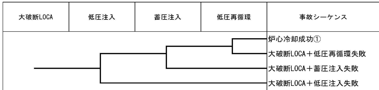
第1.1.1.d-1(a)図 大破断LOCAイベントツリー
