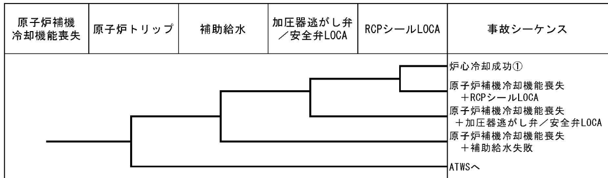
第1.1.1. d-1(1) 図 原子炉補機冷却機能喪失イベントツリー
