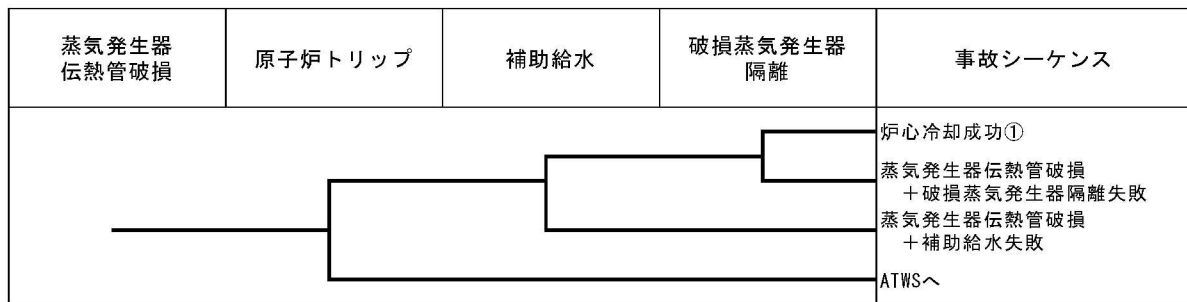
第1.1.1. d-1(k)図 蒸気発生器伝熱管破損イベントツリー
