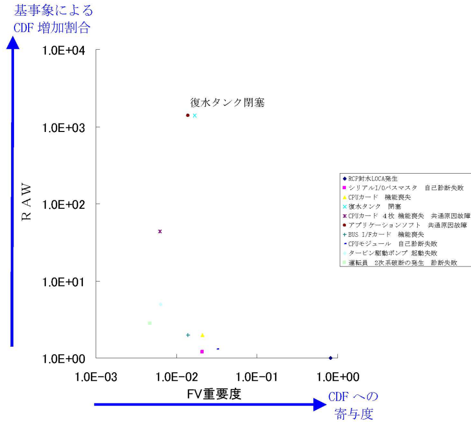
第1. 1. 1. h-3図 全炉心損傷頻度に対する重要度解析結果（基事象－FV重要度）
