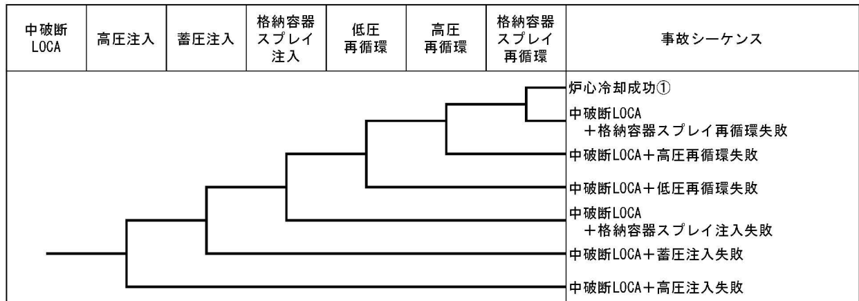
第1.1.1.d-1(b)図 中破断LOCAイベントツリー
