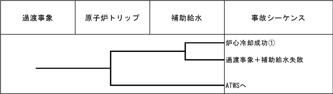
第1. 1. 1. d-1 (g) 図 過渡事象イベントツリー
