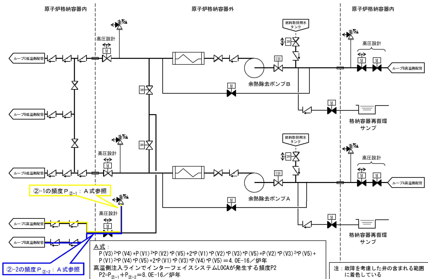
第1.1.1.b-3図 (3/4) インターフェイスシステムLOCAの想定
