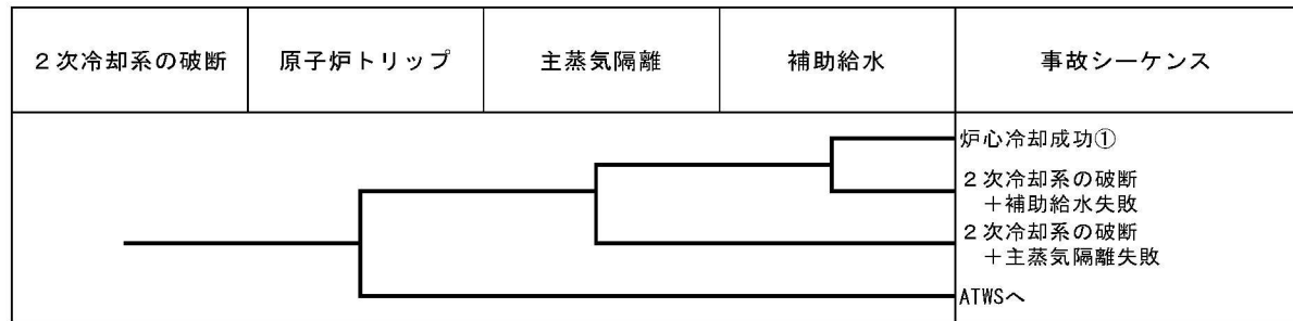
第1.1.1.d-1(j)図 2次冷却系の破断イベントツリー
