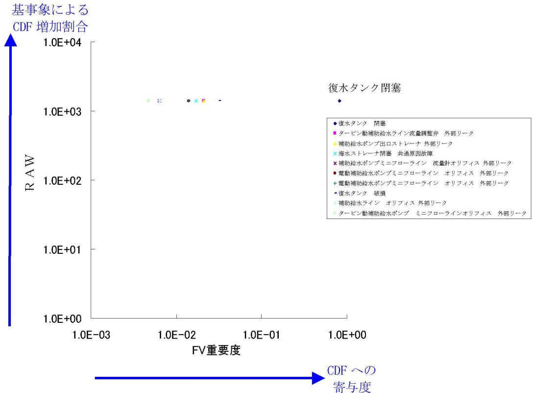
第1. 1. 1. h-4図 全炉心損傷頻度に対する重要度解析結果（基事象－RAW）
