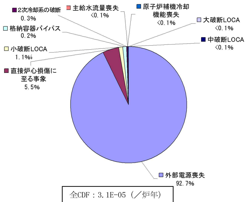
第1.2.1. d-7図 起因事象別炉心損傷頻度 寄与割合
