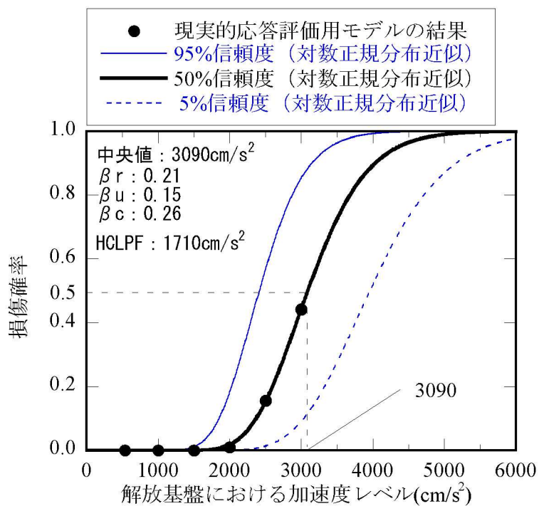
第1.2.1.c-1-7図 川内1号炉原子炉建屋 fragility 曲線とHCLPF (I/C、NS)
