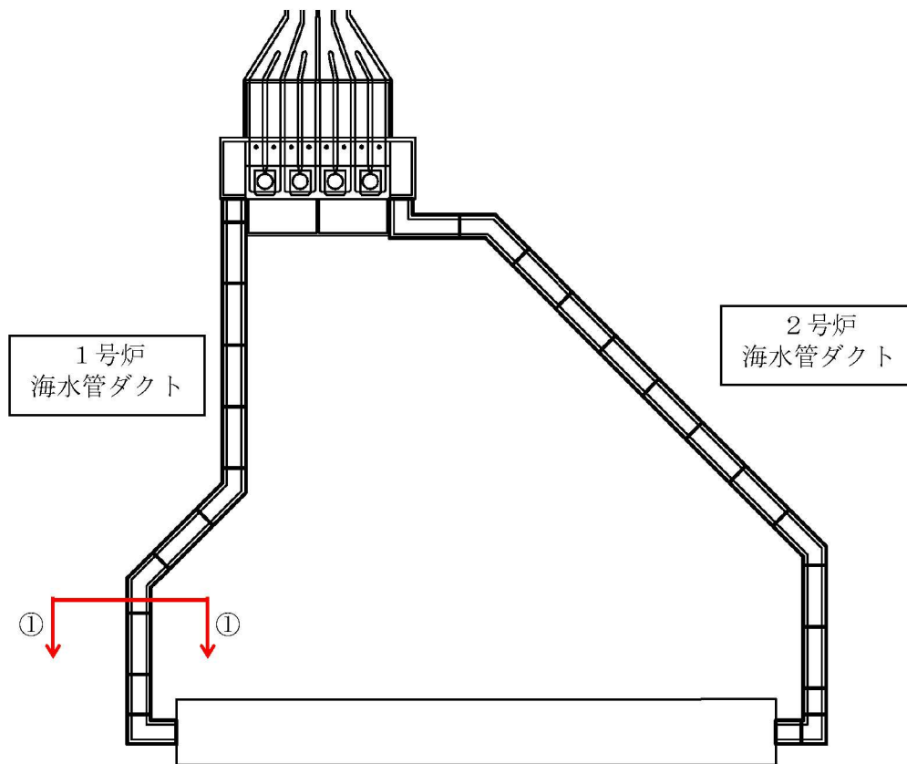
第1.2.1.c-2-1図 海水管ダクト平面図
