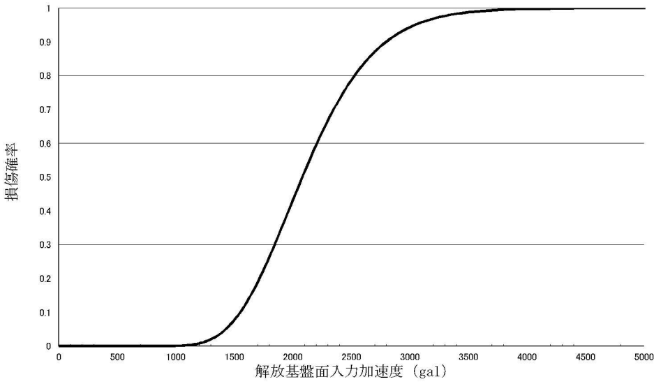
第1. 2. 1. c-3-4図 内燃機関(ディーゼル発電機) フラジリティ曲線
