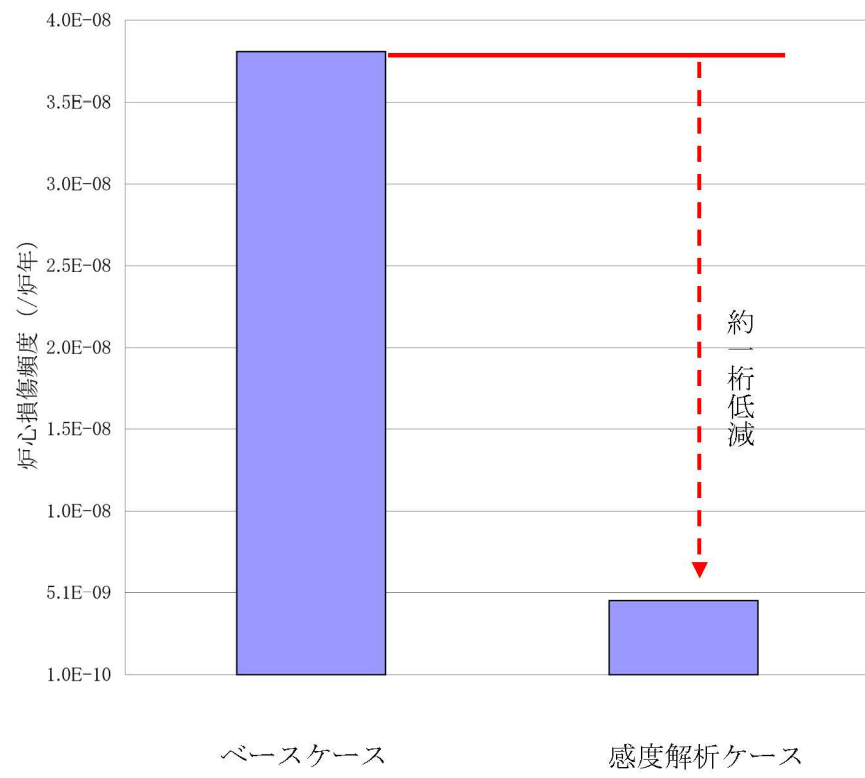
第1.2.2.d-7図 全炉心損傷頻度に対する感度解析結果
