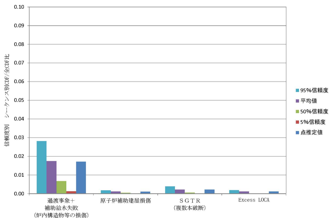
第1.2.1.d-10図 シーケンスごとの不確かさ解析結果
