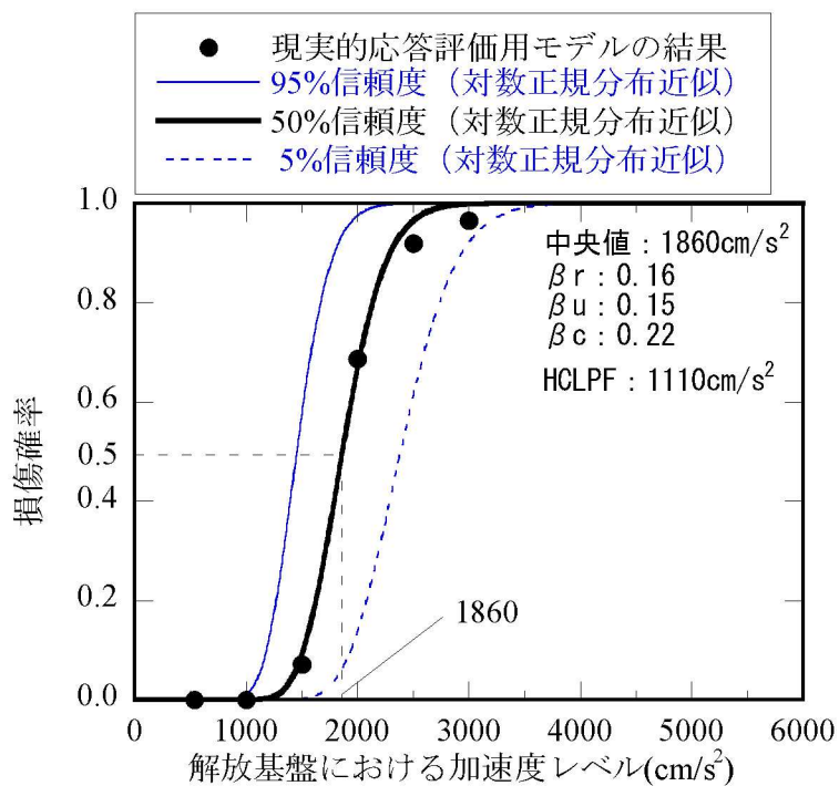
第1.2.1.c-1-8図 川内1号炉原子炉補助建屋 fragility 曲線とHCLPF (A/B、EW)
