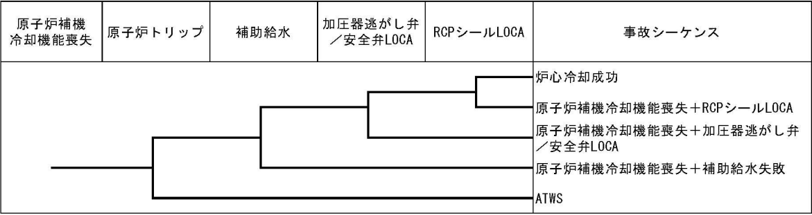
第1. 2. 2. d-2図(a) 原子炉補機冷却機能喪失イベントツリー
