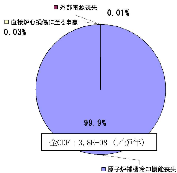
第1.2.2. d-3図 起因事象別炉心損傷頻度 寄与割合
