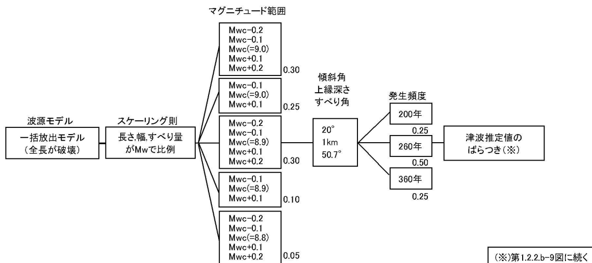
第1.2.2.b-8図 遠地（南米沖）の地震（P-1：南米ペルー沖）を波源とするロジックツリー
