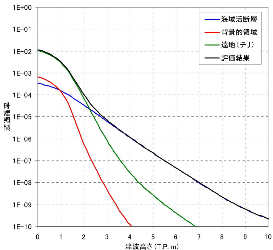
第1.2.2.b-10図 取水口地点における水位と年超過確率の関係
