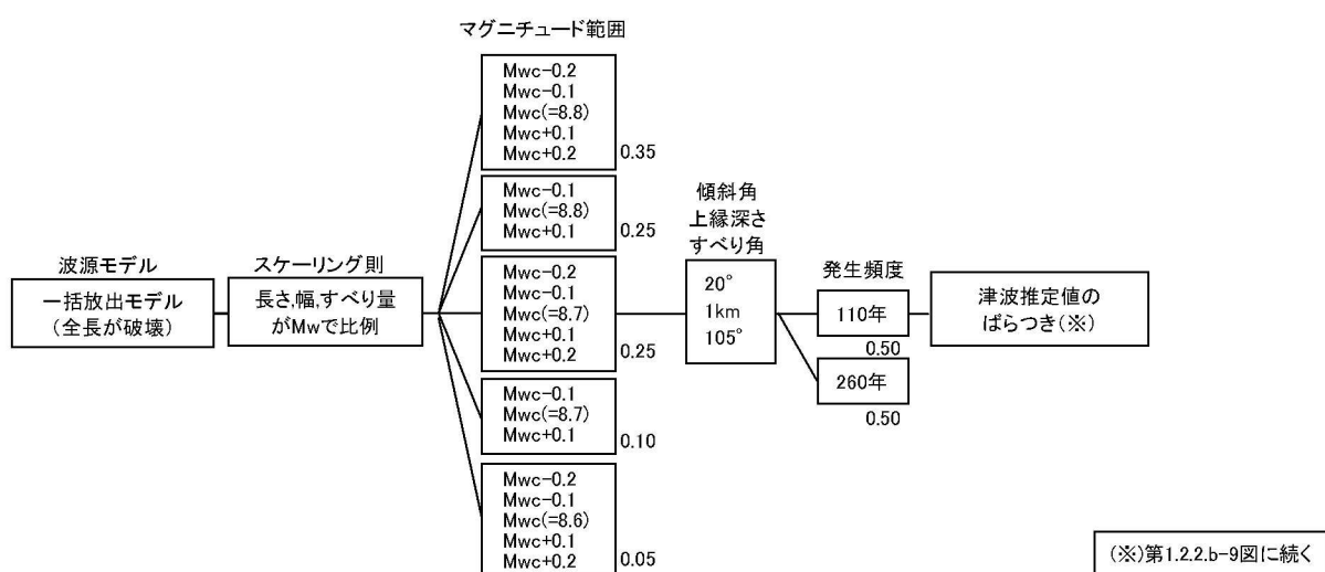
第1.2.2.b-7図 遠地（南米沖）の地震（C-10：南米チリ北部沖）を波源とするロジックツリー
