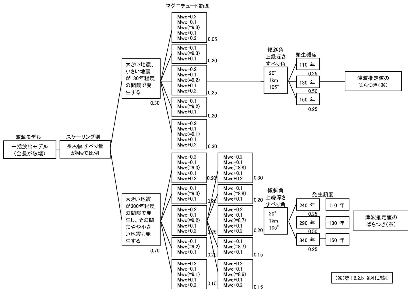
第1.2.2.b-6図 遠地（南米沖）の地震（C-3：南米チリ南部沖）を波源とするロジックツリー
