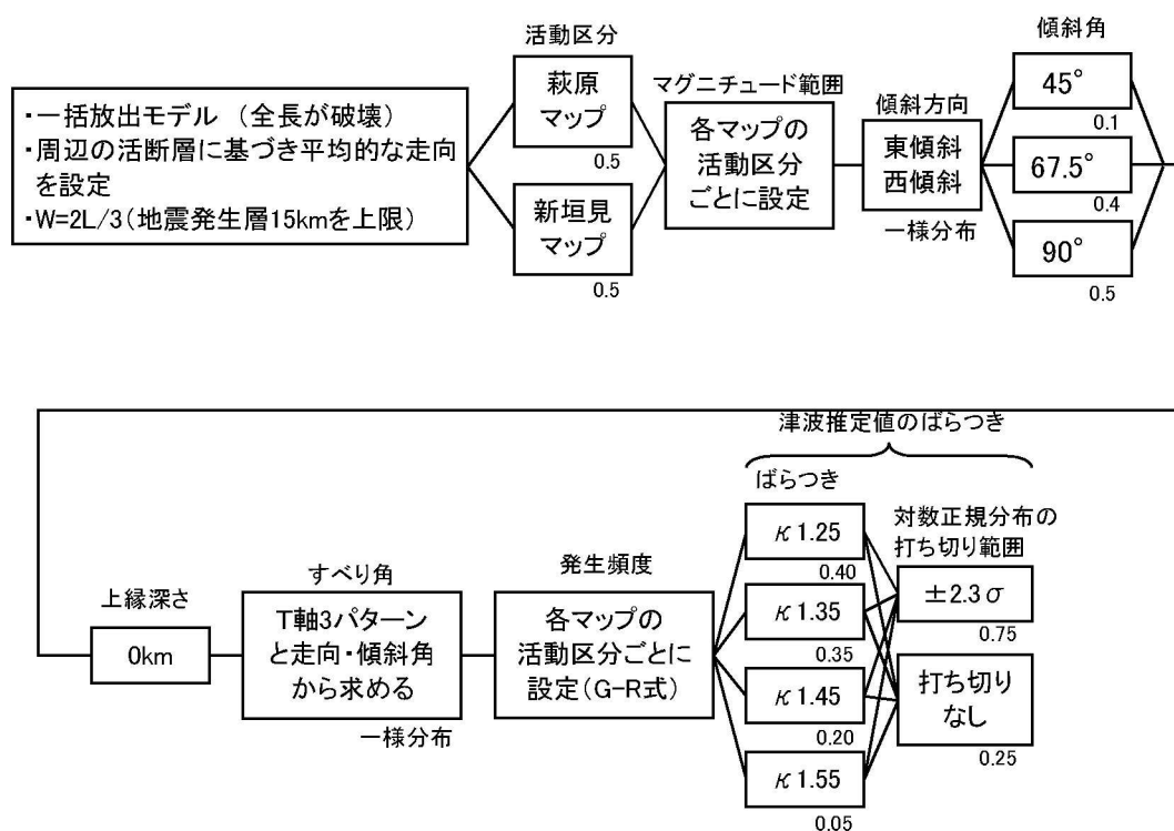
第1. 2. 2. b-5図 背景的領域の地震を波源とするロジックツリー
