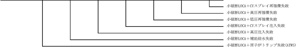
第1. 2. 1. d-6図(c) 小破断LOCAイベントツリー
