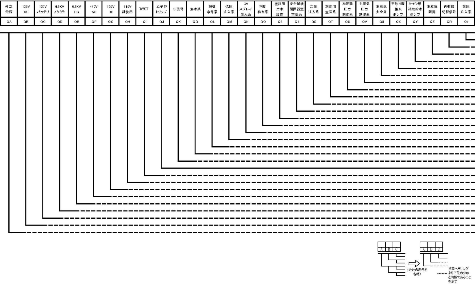
第1. 2. 1. d-3図 地震損傷機器イベントツリー
