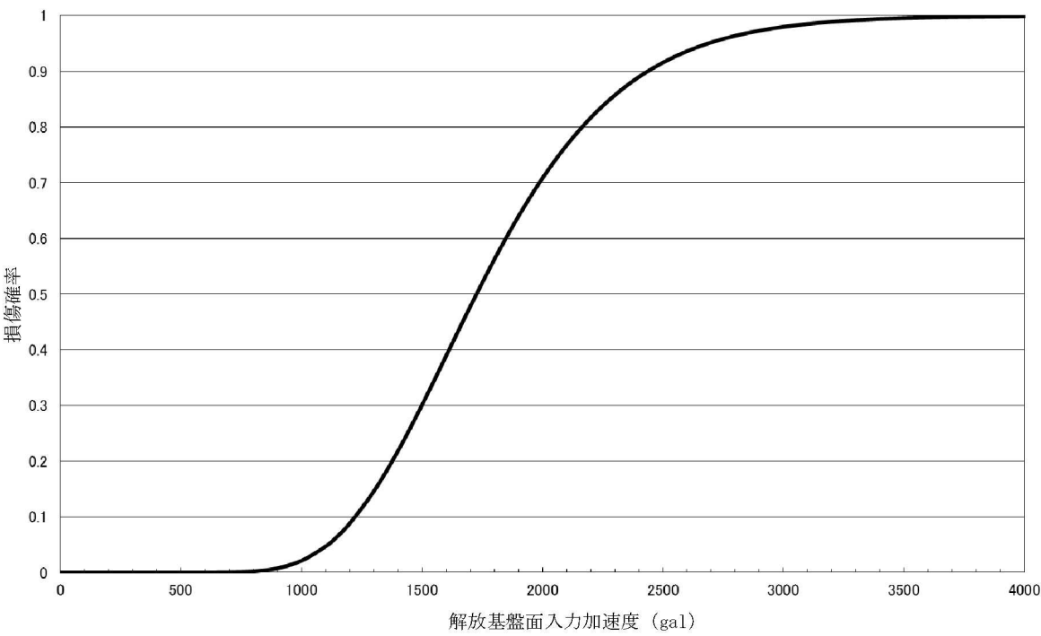
第1. 2. 1. c-3-1図 蒸気発生器 フラジリティ曲線
