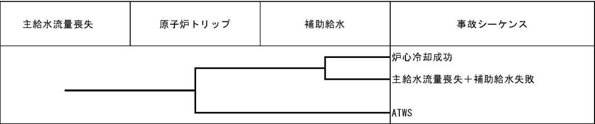
第1. 2. 2. d-2図(c) 主給水流量喪失イベントツリー
