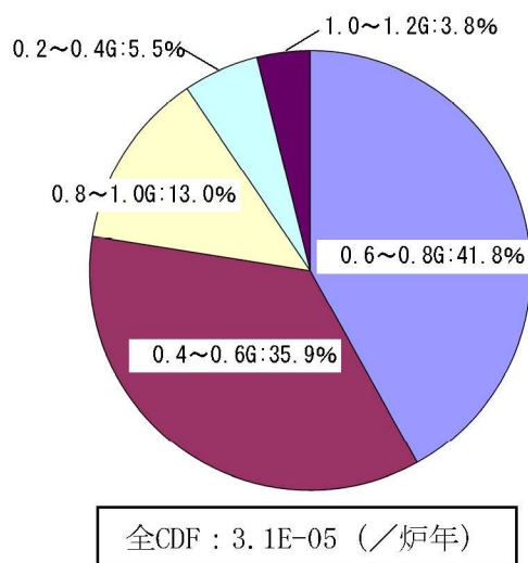
第1.2.1. d-8図 加速度区分ごとの炉心損傷頻度
