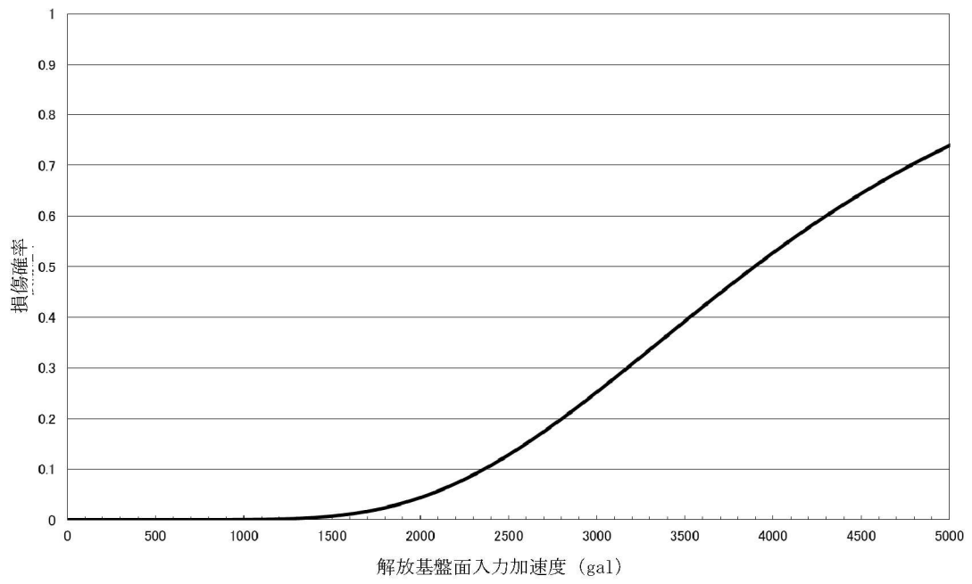
第1. 2. 1. c-3-5図 炉内計装引出管 フラジリティ曲線
