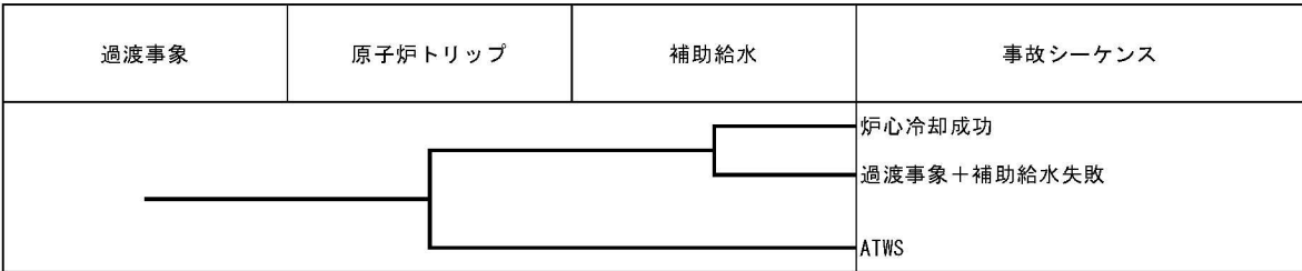
第1. 2. 2. d-2図(d) 過渡事象イベントツリー
