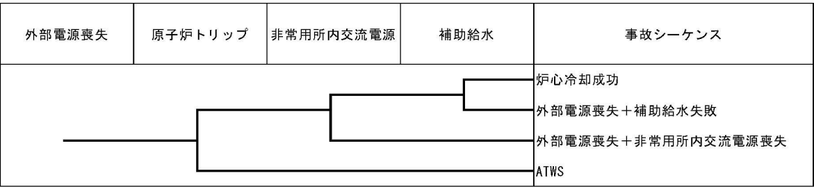
第1. 2. 2. d-2図(b) 外部電源喪失イベントツリー
