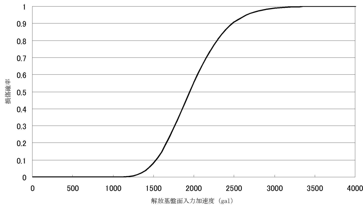
第1. 2. 1. c-3-2図 余熱除去冷却器 フラジリティ曲線
