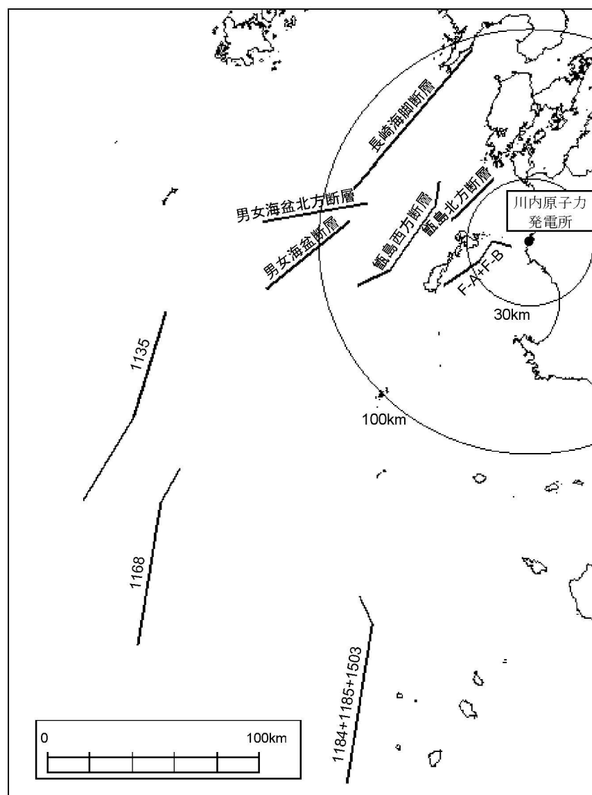
第1.2.2. b-1図 海域の活断層の対象波源
