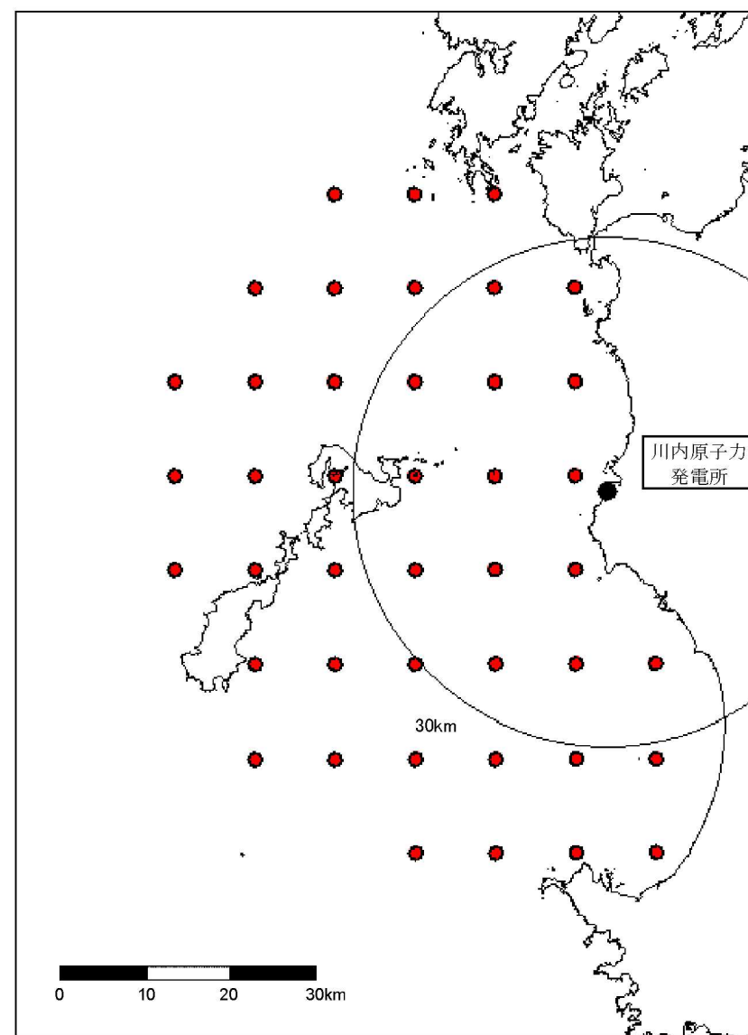
第1.2.2. b-2図 背景的領域の対象波源
