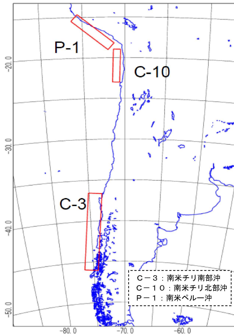
第1.2.2. b-3図 遠地（南米沖）の地震の対象波源
