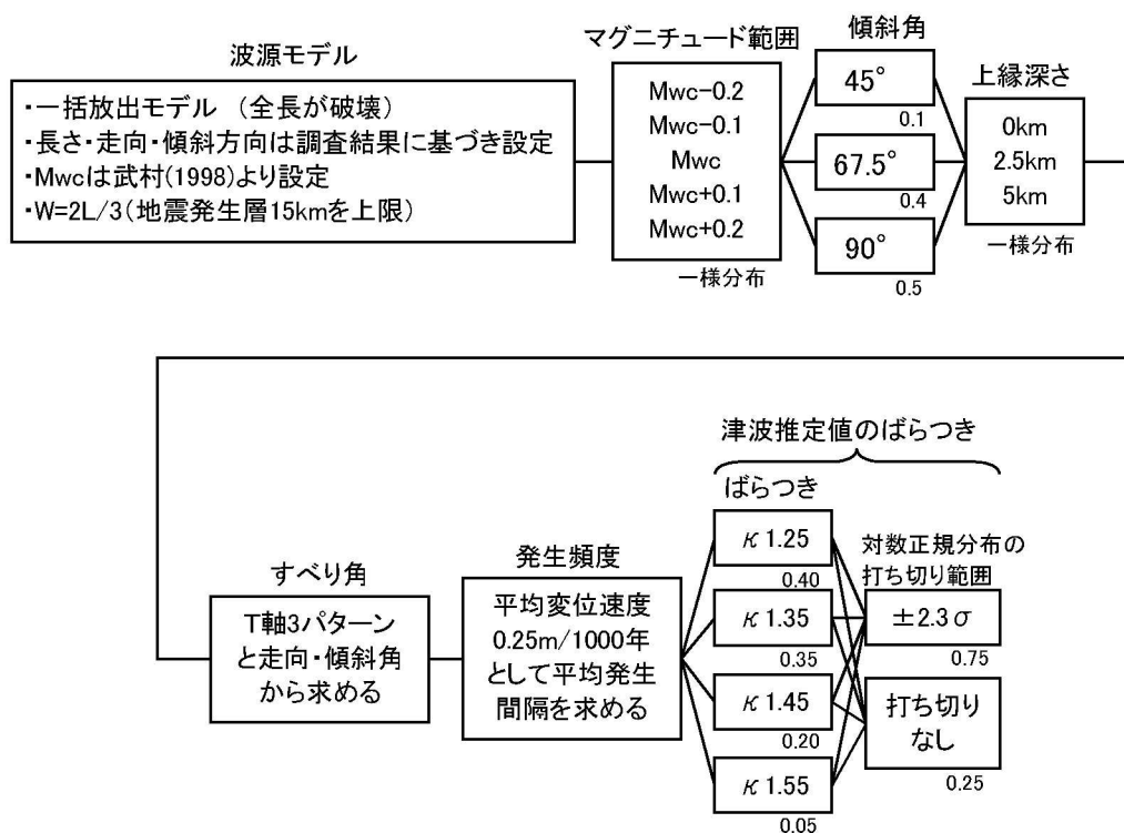
第1. 2. 2. b-4図 海域の活断層の地震を波源とするロジックツリー
