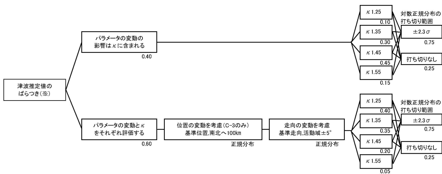
第1.2.2.b-9図 遠地（南米沖）の地震を波源とするロジックツリーにおける津波推定値のばらつき
