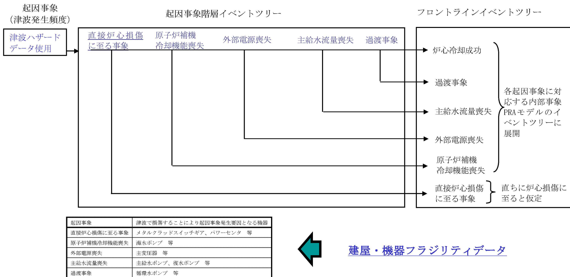
第1.2.2. d-1図 津波PRA階層イベントツリー
