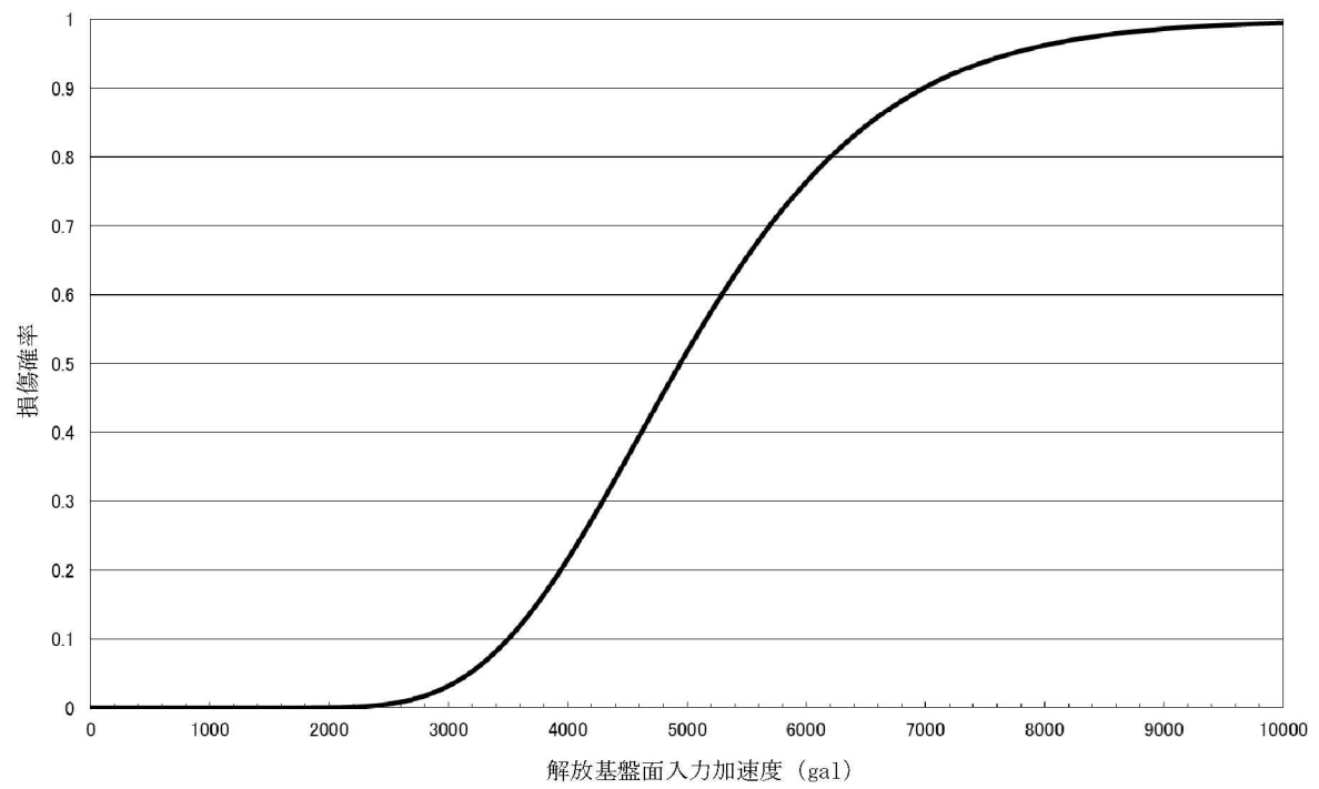
第1.2.1.c-3-3図 原子炉ソレノイド用直流分電盤 フラジリティ曲線
