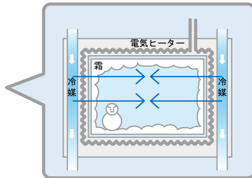
冷却器内部の状況
