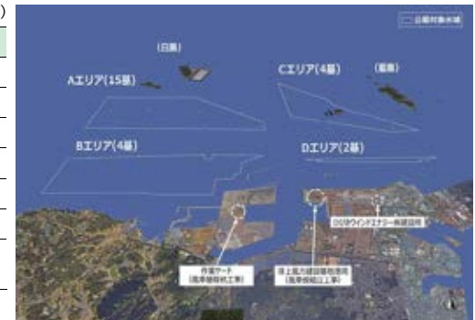
北九州響灘洋上ウインドファームの事業実施区域(ひびきウインドエナジー株式会社資料より引用) 定格出力9,600kWの風車を25基設置
