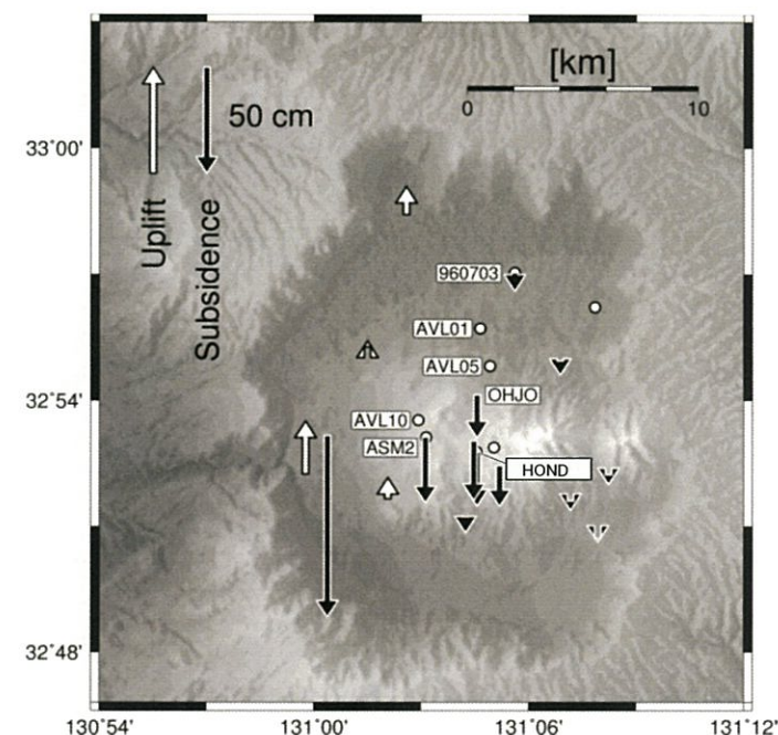
2016年熊本地震時の各GPS観測点における鉛直変動(風間ほか, 2019)
