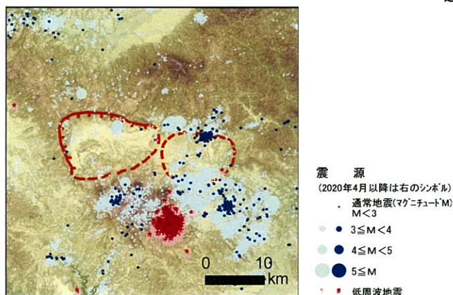
加久藤・小林カルデラの震源分布
