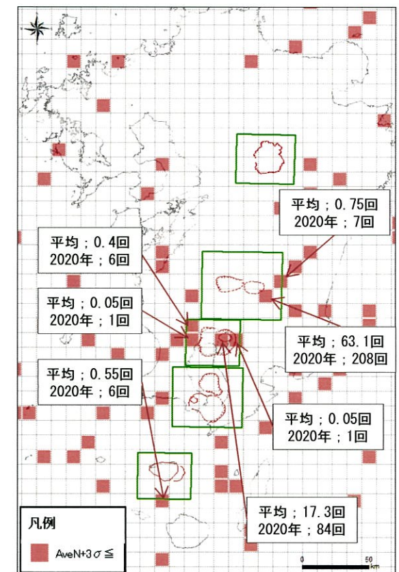
2000～2019年平均地震数(通常地震)と2020年 地震数(通常地震)の比較
