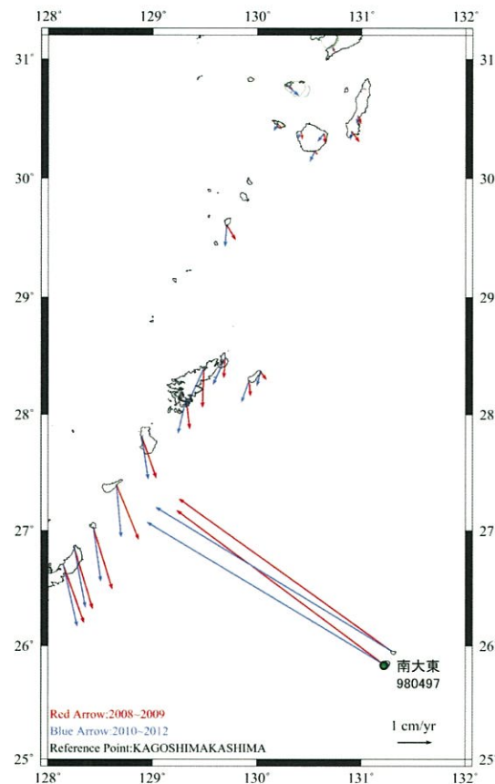
期間(1)→と(2)→のベクトル図
