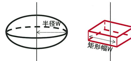
圧力源イメージ:Yamasaki et al.(2020)(左) 本検討(右)
