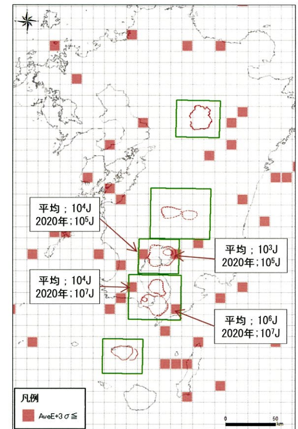
2000～2019年平均地震エネルギー(通常地震) と2020年地震エネルギー(通常地震)の比較
