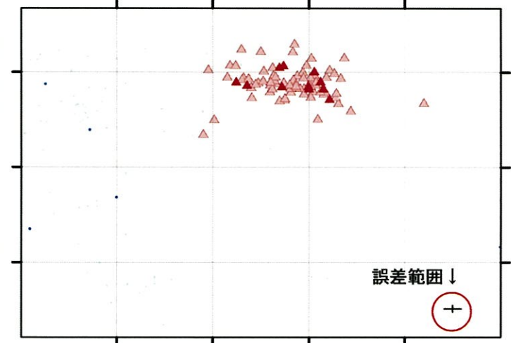
0 10 20 30 40 50 深さ (km)
