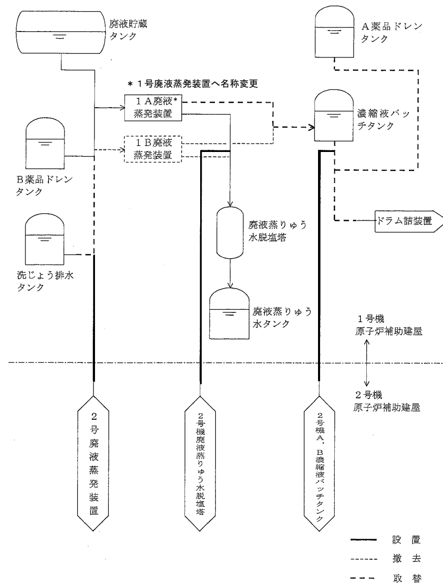
図－６ 液体廃棄物処理設備共用化及び撤去概要図
