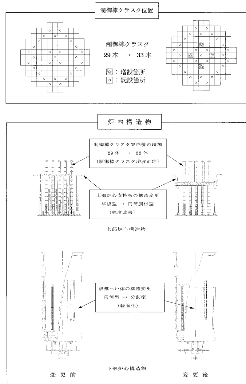
図－２ 制御棒クラスタ増設及び炉内構造物取替え概要図
