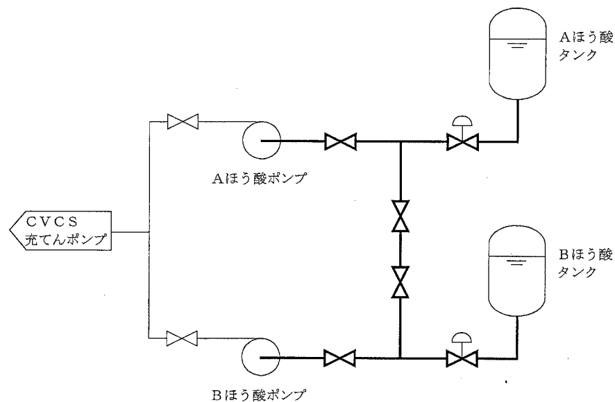
図－５ 化学体積制御設備配管取替概要図
