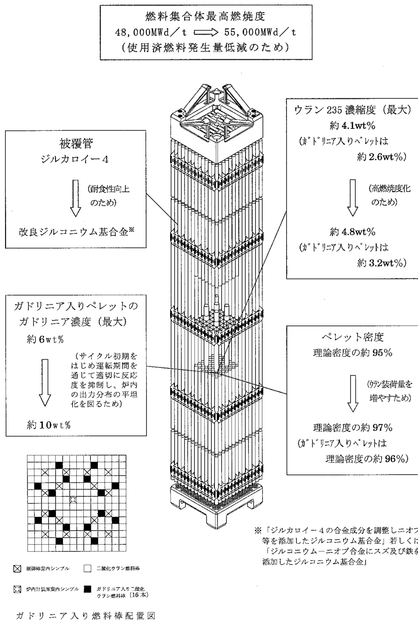
図－１ 燃料集合体概要図
