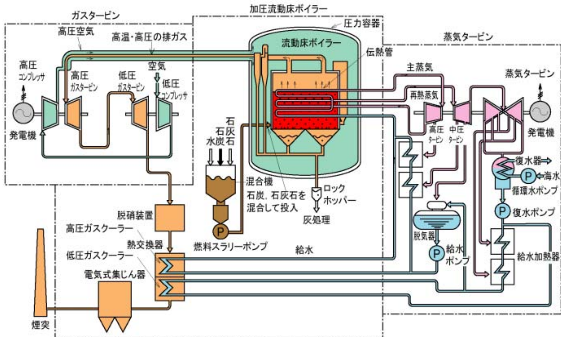
荻田新第1号機 システムフロー図
