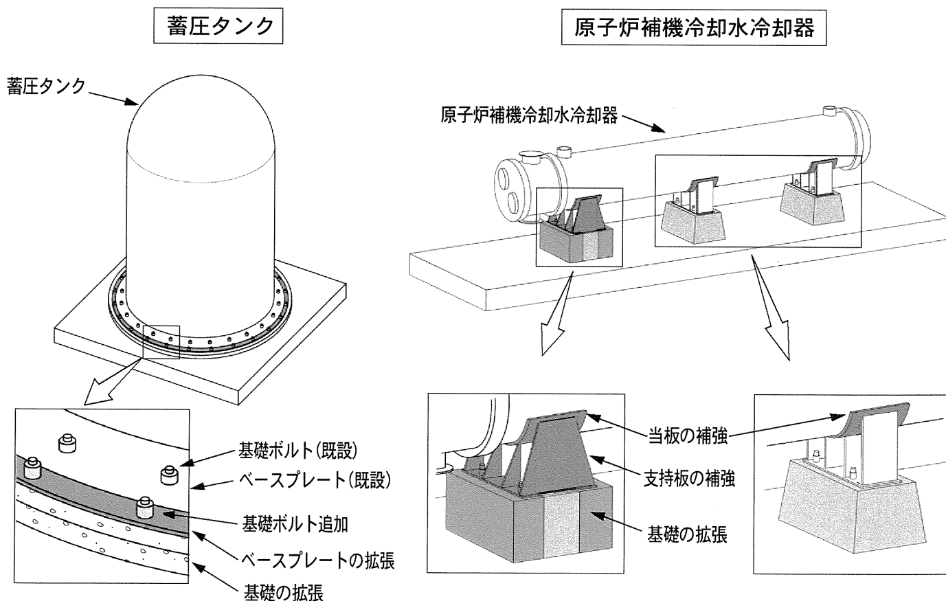
図－4 耐震安全性向上工事概要図
