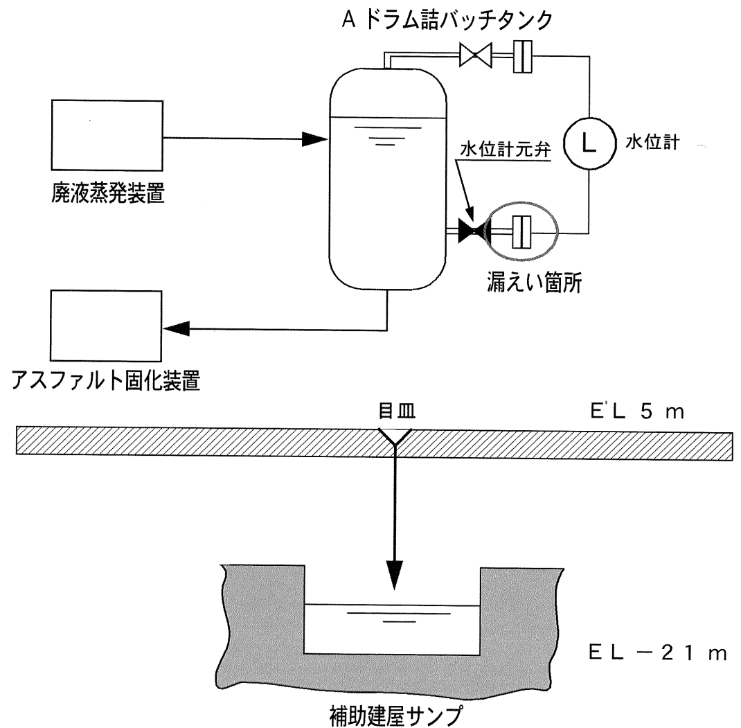
廃棄物処理系統図
