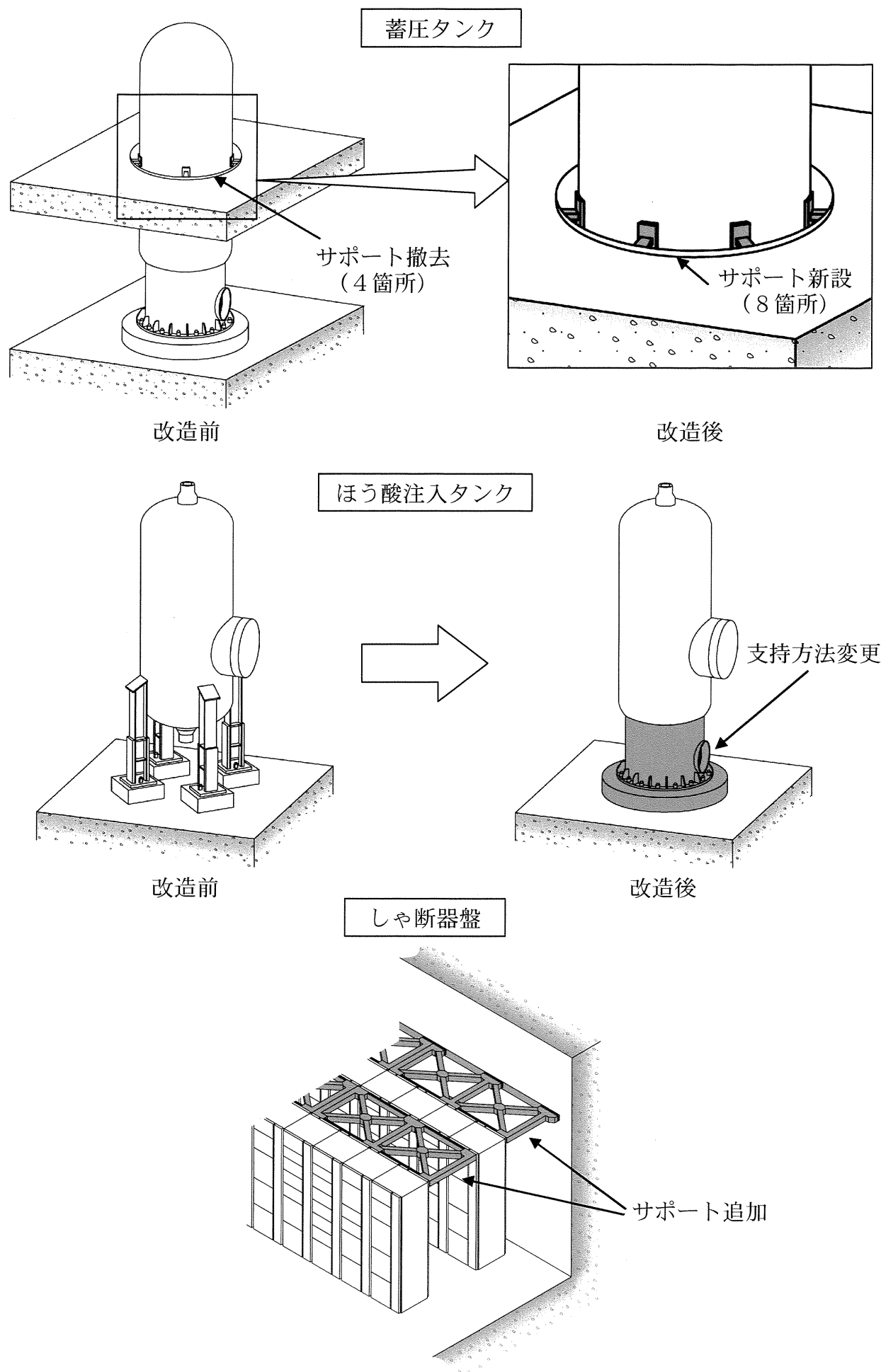
図－１ 耐震安全性向上工事概要図
