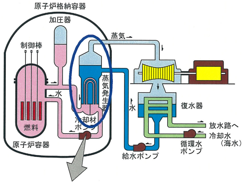
概略系統図
