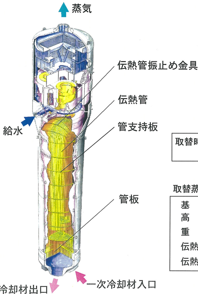
蒸気発生器概略図
