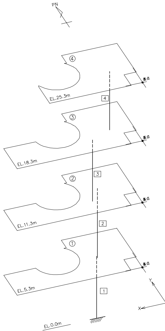
図 2-3 原子炉補助建屋の解析モデル (水平)
