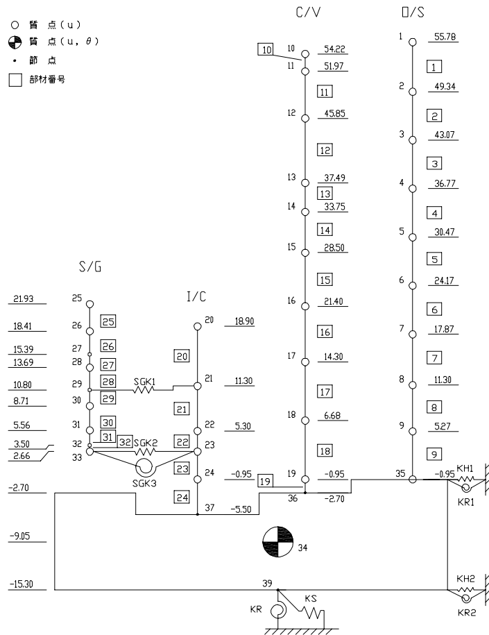
図 2-1 原子炉建屋の解析モデル (水平)
