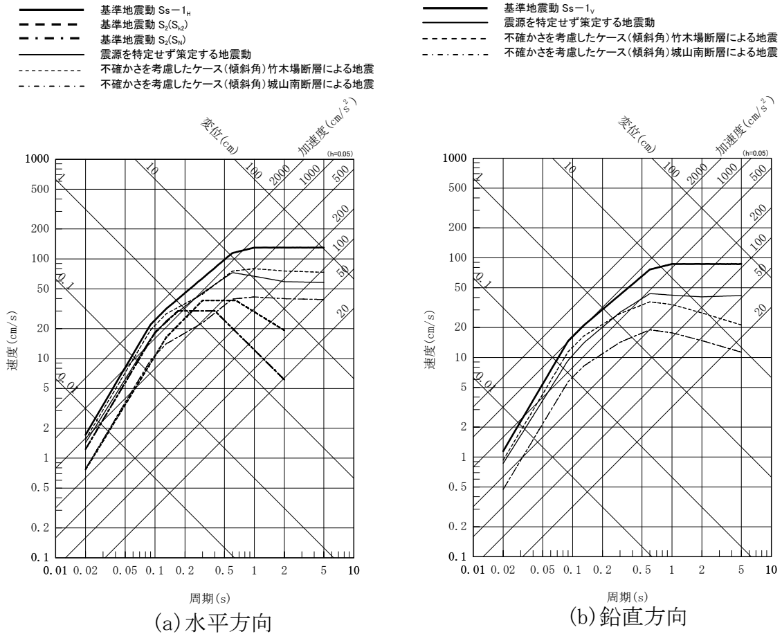
図2 応答スペクトルに基づく地震動評価
