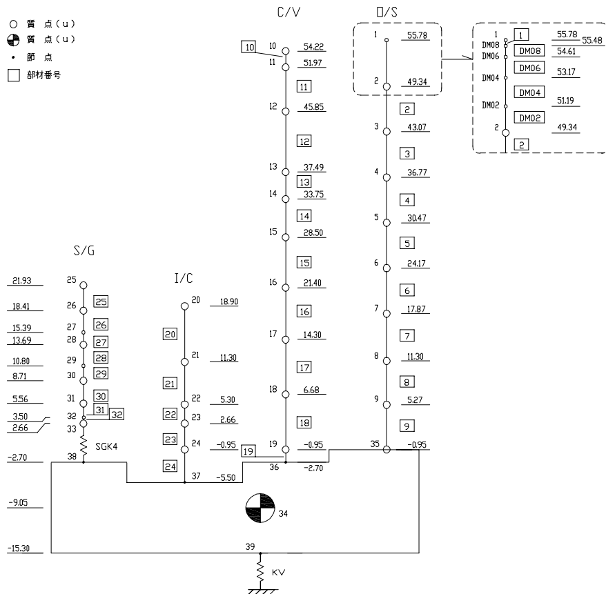
図 2-2 原子炉建屋の解析モデル (鉛直)
