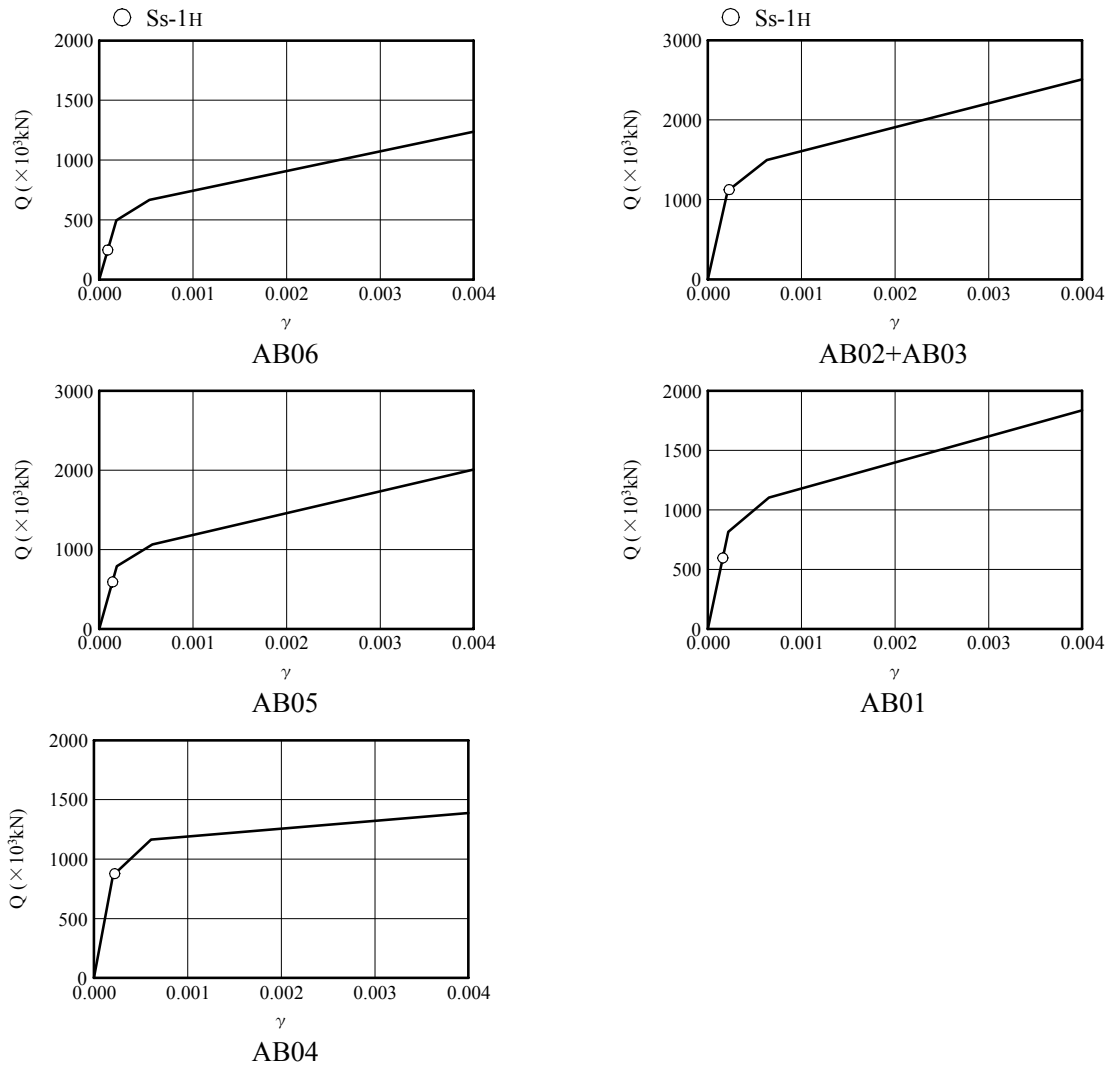
図 2-11-6 Q- \gamma 関係と最大応答値 (原子炉補助建屋 EW方向)
