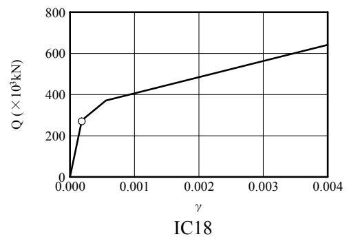
図 2-11-2 Q- \gamma 関係と最大応答値 (原子炉建屋 OS IC NS方向)
