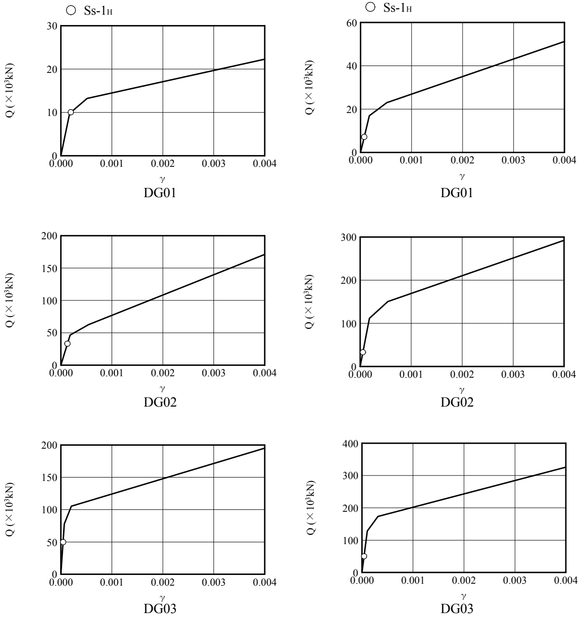
図 2-11-8 Q- \gamma 関係と最大応答値 (ディーゼル建屋 左図：NS方向 右図：EW方向)
