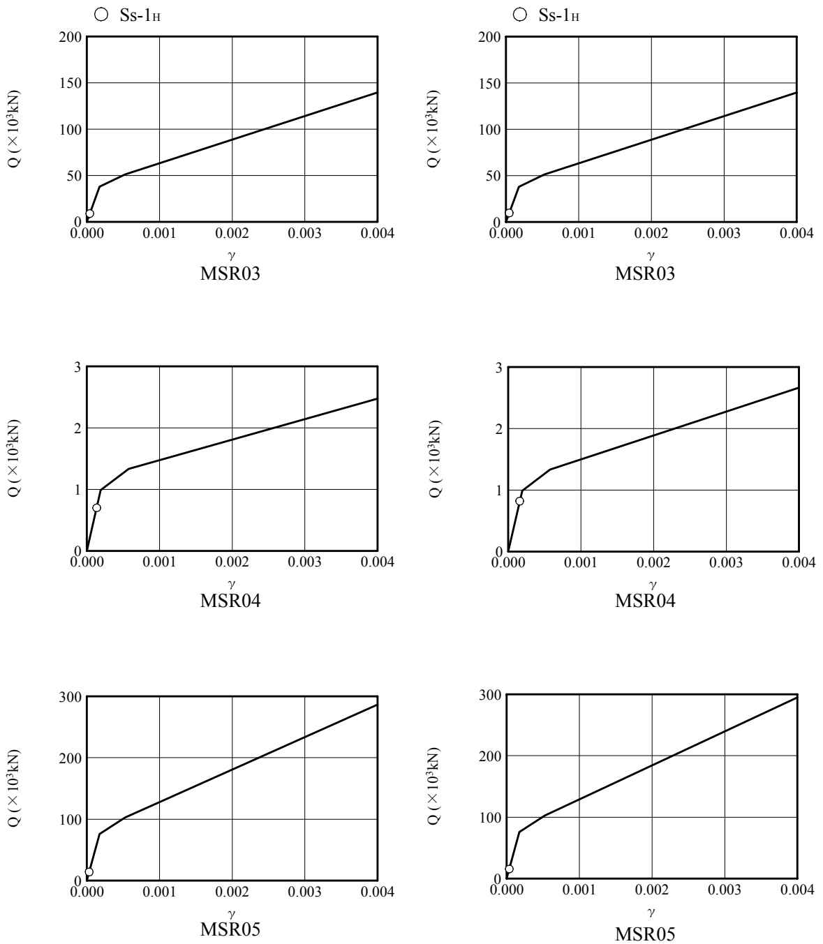
図 2-11-9 Q- \gamma 関係と最大応答値 (主蒸気管室建屋 左図：NS方向 右図：EW方向)
