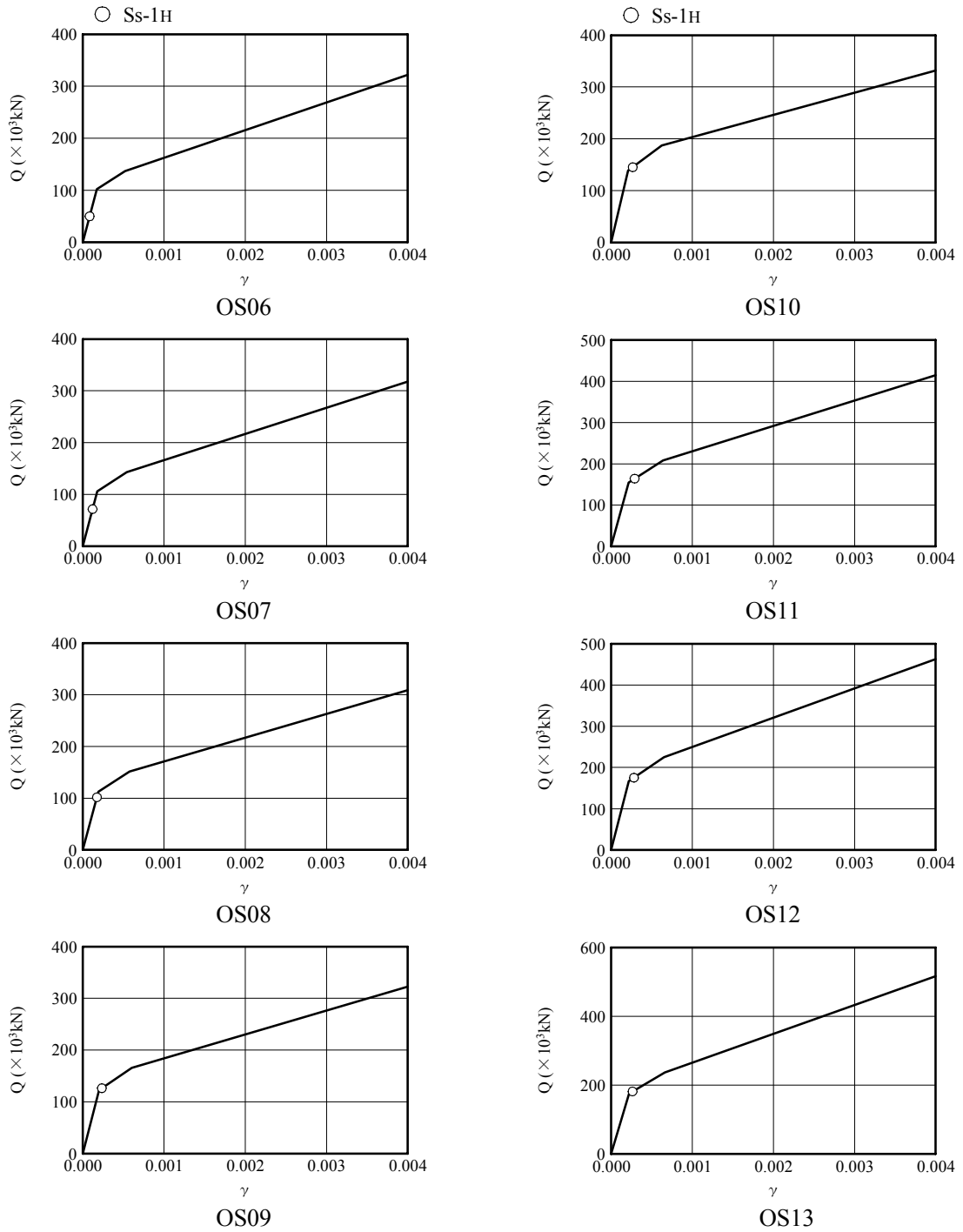
図 2-11-3 Q- \gamma 関係と最大応答値
