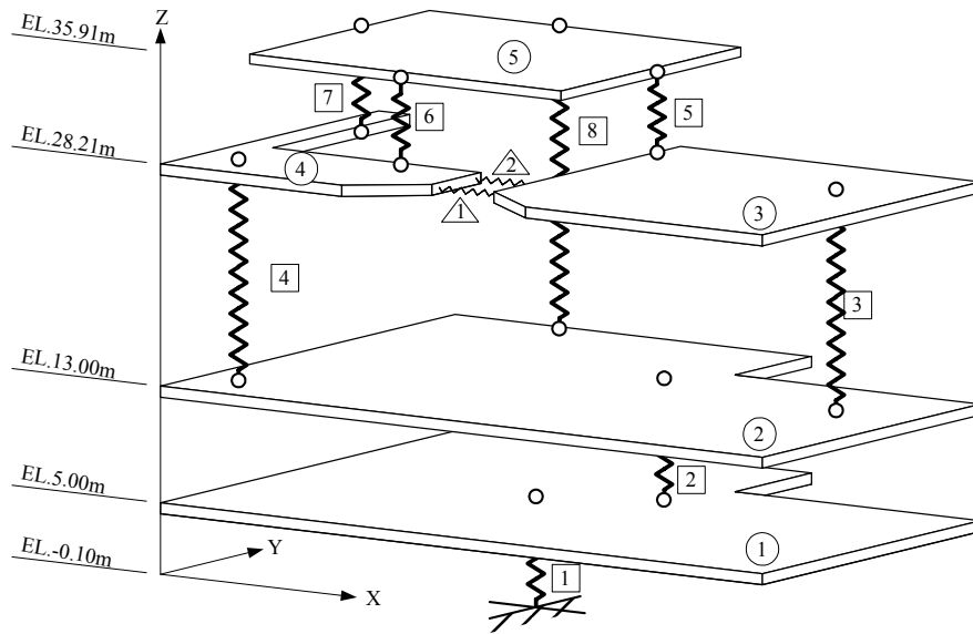
図 2-5 燃料取扱建屋の解析モデル (水平)
