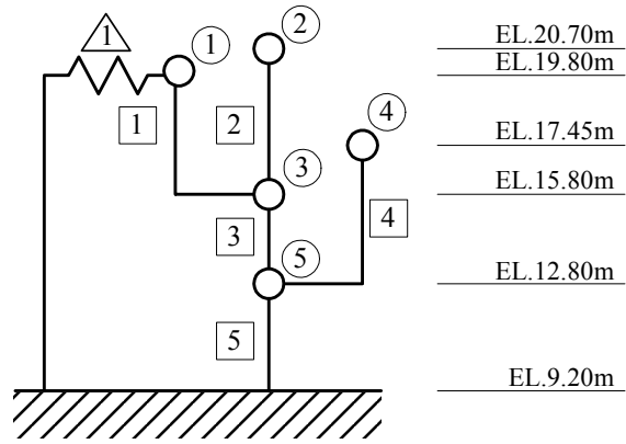
図 2-9 主蒸気管室建屋の解析モデル (水平)
