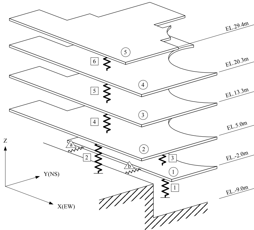
図 2-3 原子炉補助建屋の解析モデル (水平)
