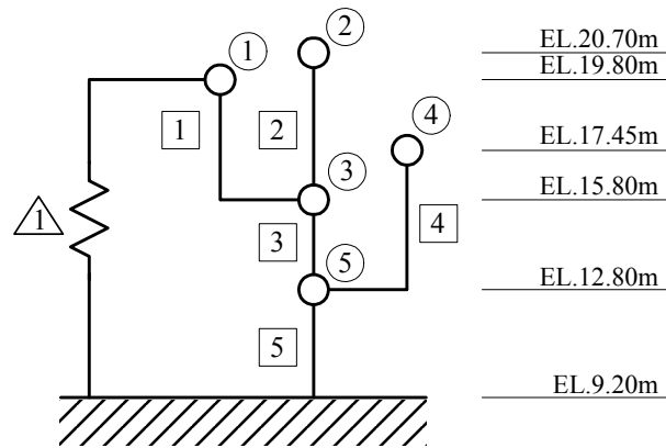
図 2-10 主蒸気管室建屋の解析モデル (鉛直)
