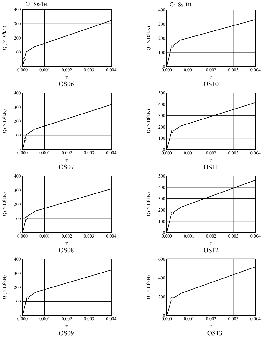
図 2-11-1 Q- \gamma 関係と最大応答値
