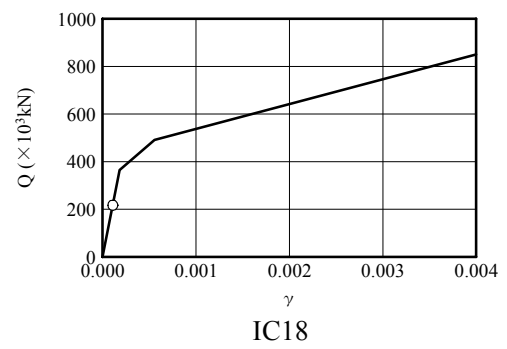
図 2-11-4 Q- \gamma 関係と最大応答値 (原子炉建屋 OS IC EW方向)
