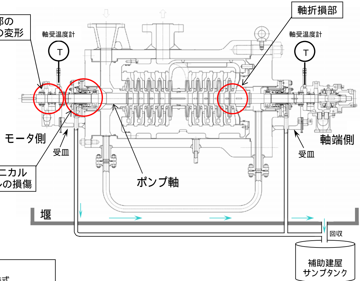
ポンプ構造図
