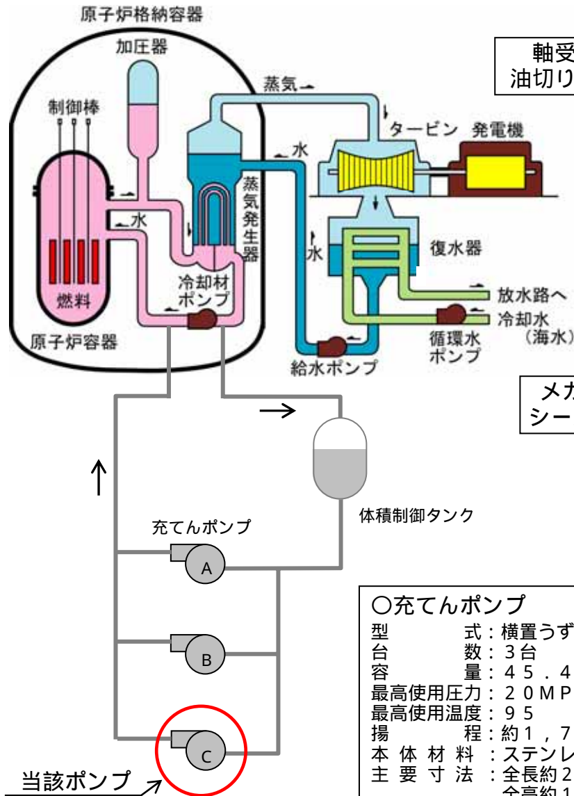
概略系統図
