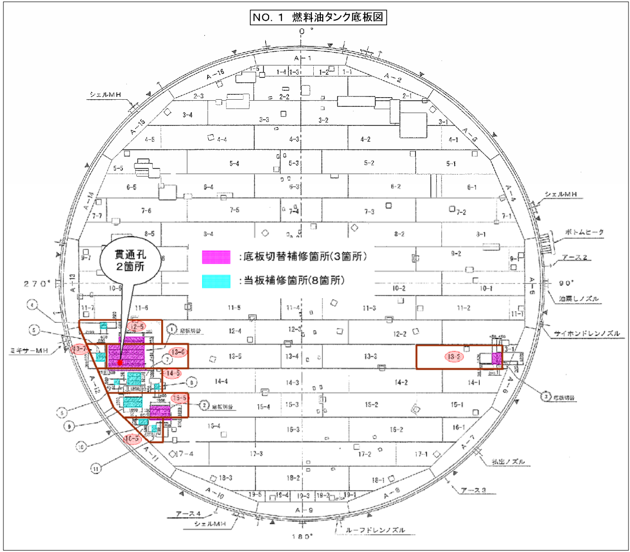
相浦発電所 燃料油タンク点検補修状況
