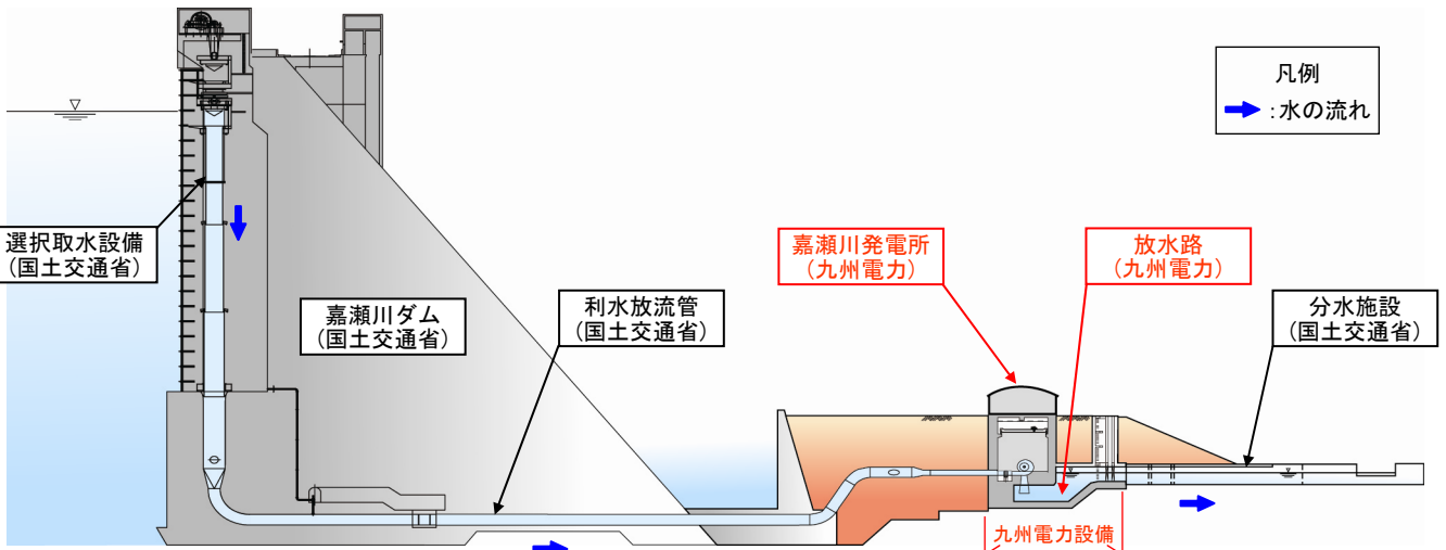
[嘉瀬川ダム・嘉瀬川発電所断面図]
