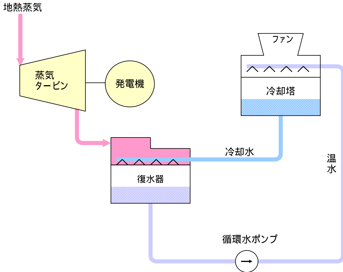
循環水ポンプ概略図
