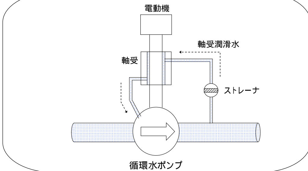
循環水ポンプ概略図
