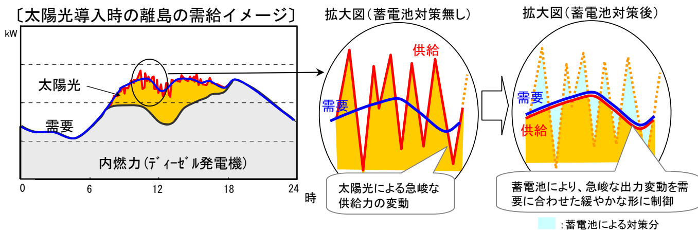
(図2) 蓄電池による太陽光出力変動抑制のイメージ
