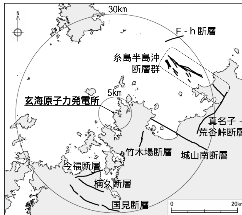
玄海原子力発電所周辺の活断層分布図 (半径30km以内)
