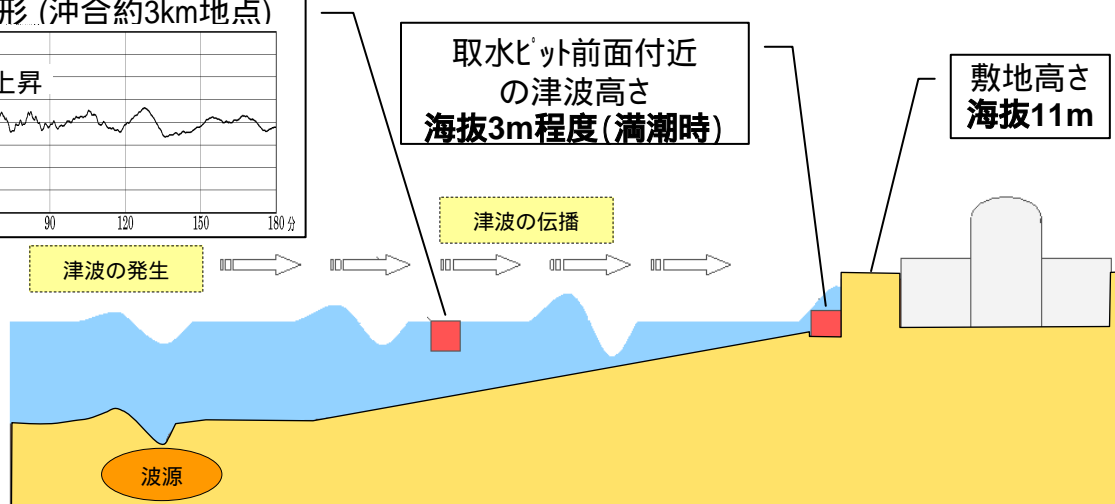
玄海原子力発電所の津波評価の概要
