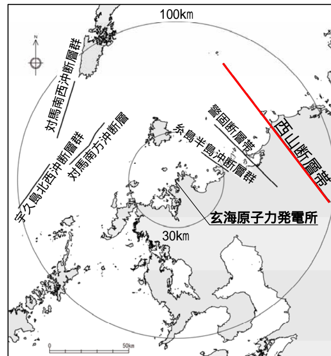
玄海原子力発電所周辺海域の活断層分布図
