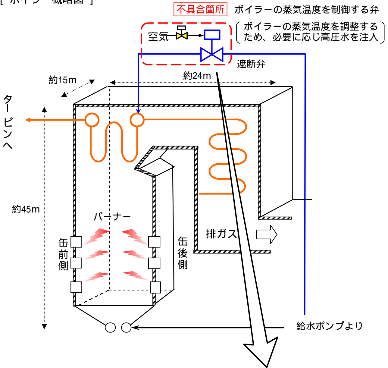
[ ボイラー概略図 ]
