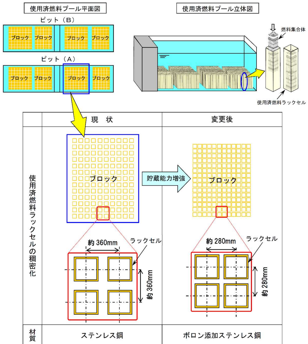
使用済燃料貯蔵設備貯蔵能力増強概要図
