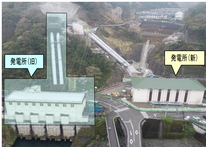
発電所全景
