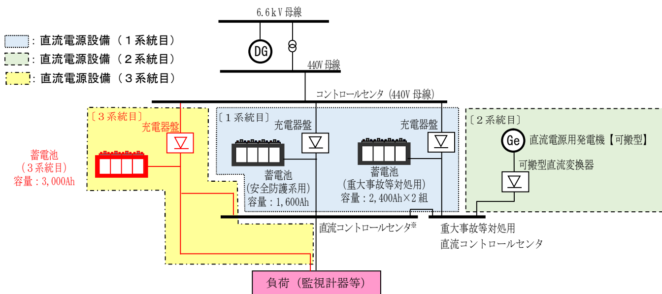
【直流電源設備の系統概要図】
