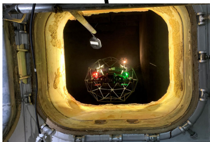
ボイラー内へ入るドローン
