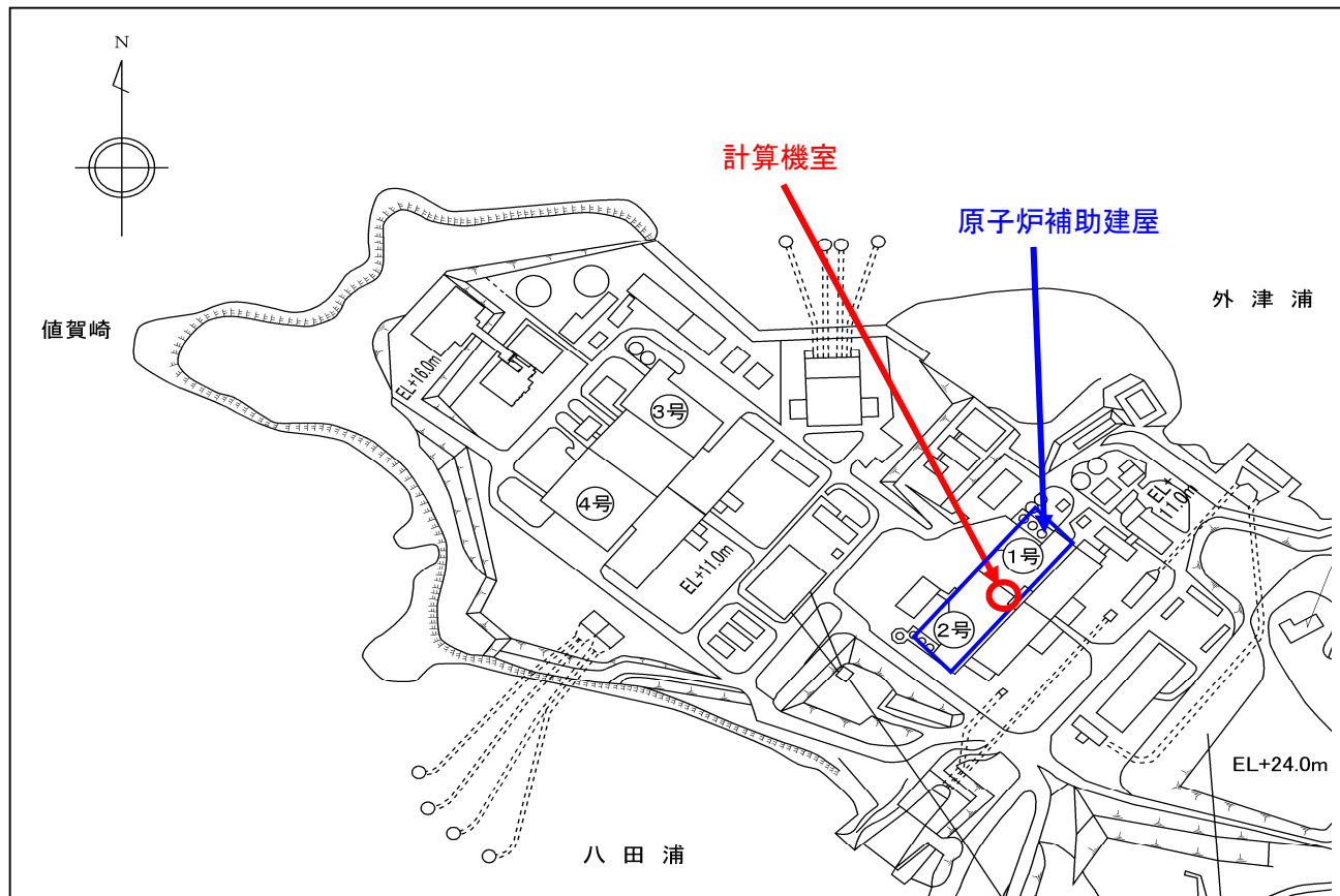
玄海原子力発電所概要図
