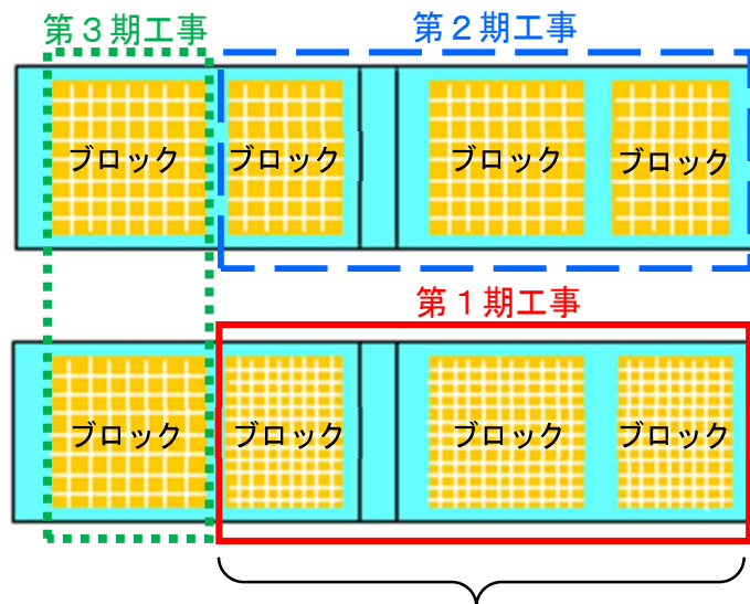
【使用済燃料プール平面図】
