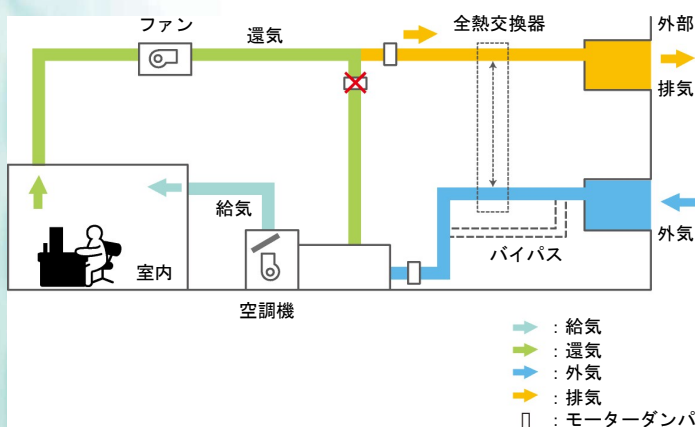
代表的なダクト系統図
