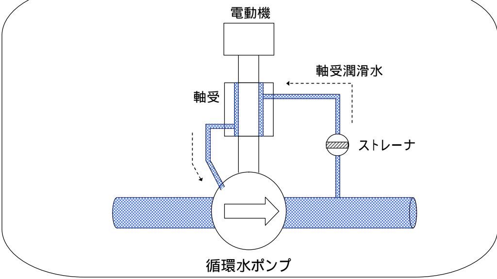
循環水ポンプ概略図
