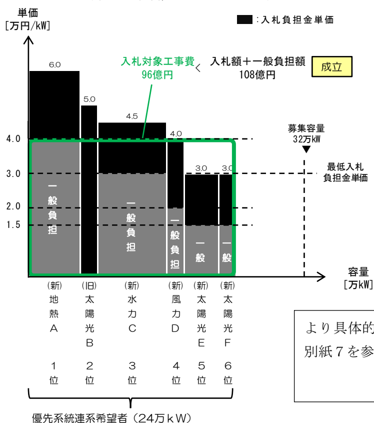
〔系統連系順位の決定イメージ〕
