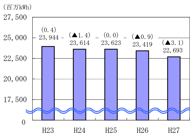
過去5か年の大口電力の推移
