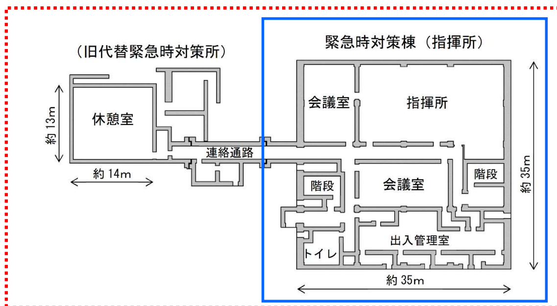
[ 平 面 (地上1階)]
