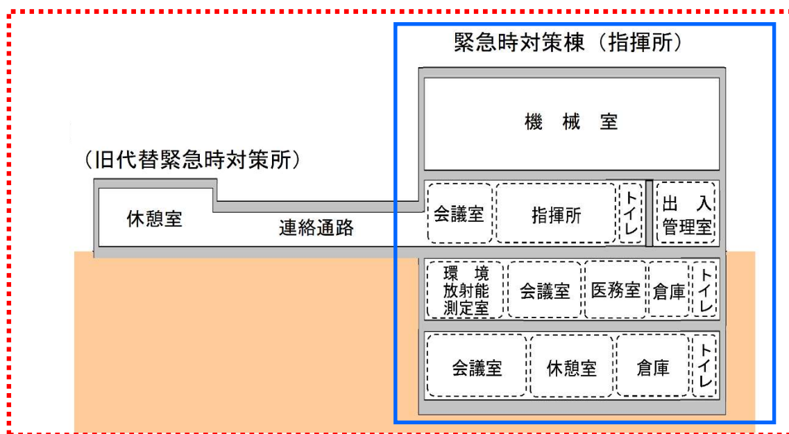
[ 断 面 ]
