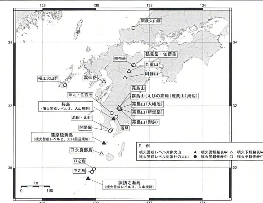
気象庁：月間火山概況（2023年3月）
