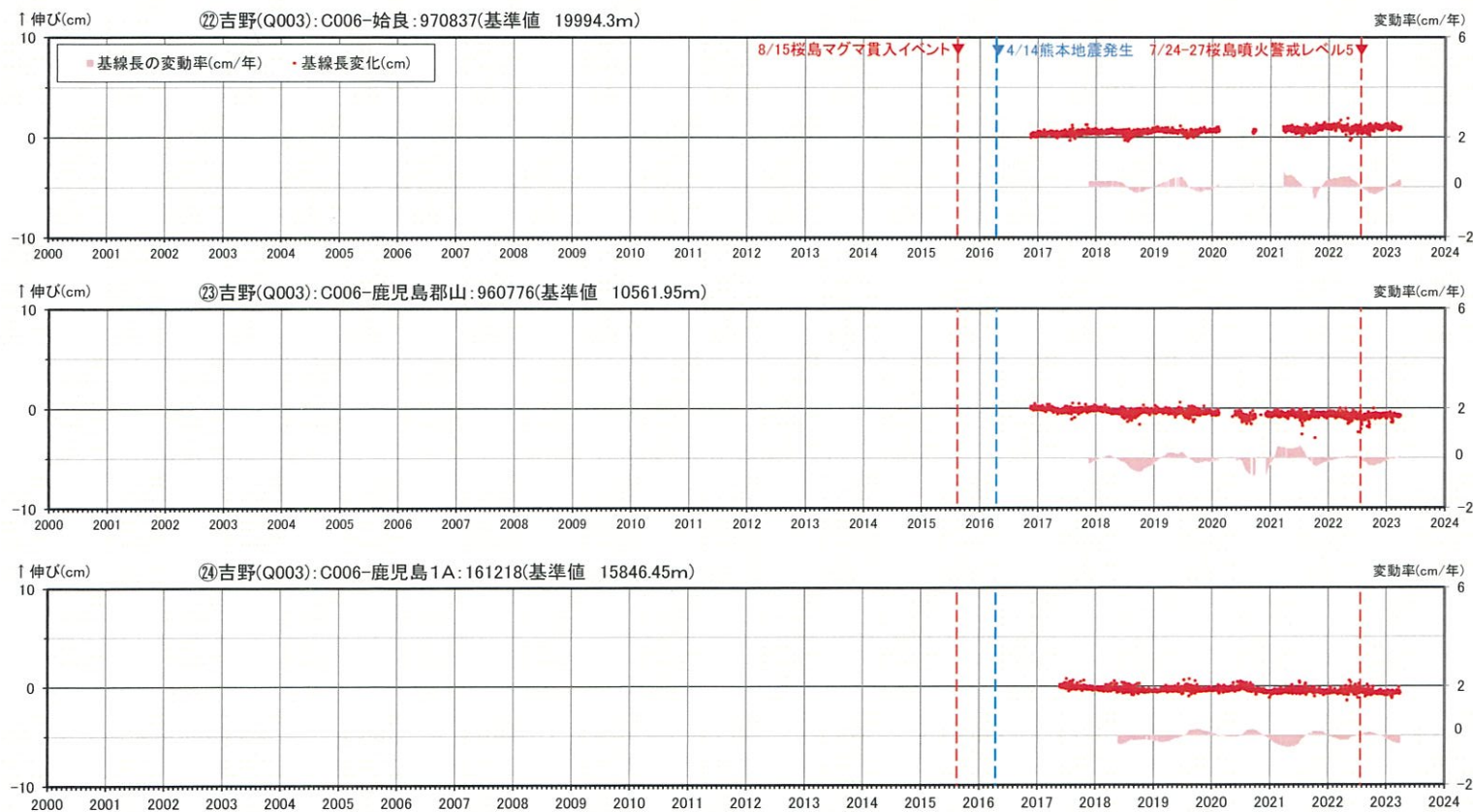
基線②②～②④の時系列変化
