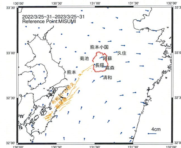
至近1年間の地殻変動
