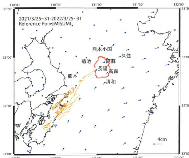
2021年度の1年間の地殻変動
