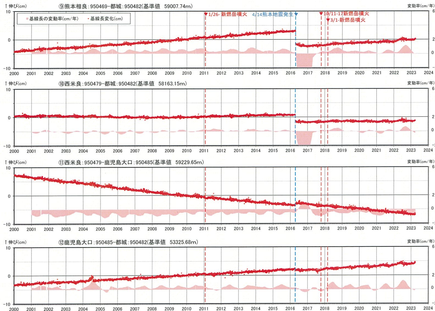
基線⑨～⑫の時系列変化
