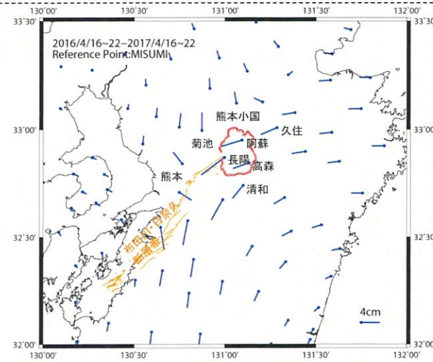
本震後1年間の地殻変動
