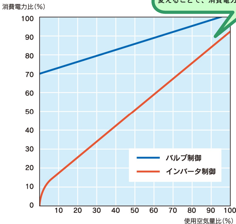
消費電力比と使用空気量比の関係
