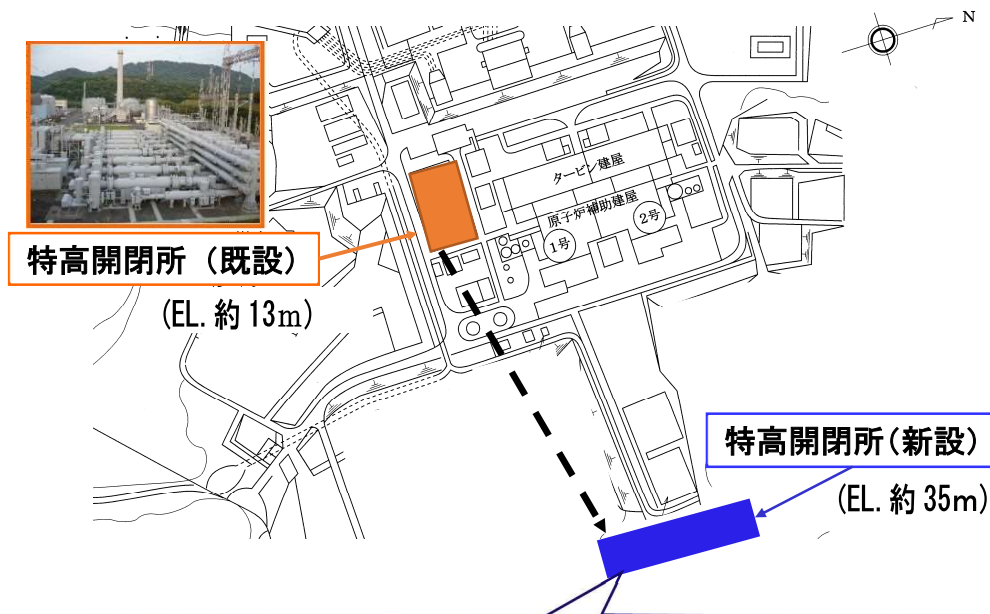
【受電回線数増強 概略図】
